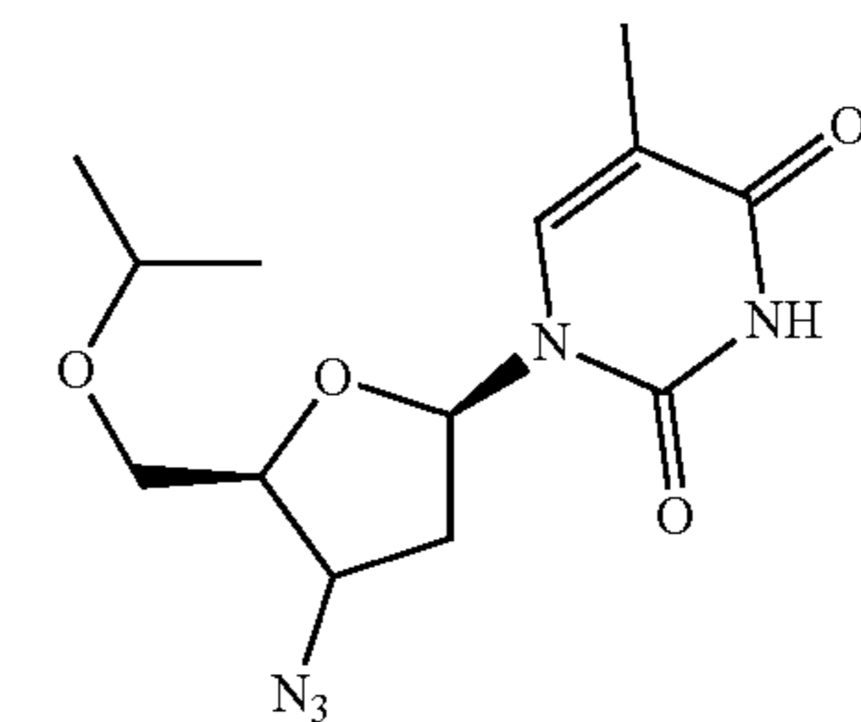
O-isopropyl-AZT
