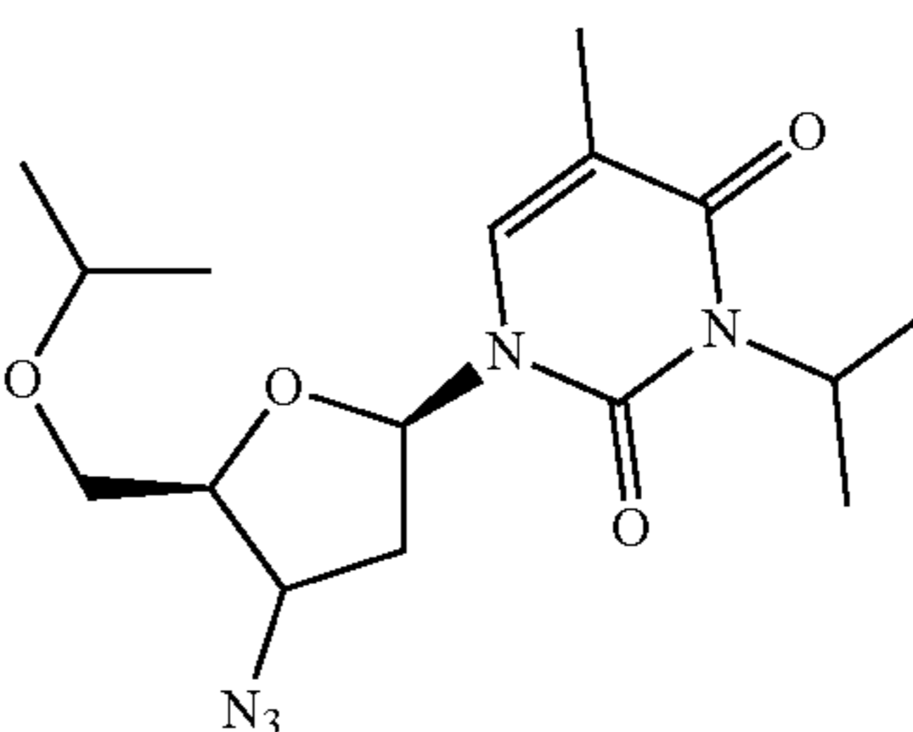
2-isopropyl-AZT
