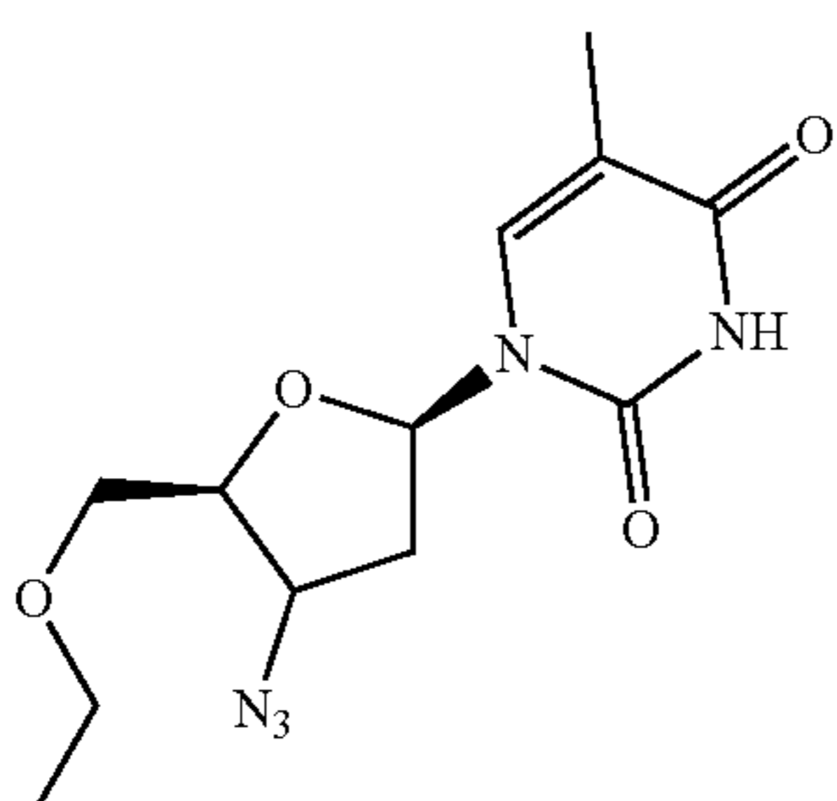
O-Et-AZT
