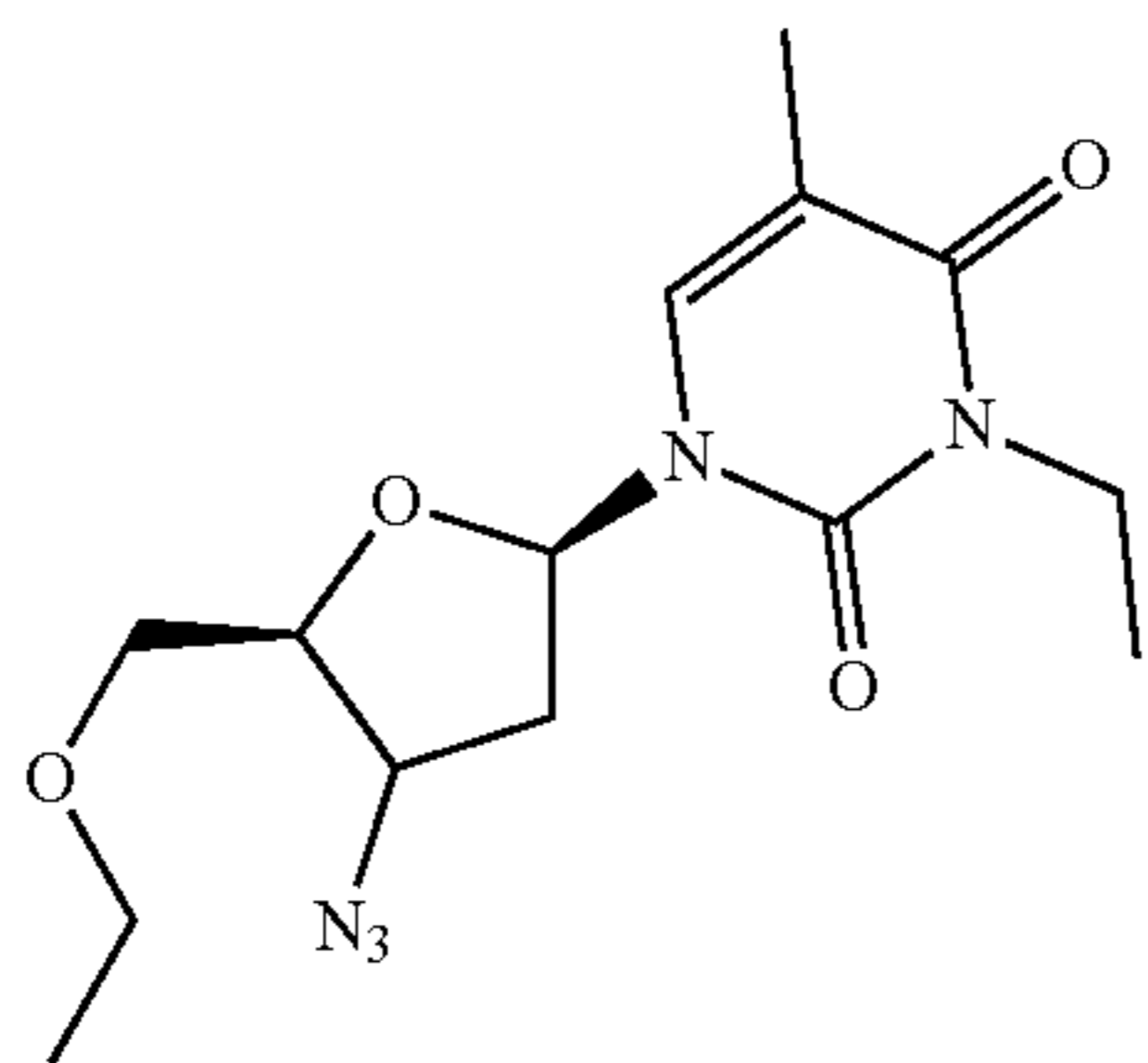
2-Et-AZT
