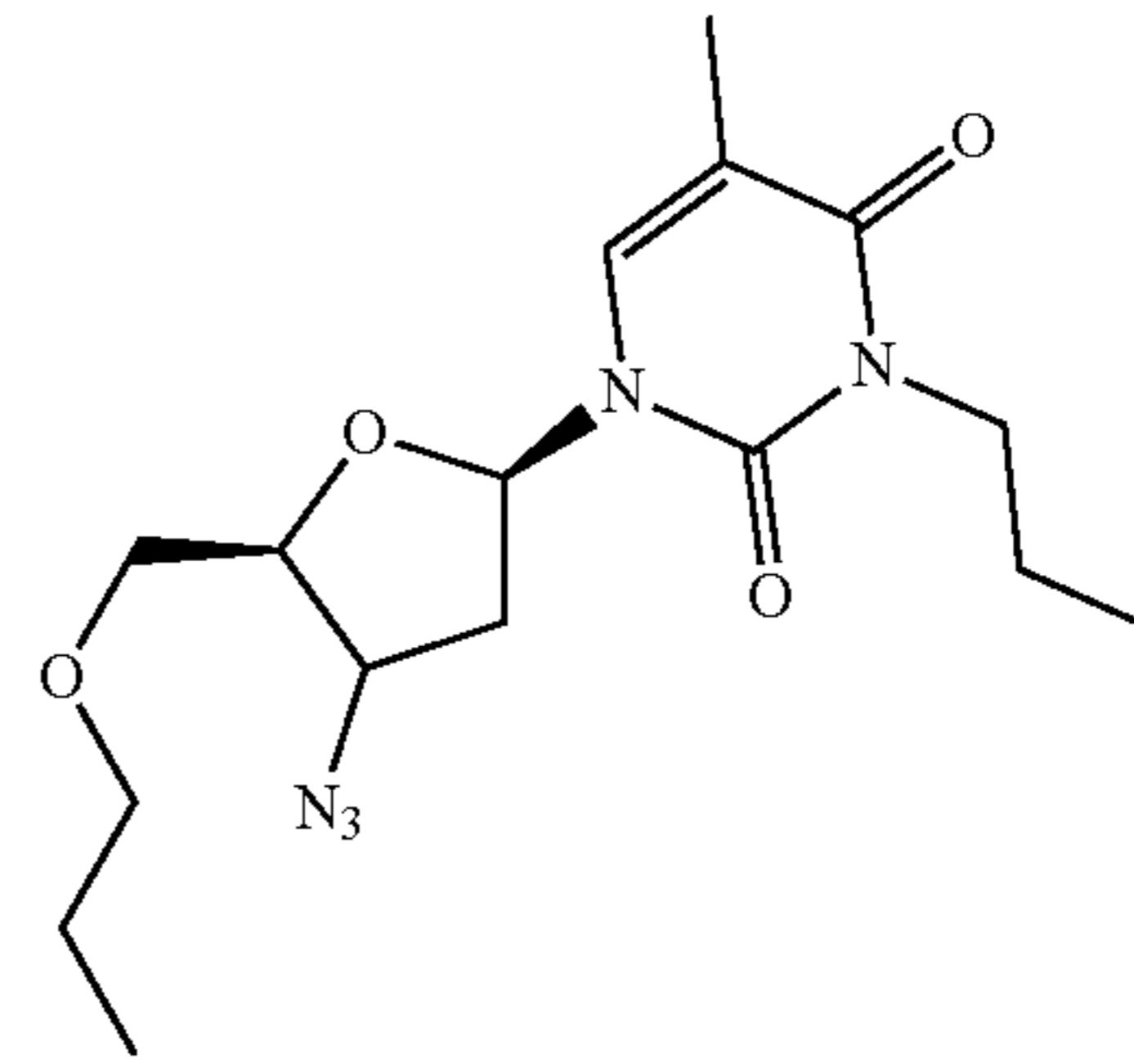
2-Propyl-AZT
