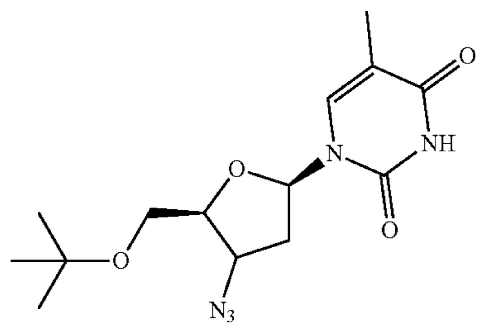
O-tert-butyl-AZT
