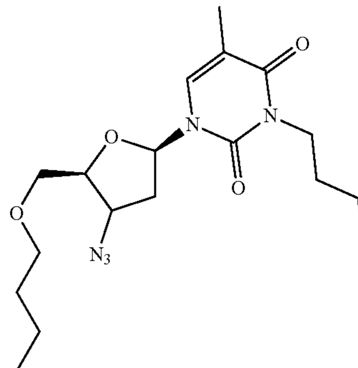
2-Butyl-AZT
