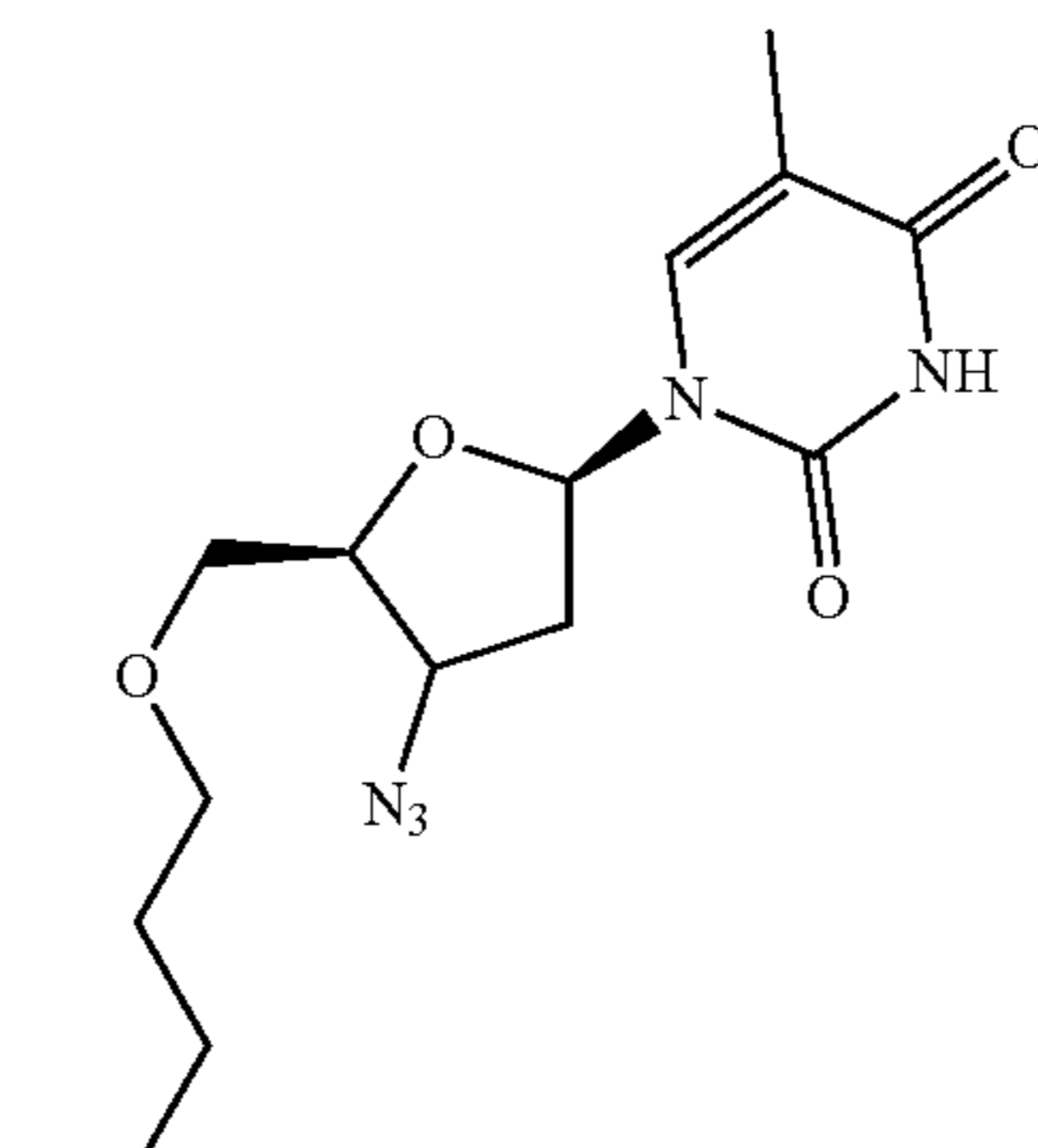
O-Butyl-AZT
