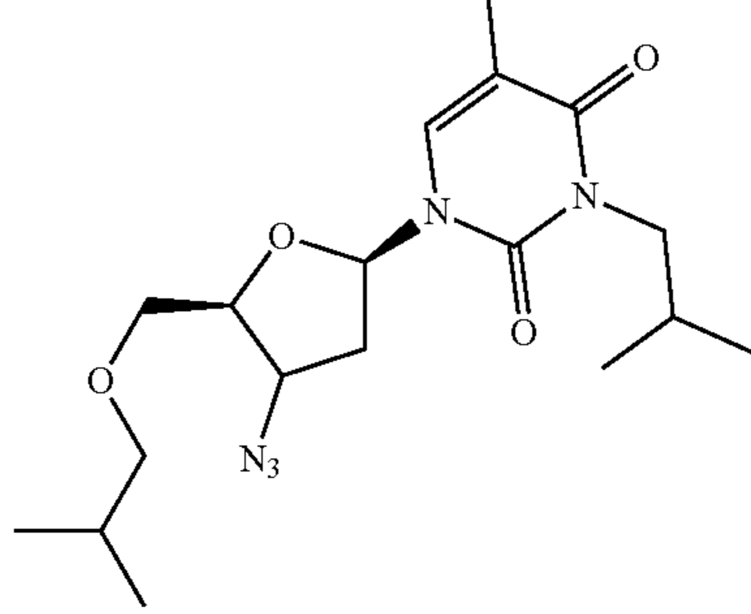
2-isobutyl-AZT
