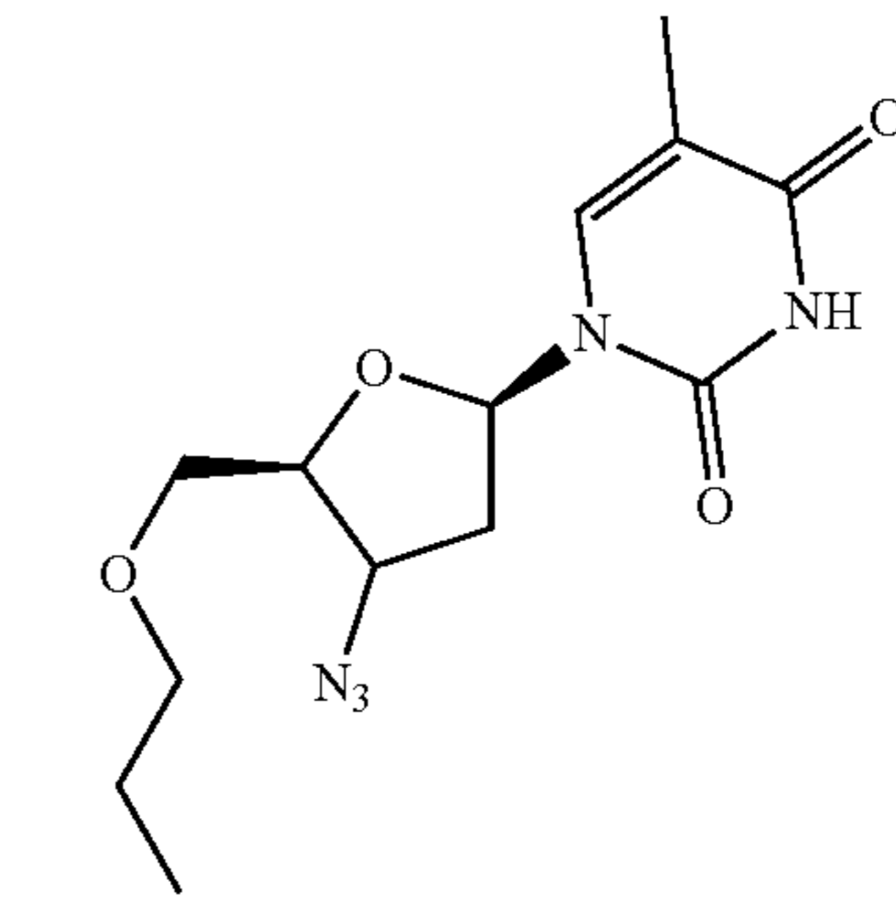
O-Propyl-AZT
