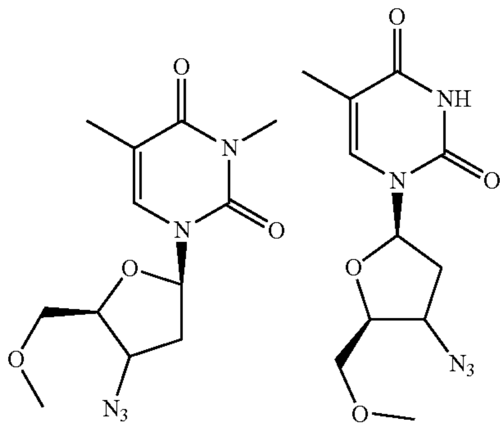
2-Me-AZT
