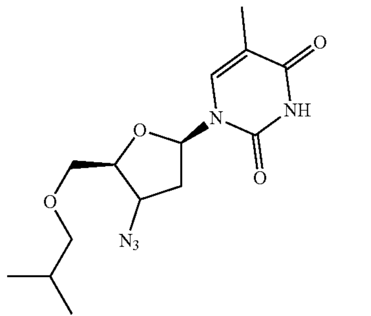
O-isobutyl-AZT
