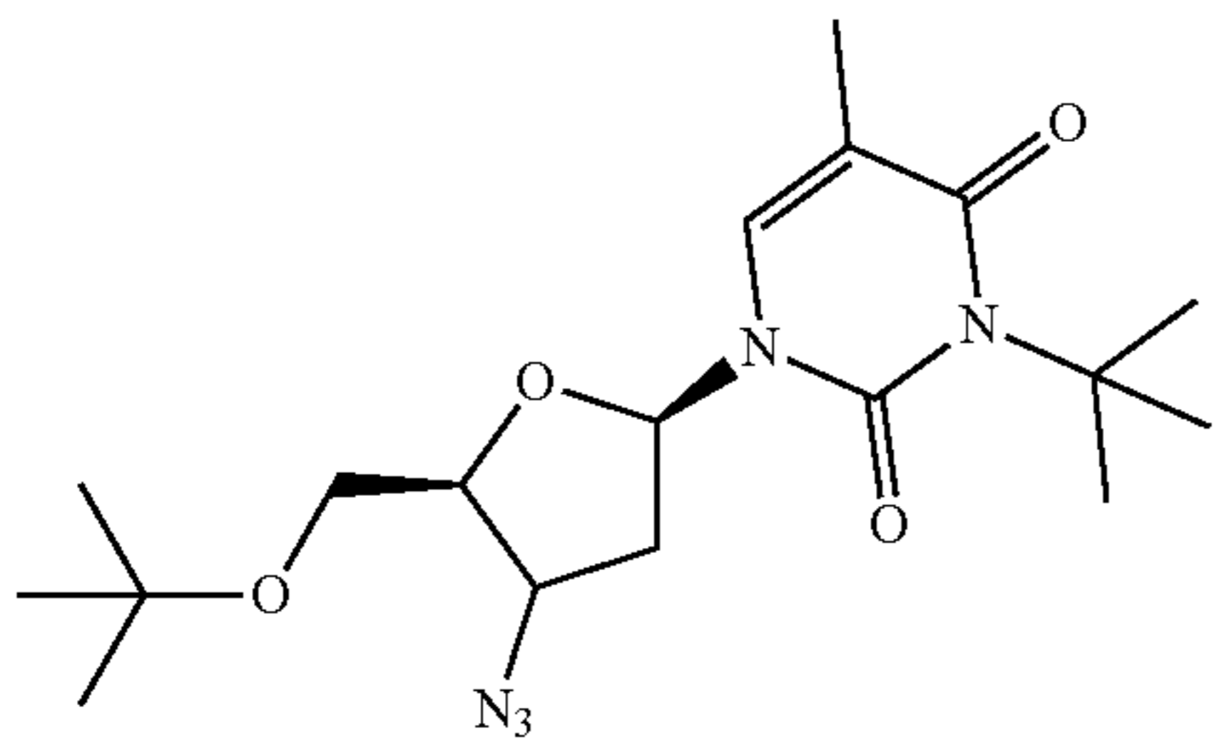
2-tert-butyl-AZT
