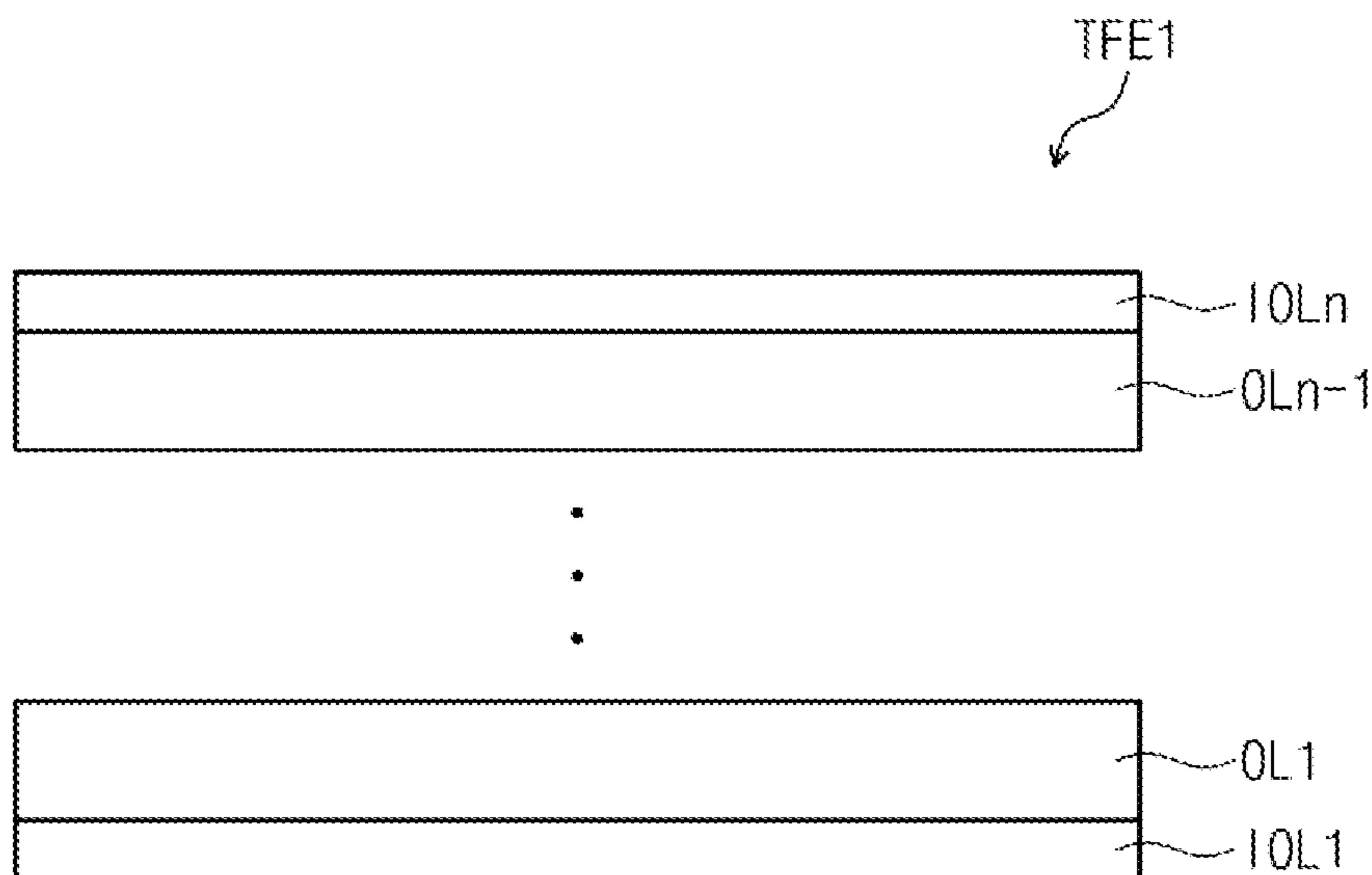
FIG. 5A
