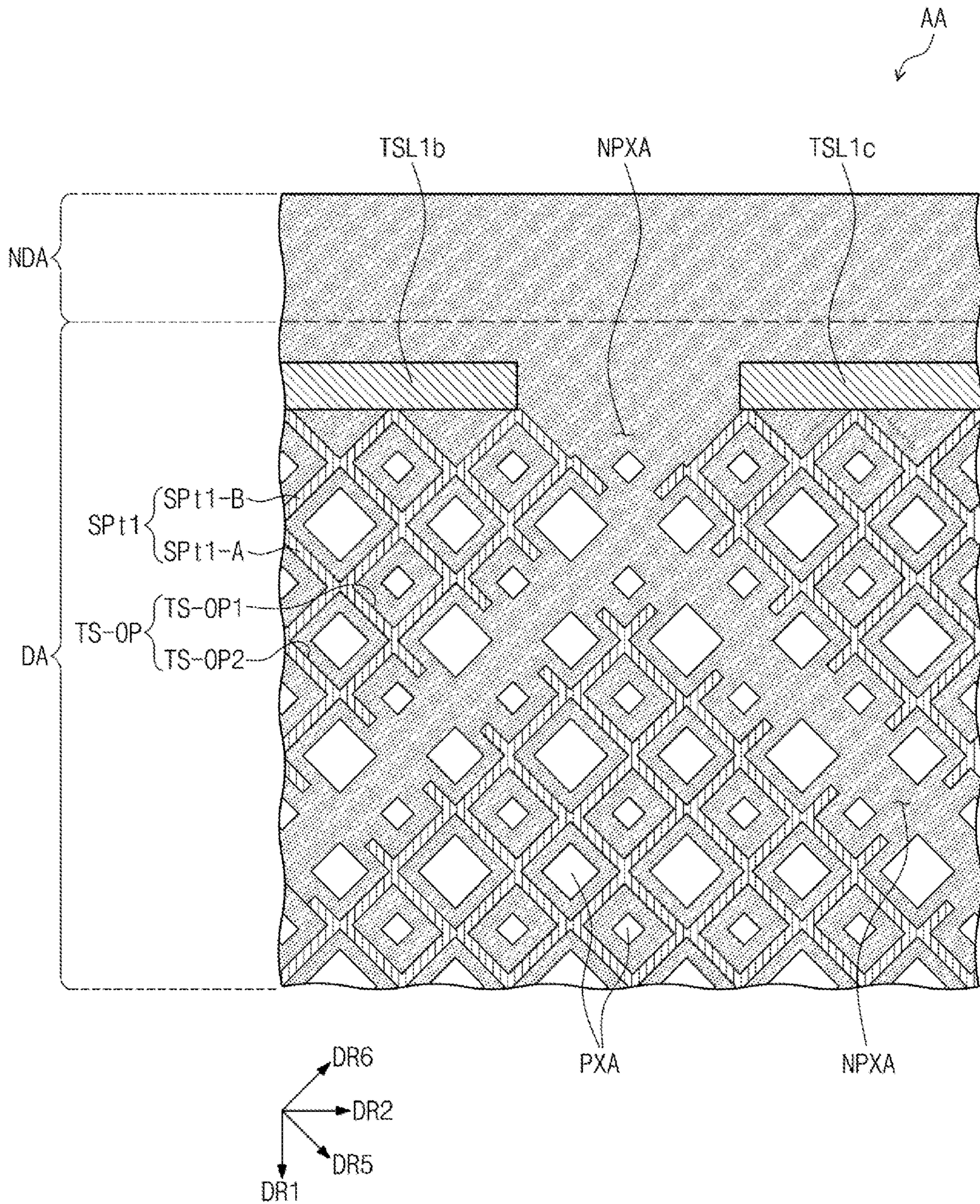
FIG. 7A
