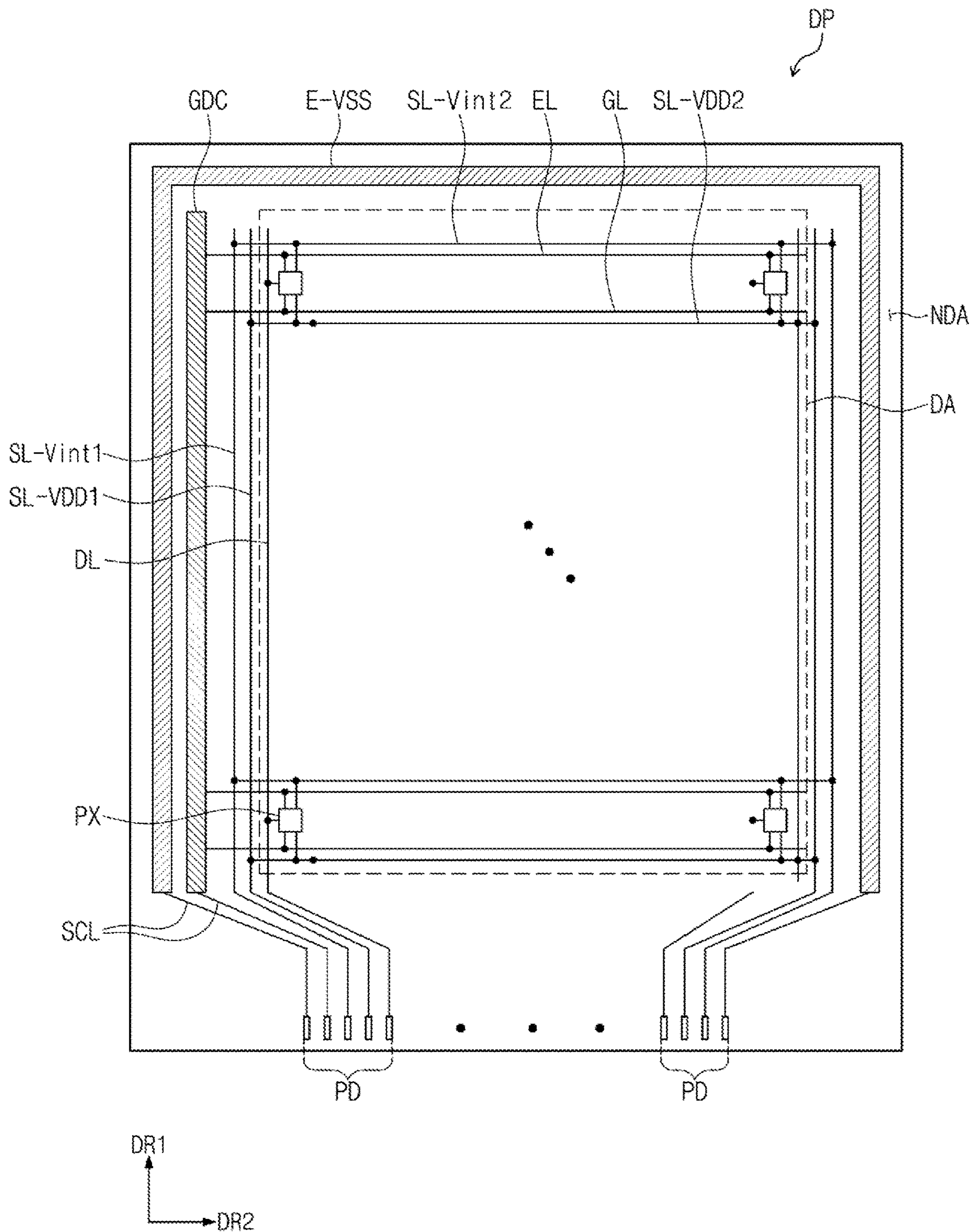
FIG. 3A
