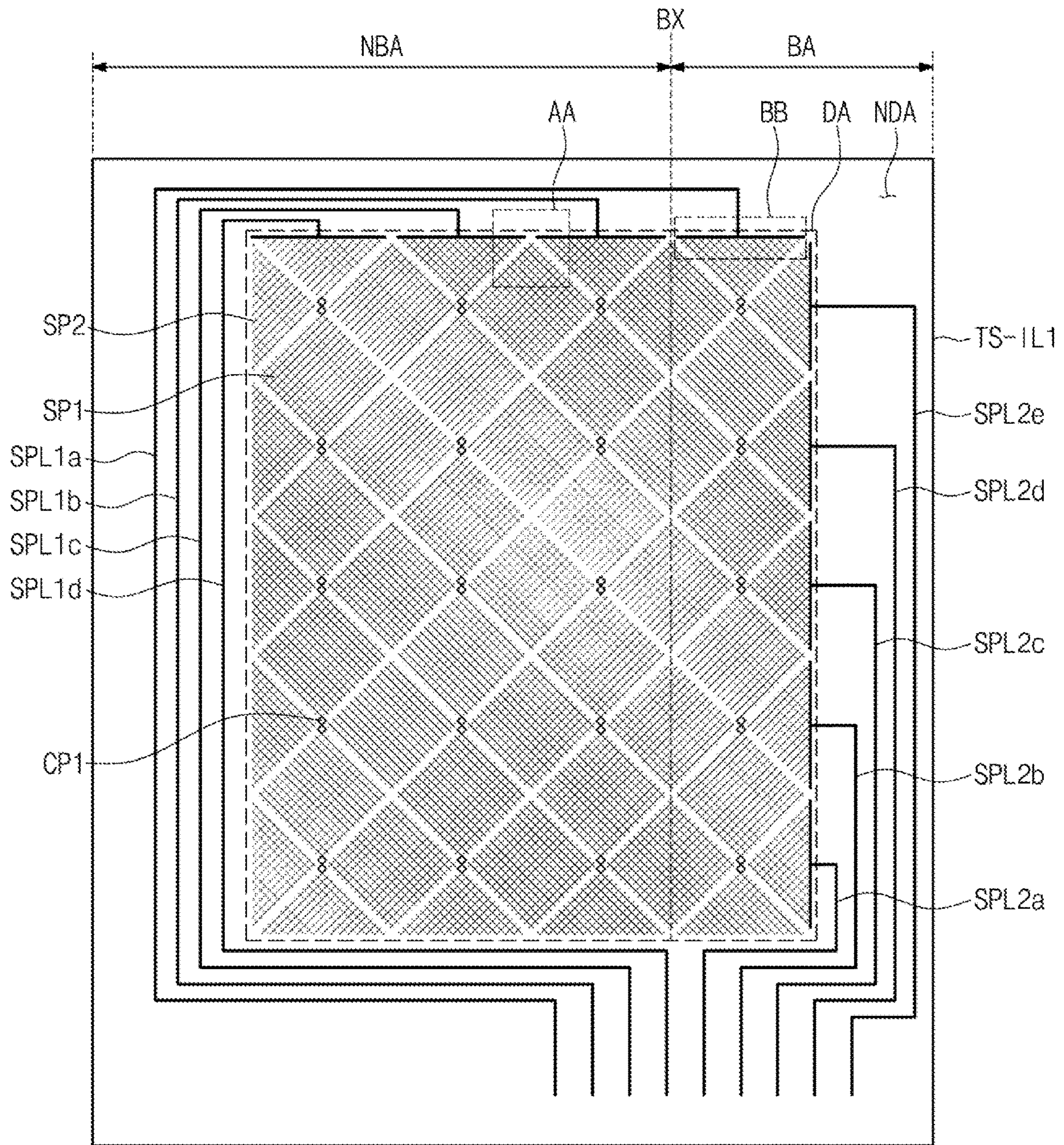
FIG. 6E
