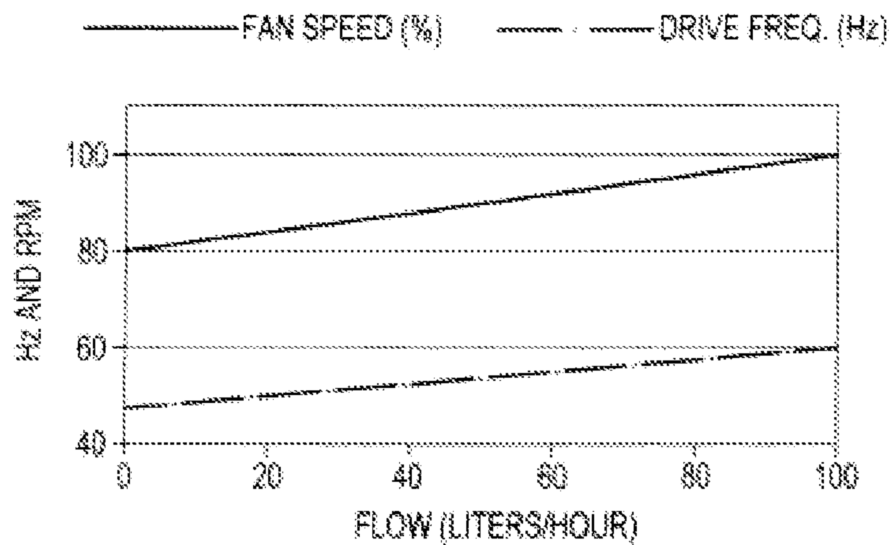
FIG. 11 FAN SPEED SCHEDULE
