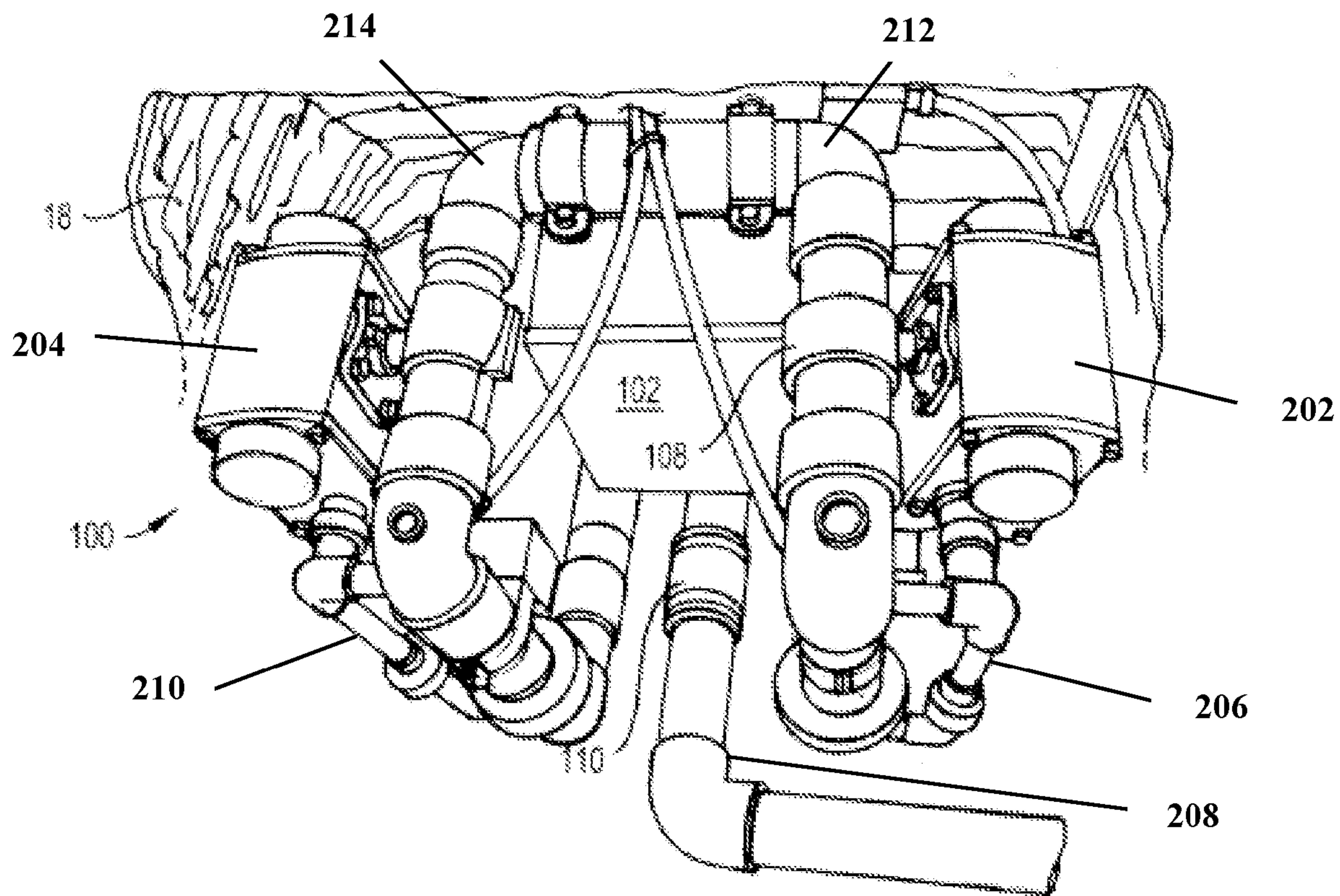
FIG. 10 CONDENSATE FLOW METER
