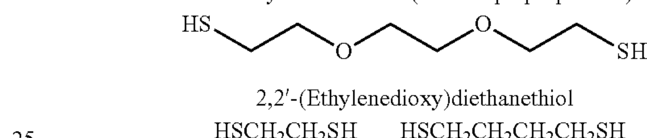
2,2'-(Ethylenedioxy)diethanethiol
