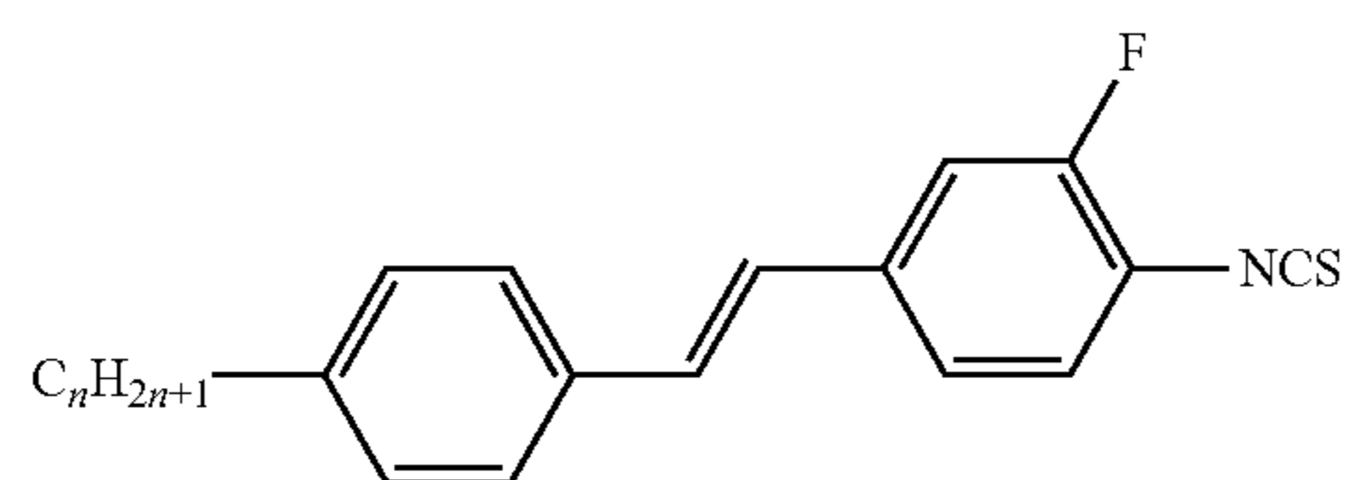
PVG-n-S
