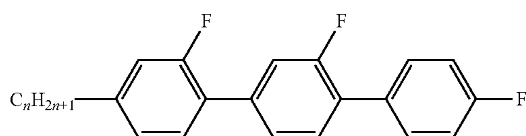
GGP-n-F
