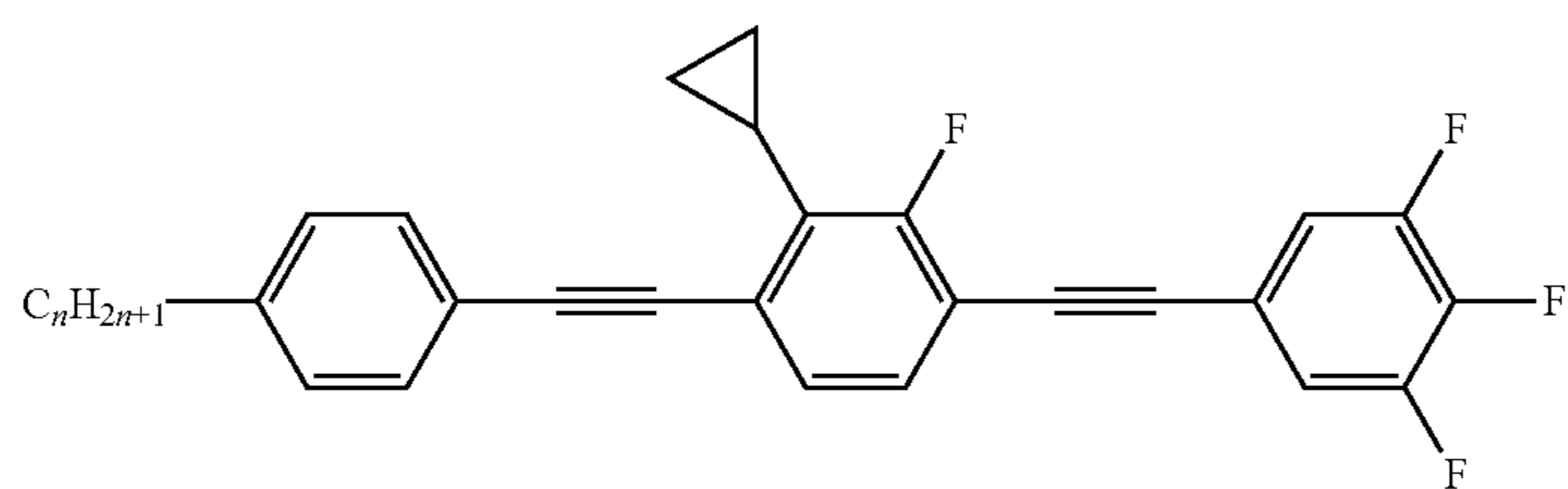
PTG(c3)TU-n-F
