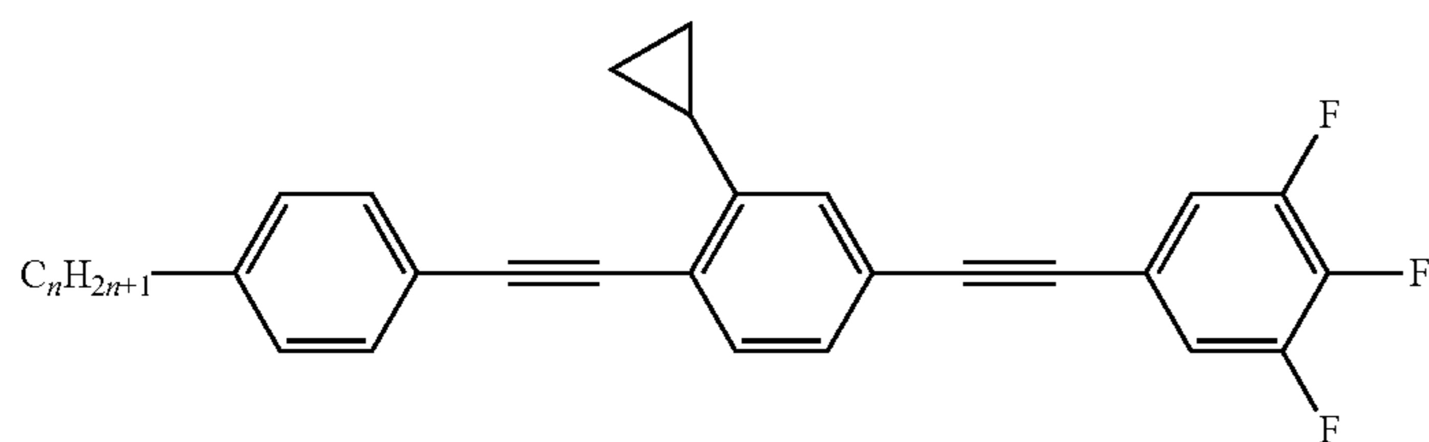
PTPI(c3)TU-n-F
