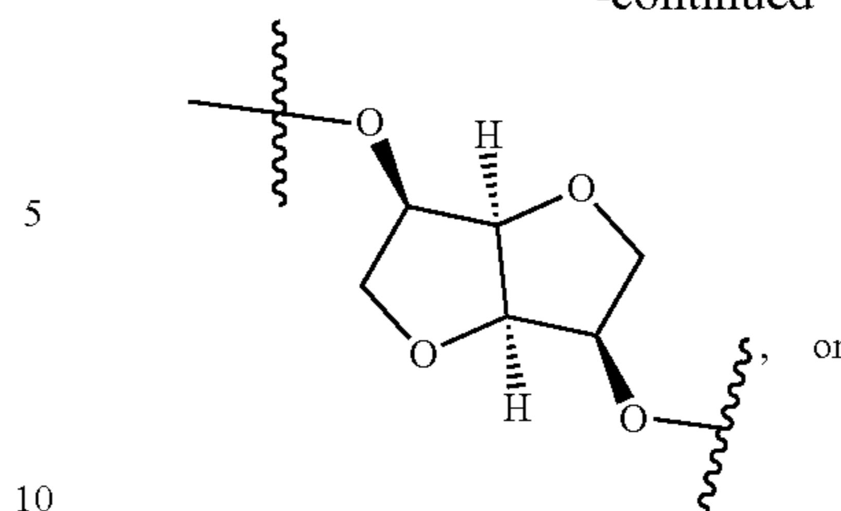
(dianhydromannitol)
