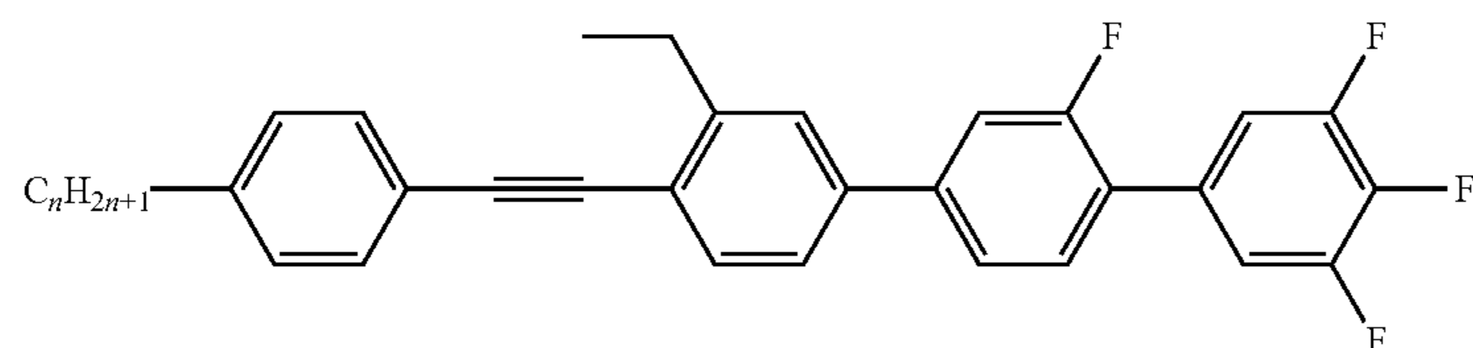
PTPI(2)GU-n-F
