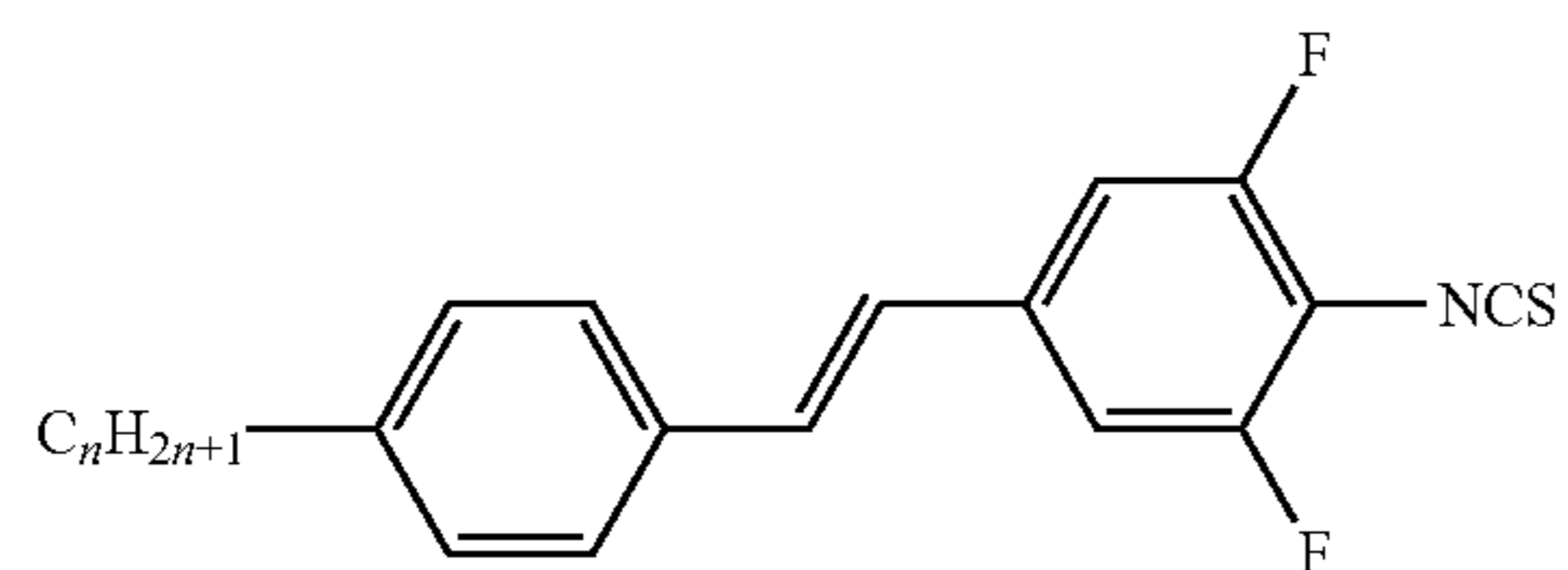
PVU-n-S
