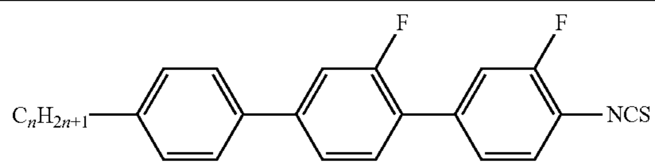
PGG-n-S
