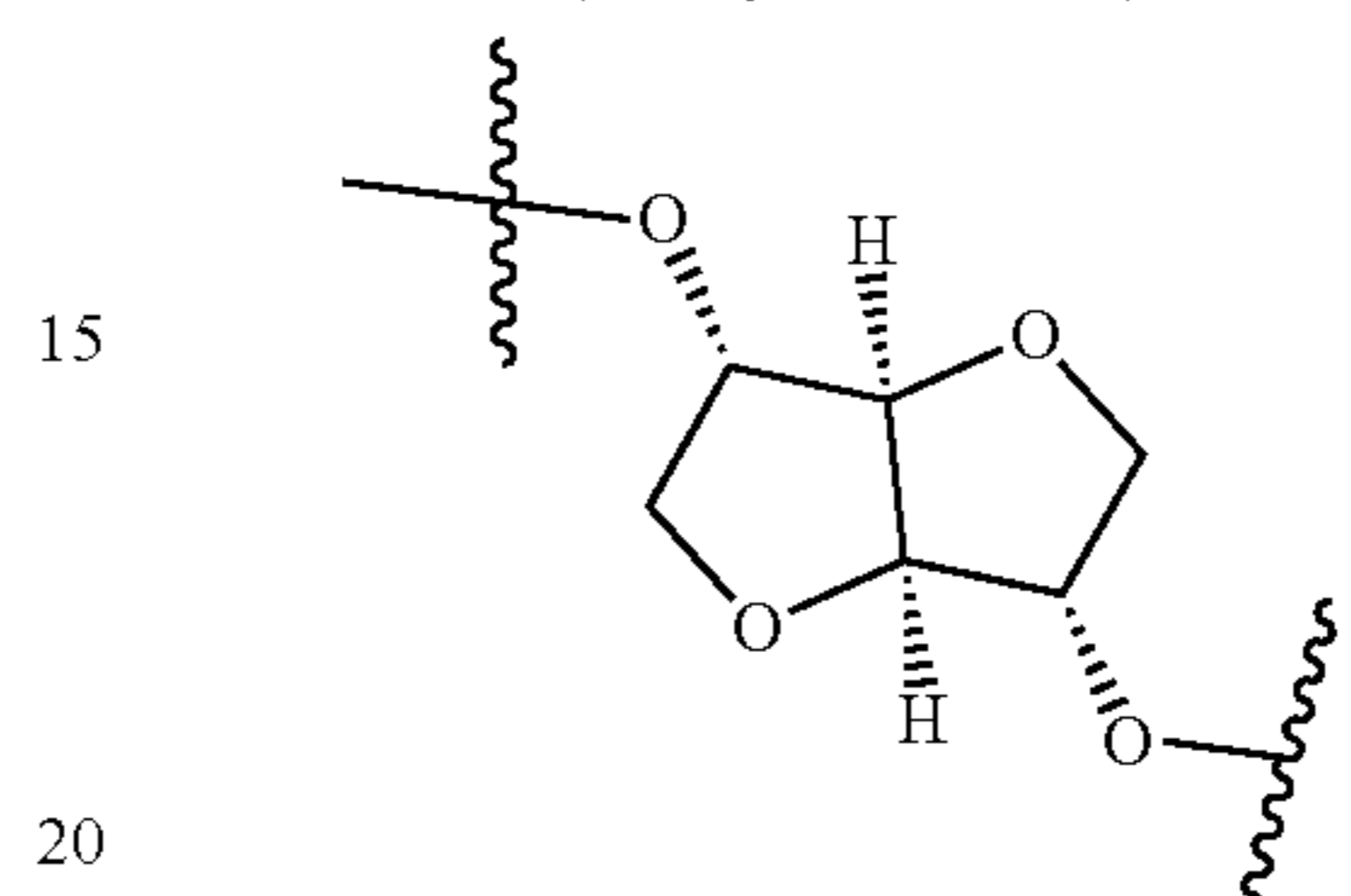
(dianhydroiditol)
