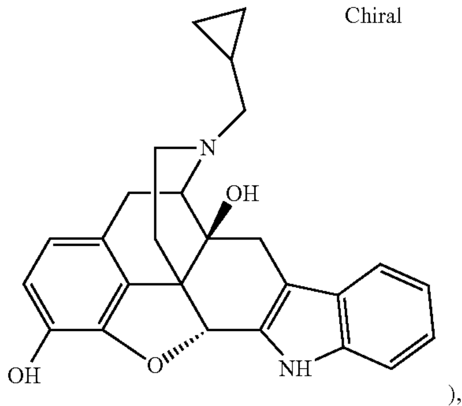
naltrindole (
