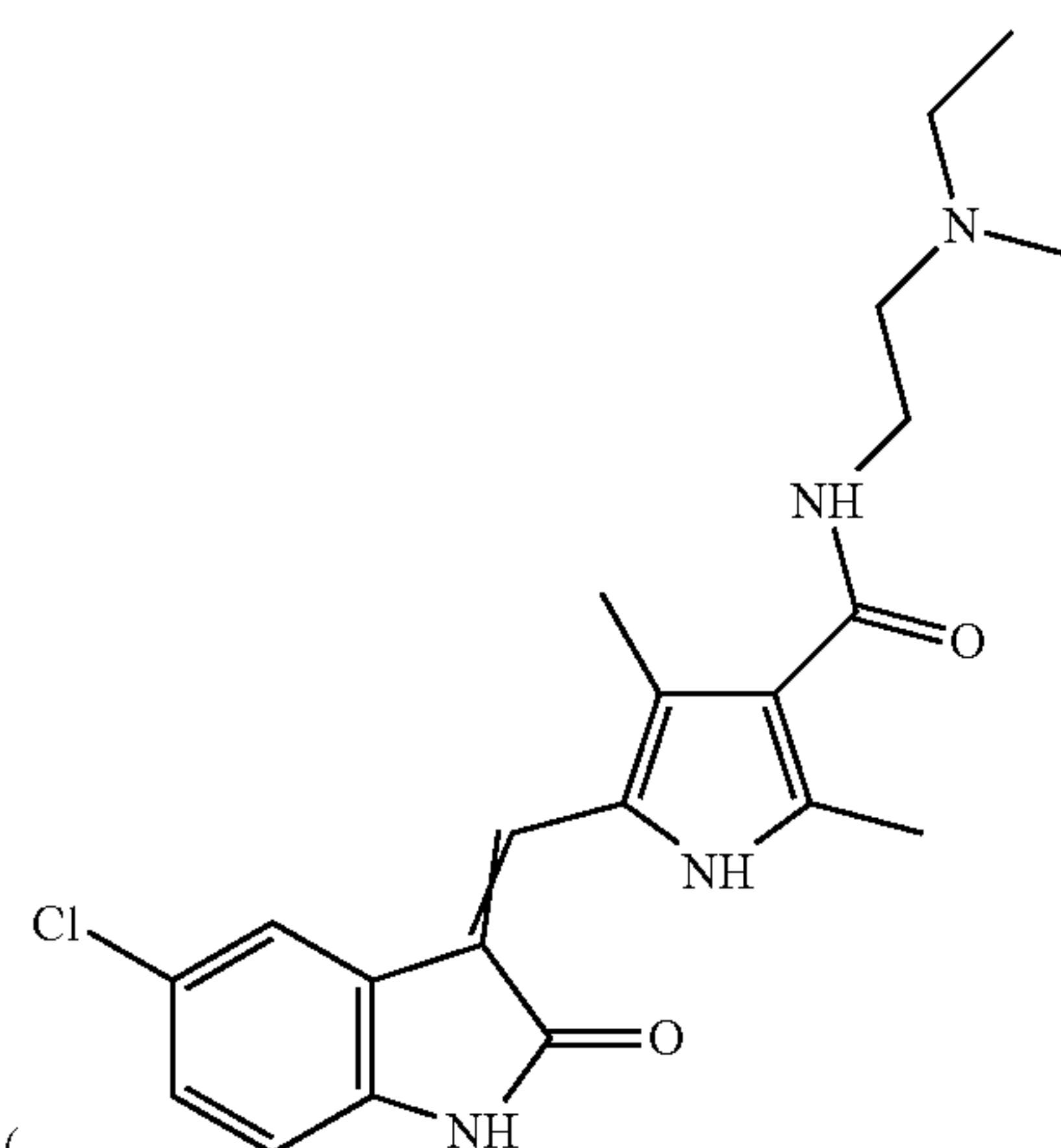
SU11652 ( ),
