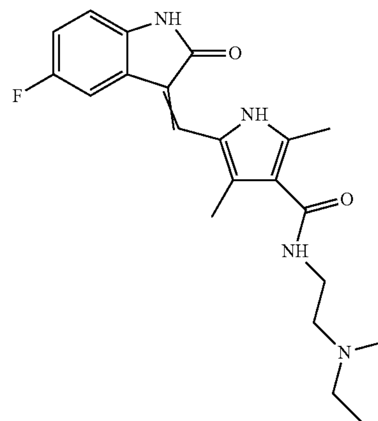
Sunitinib (SU 11248, ),
