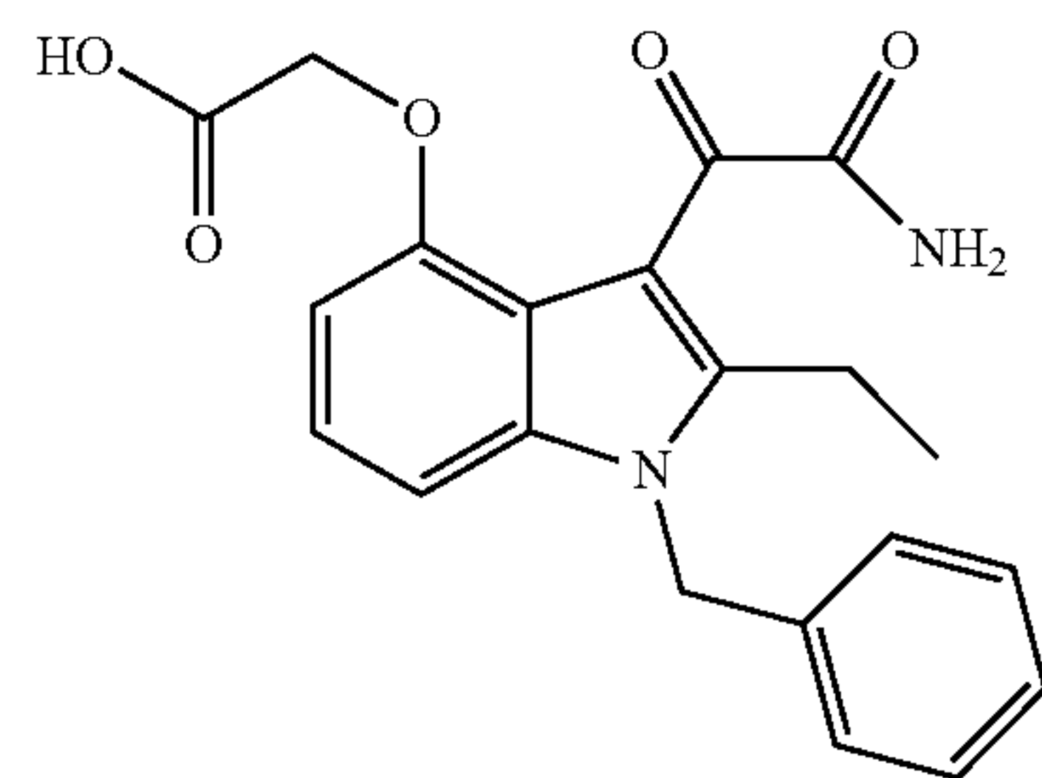
Varespladib
