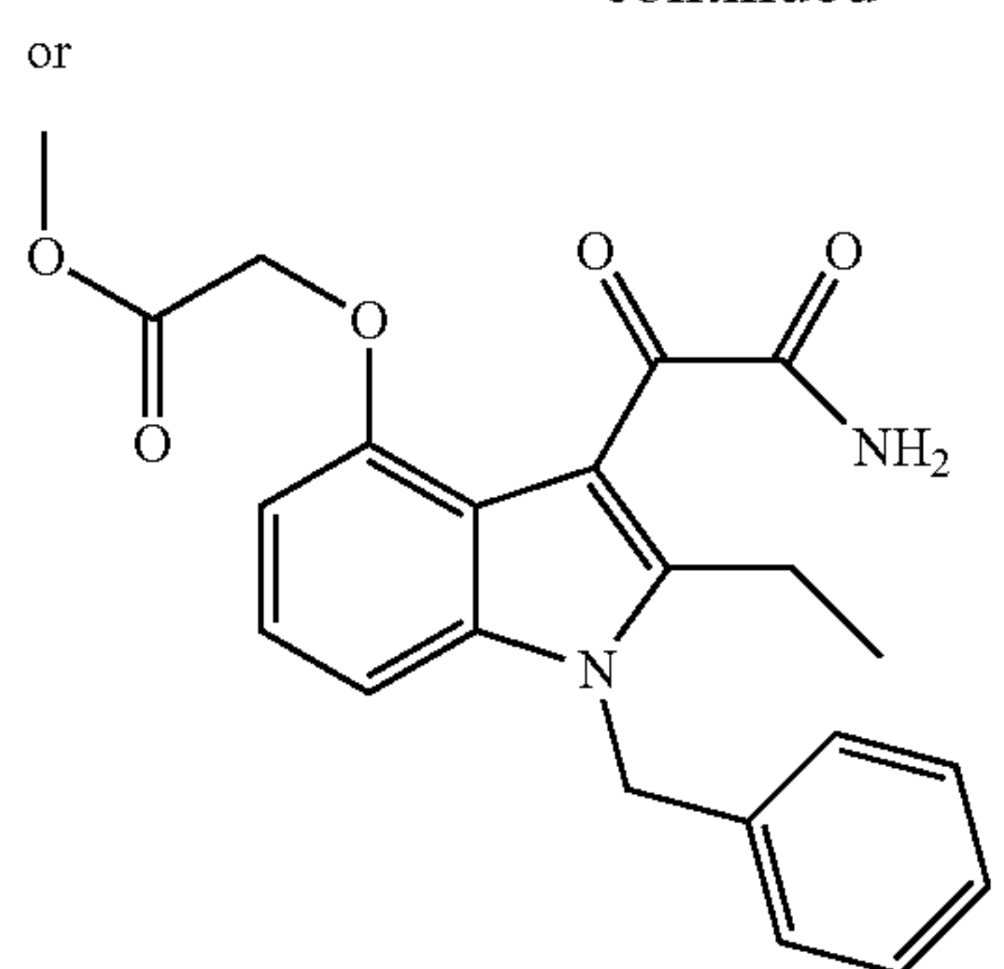
Varespladib Methyl
