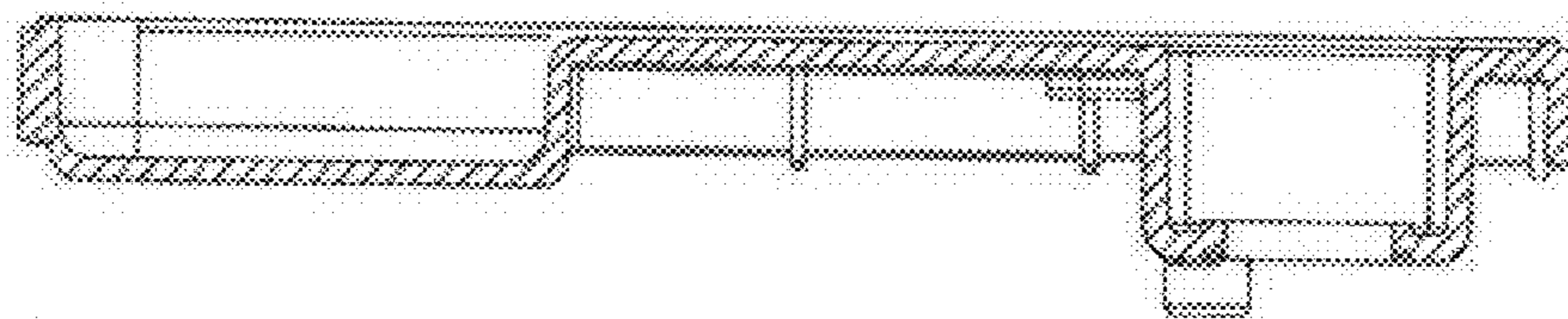
SECTION D-D
