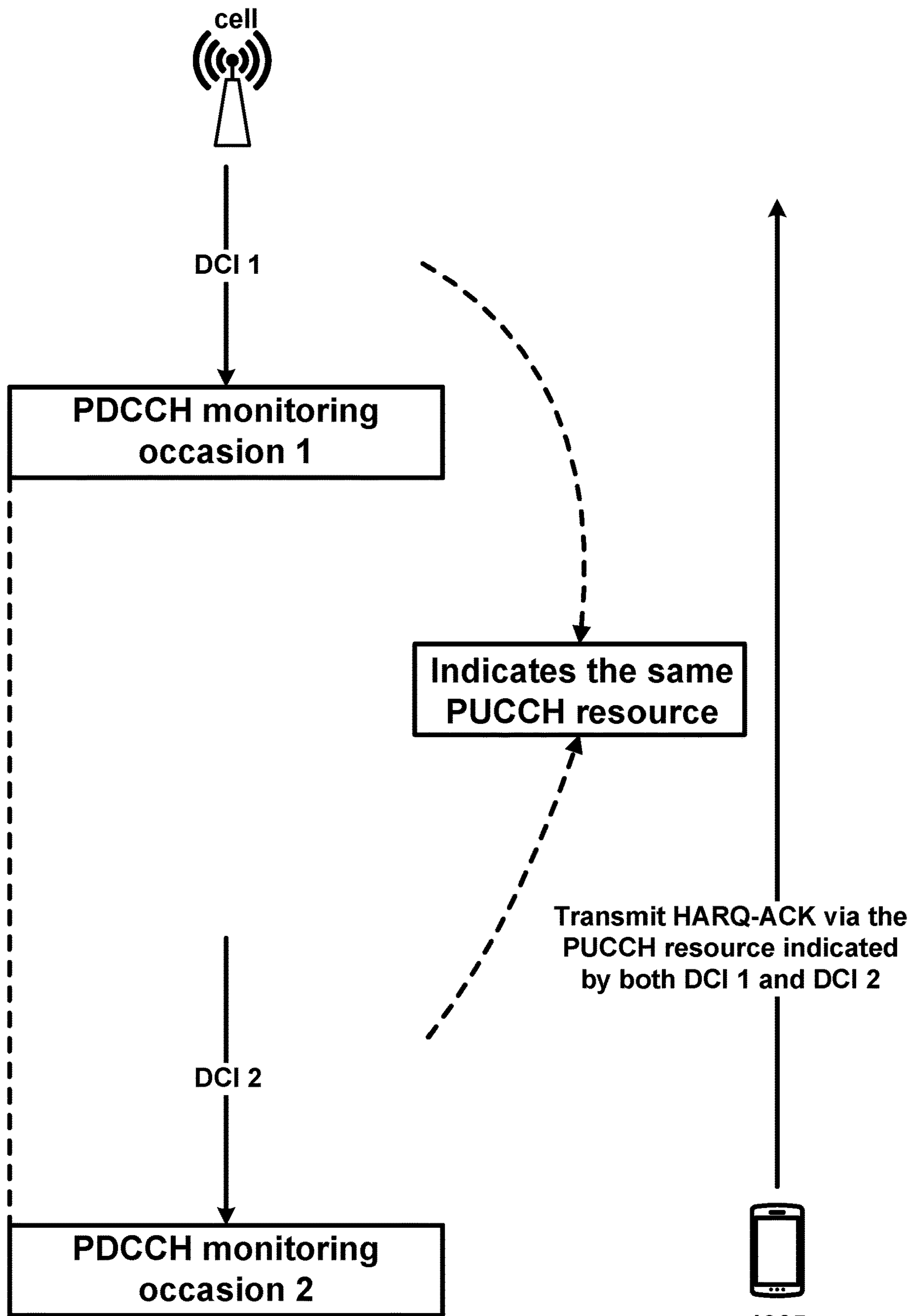
FIG. 25
