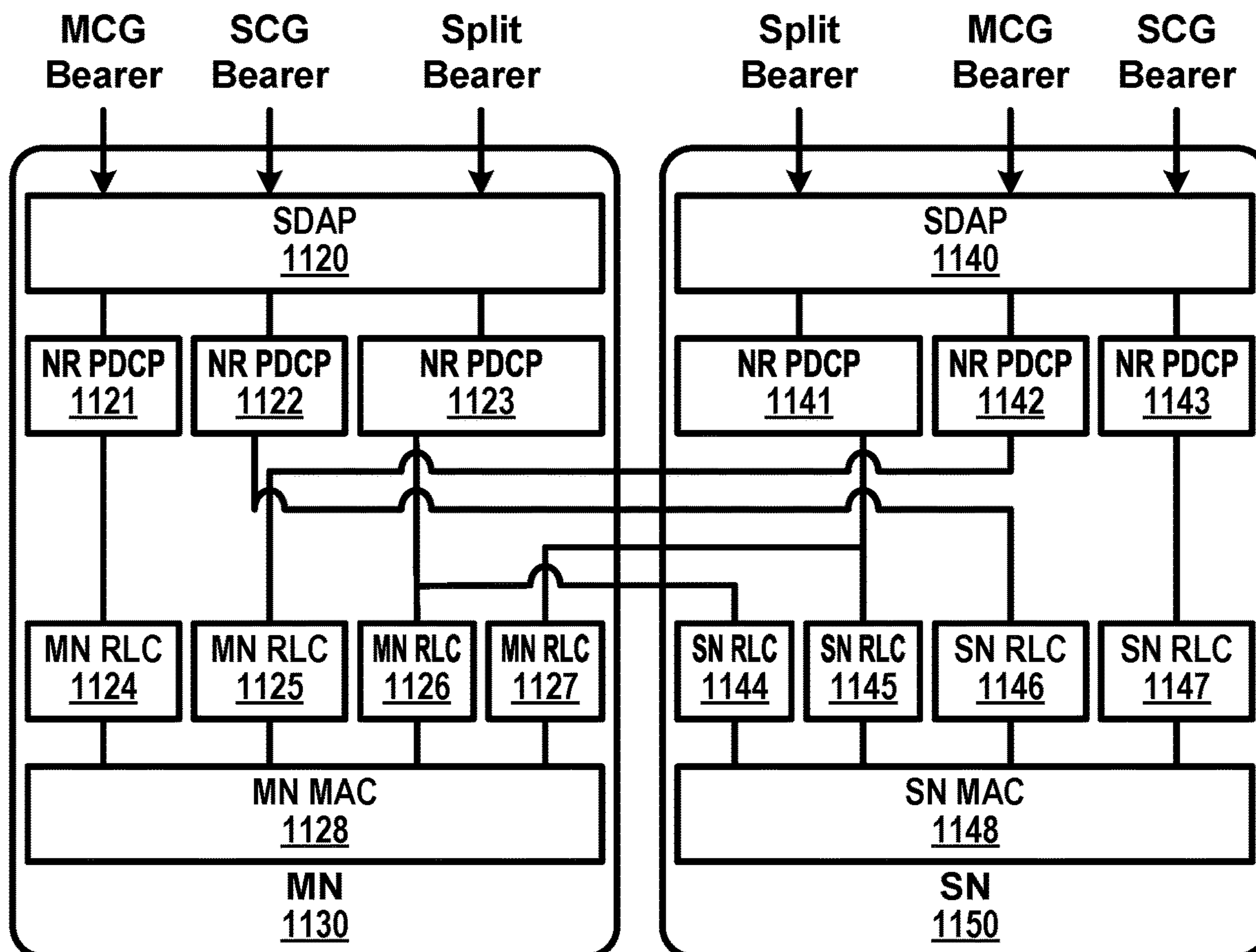
FIG. 11B
