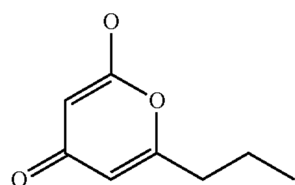
Mol. Wt.: 154.16
