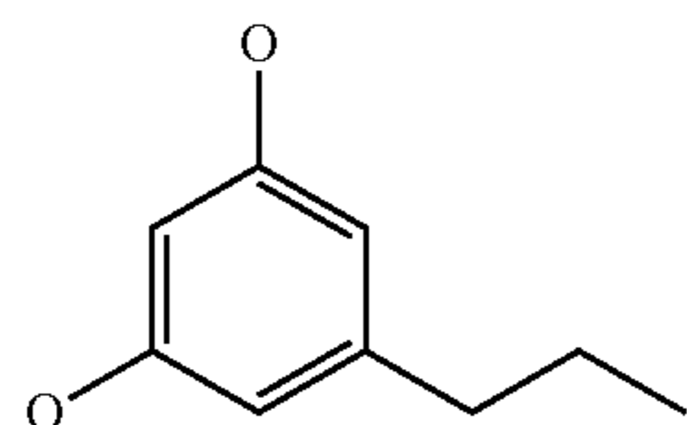
Mol. Wt.: 152.19
