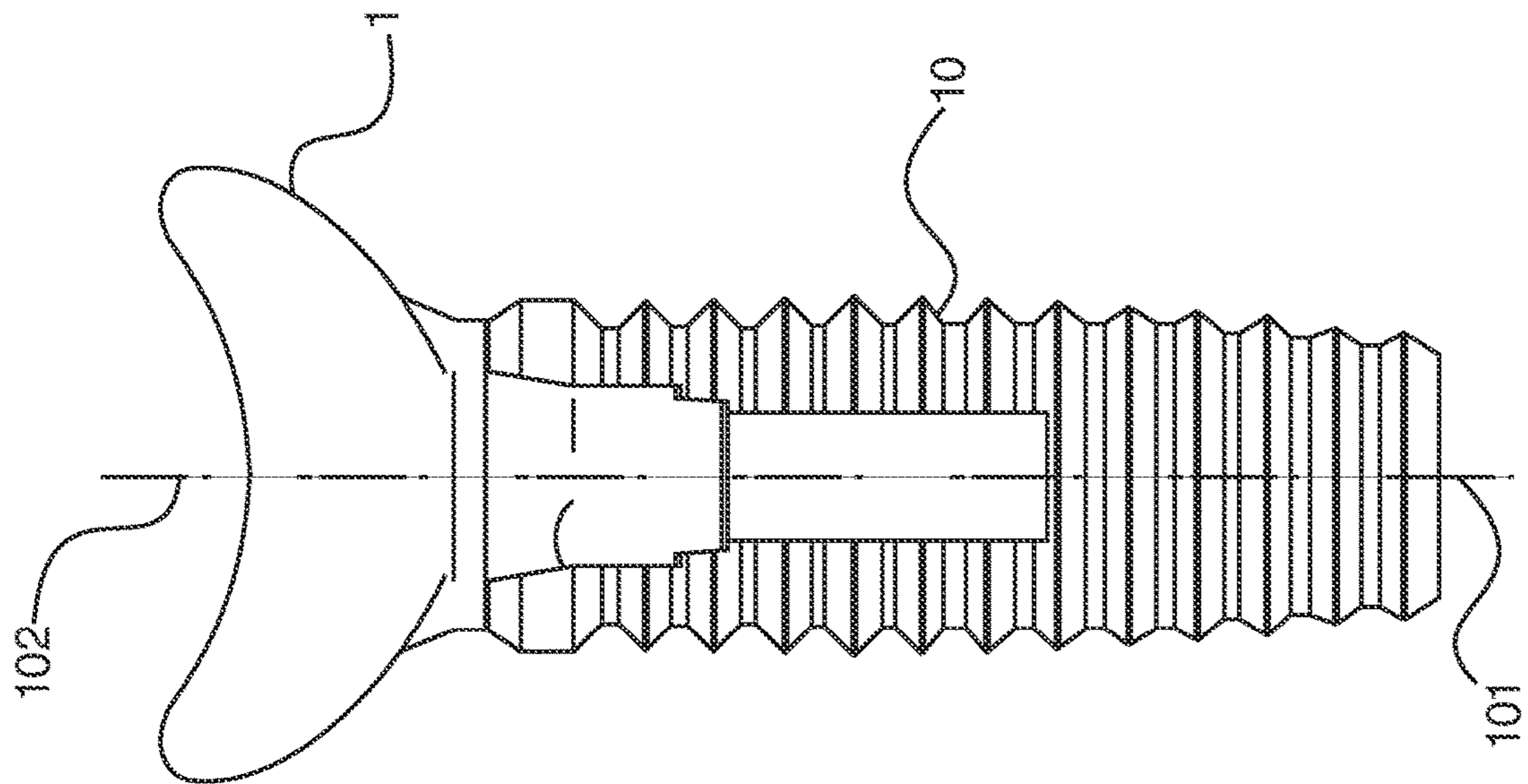
FIG. 19
