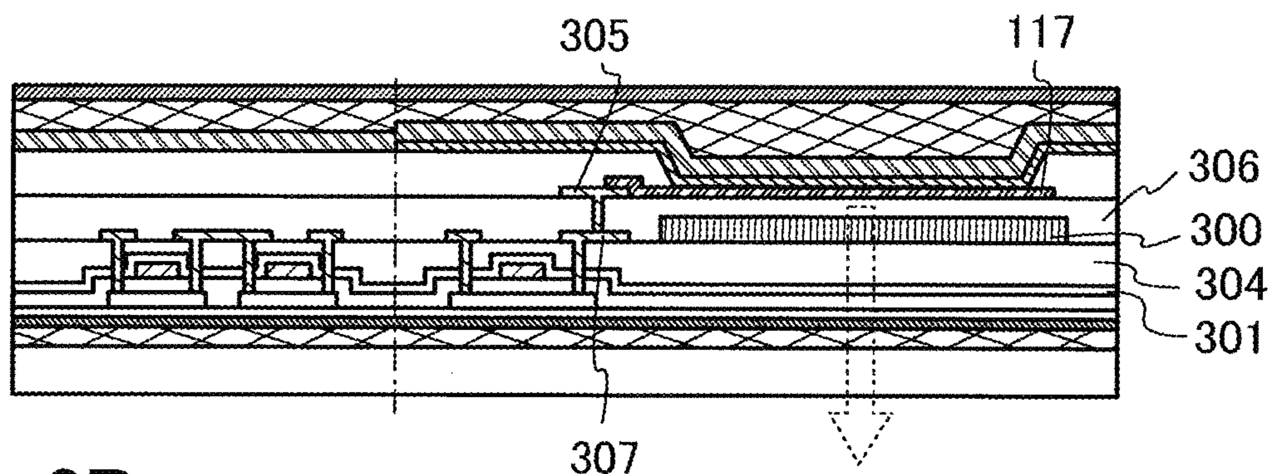
FIG. 2B
