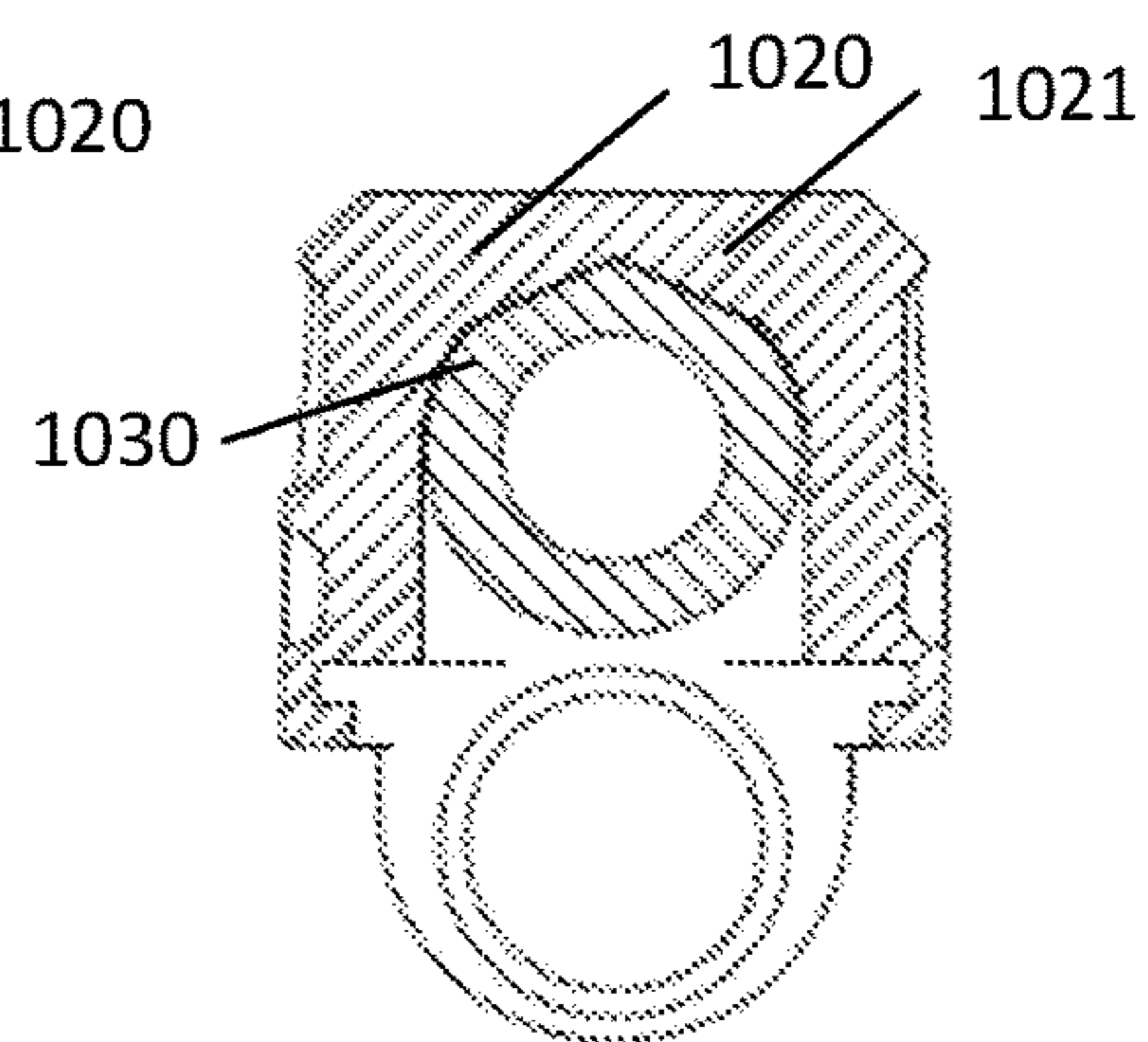
SECTION AU-AU
