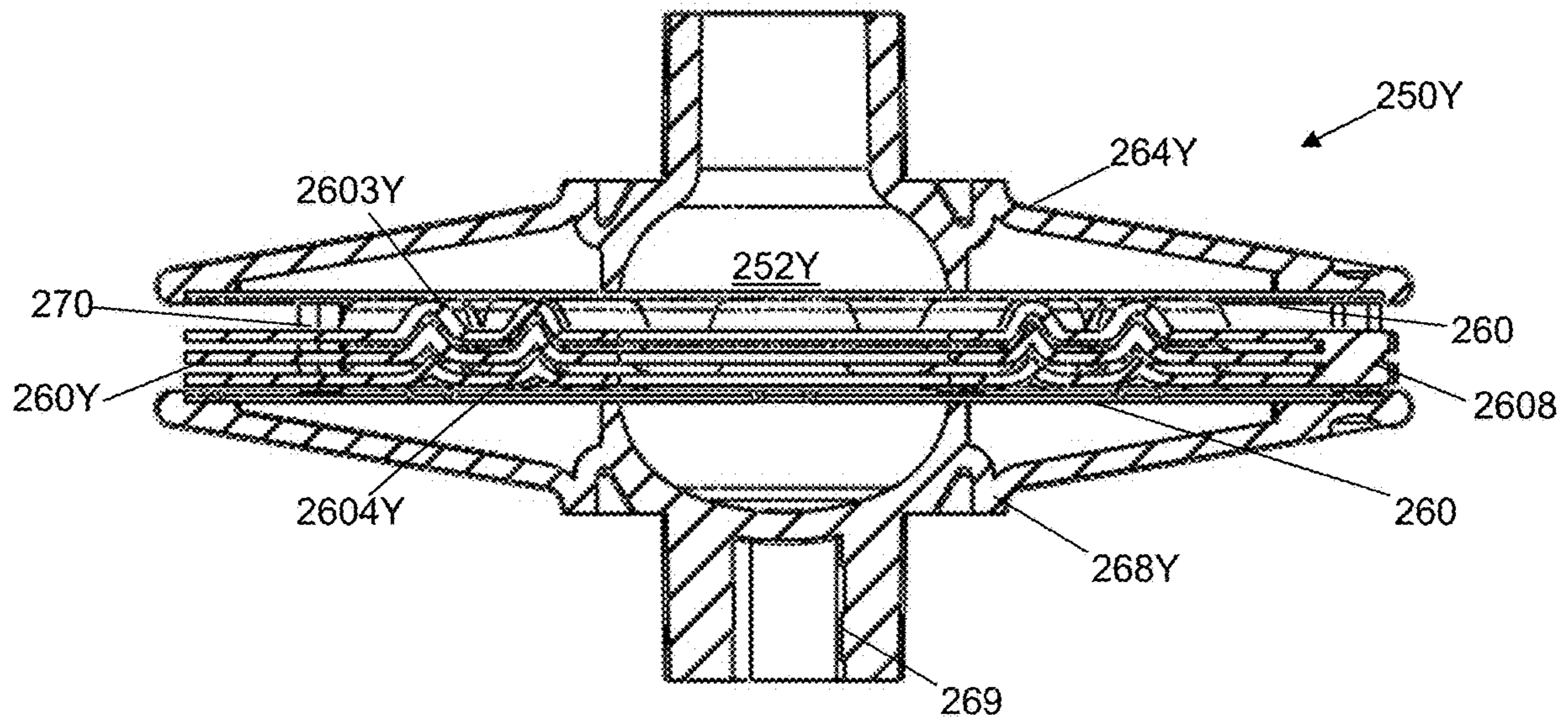
FIG. 19E
