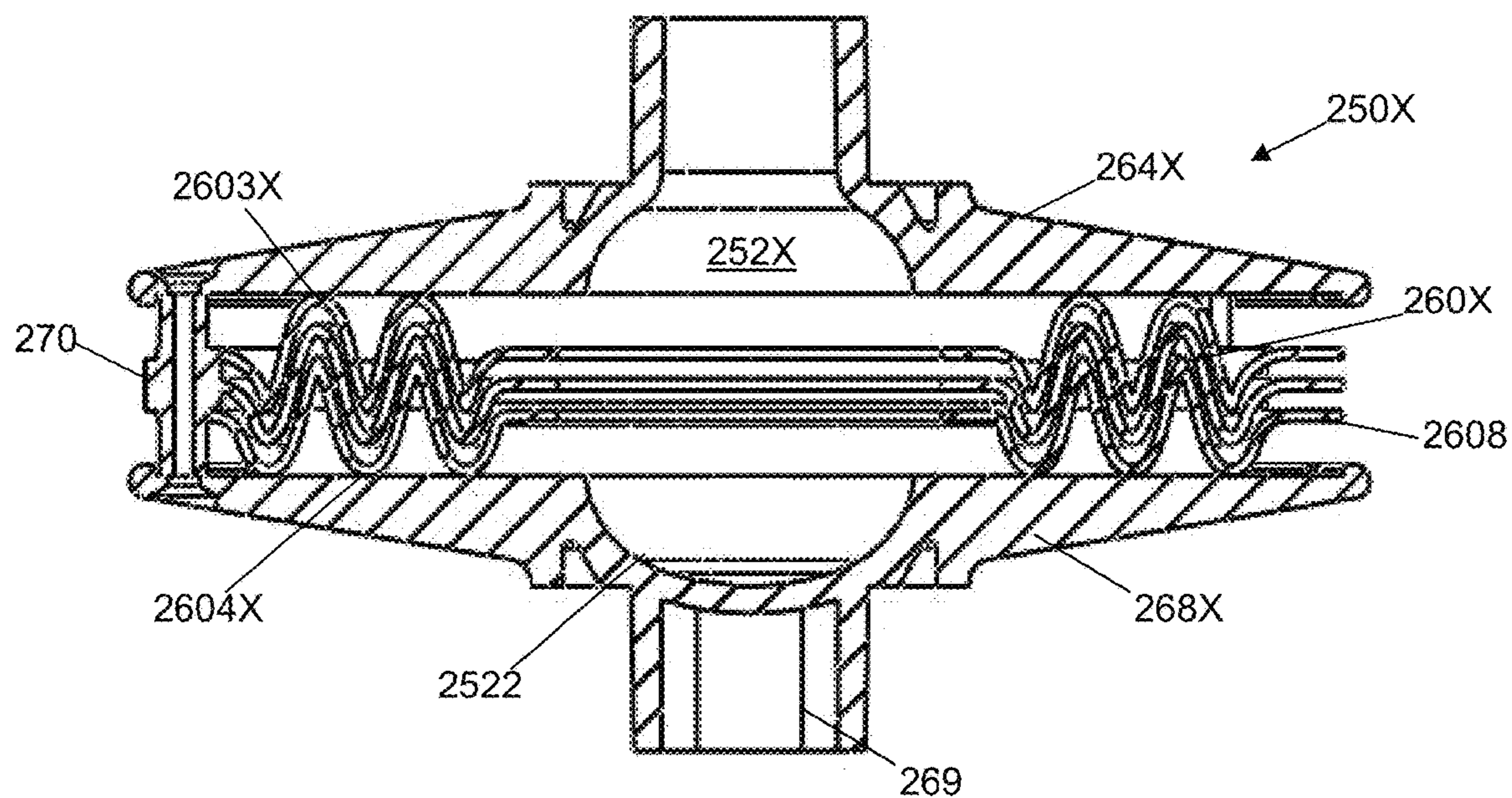
FIG. 18B
