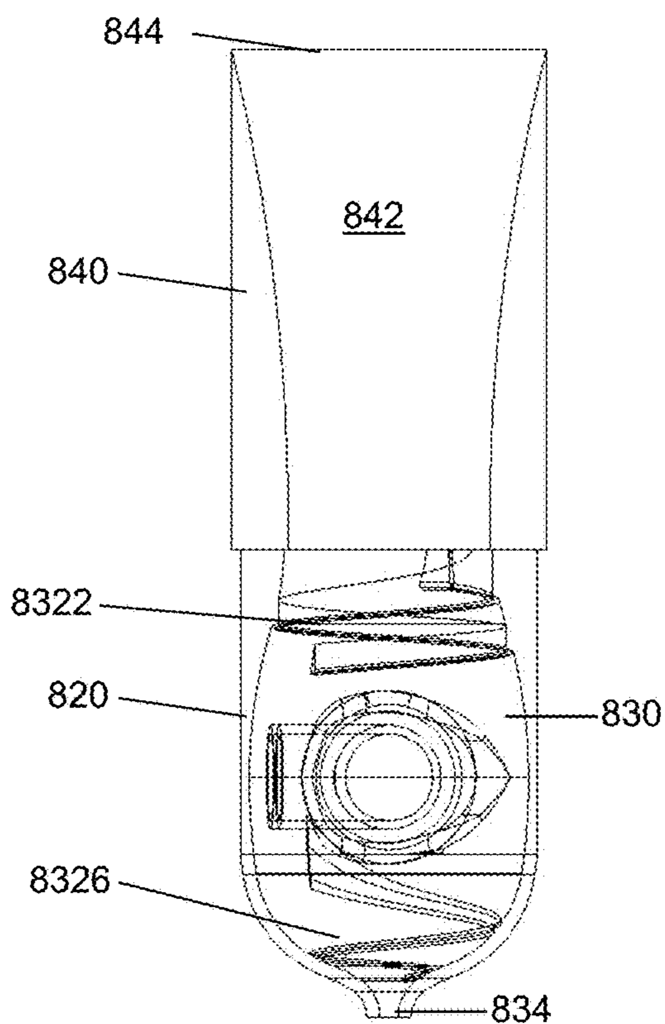
FIG. 6
