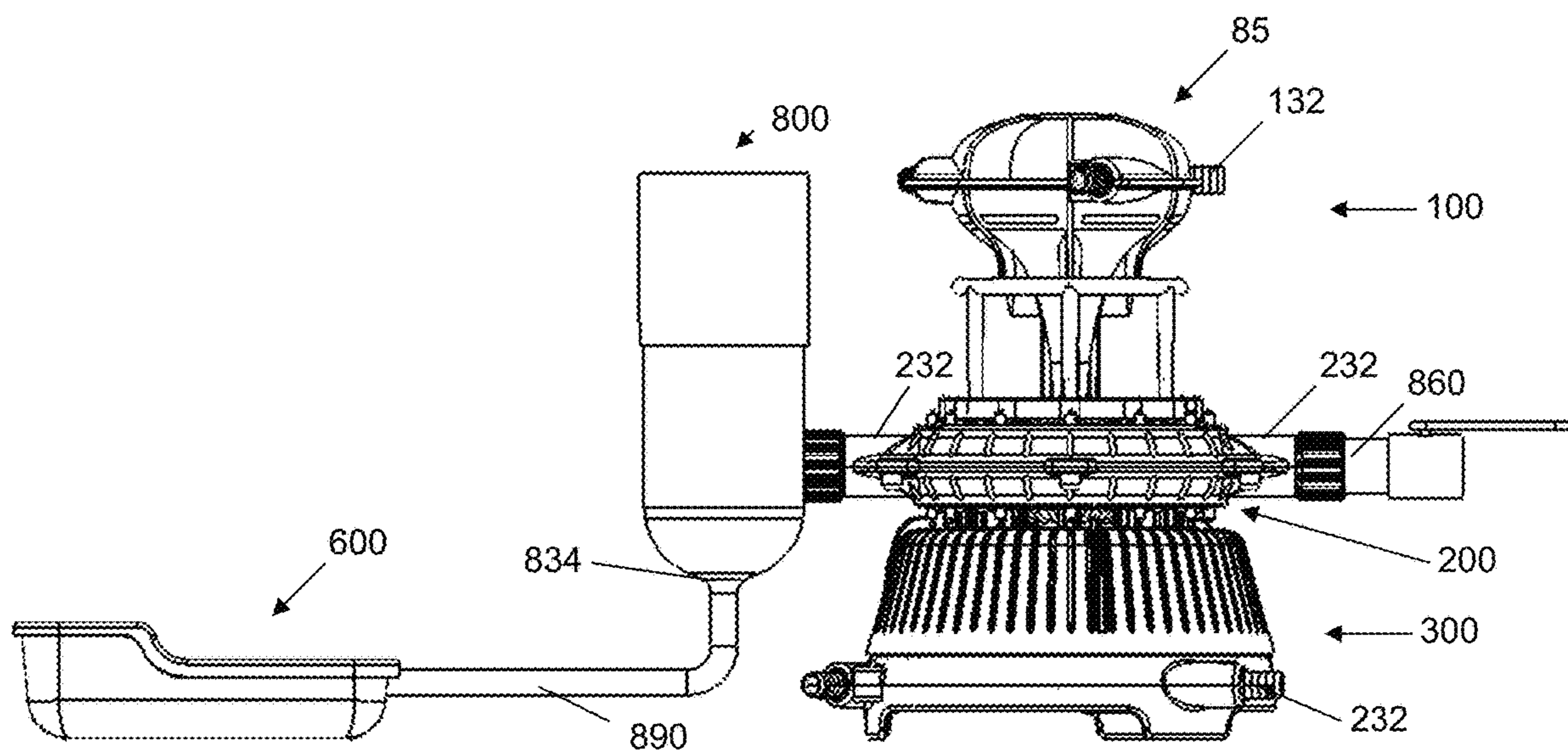
FIG. 10A
