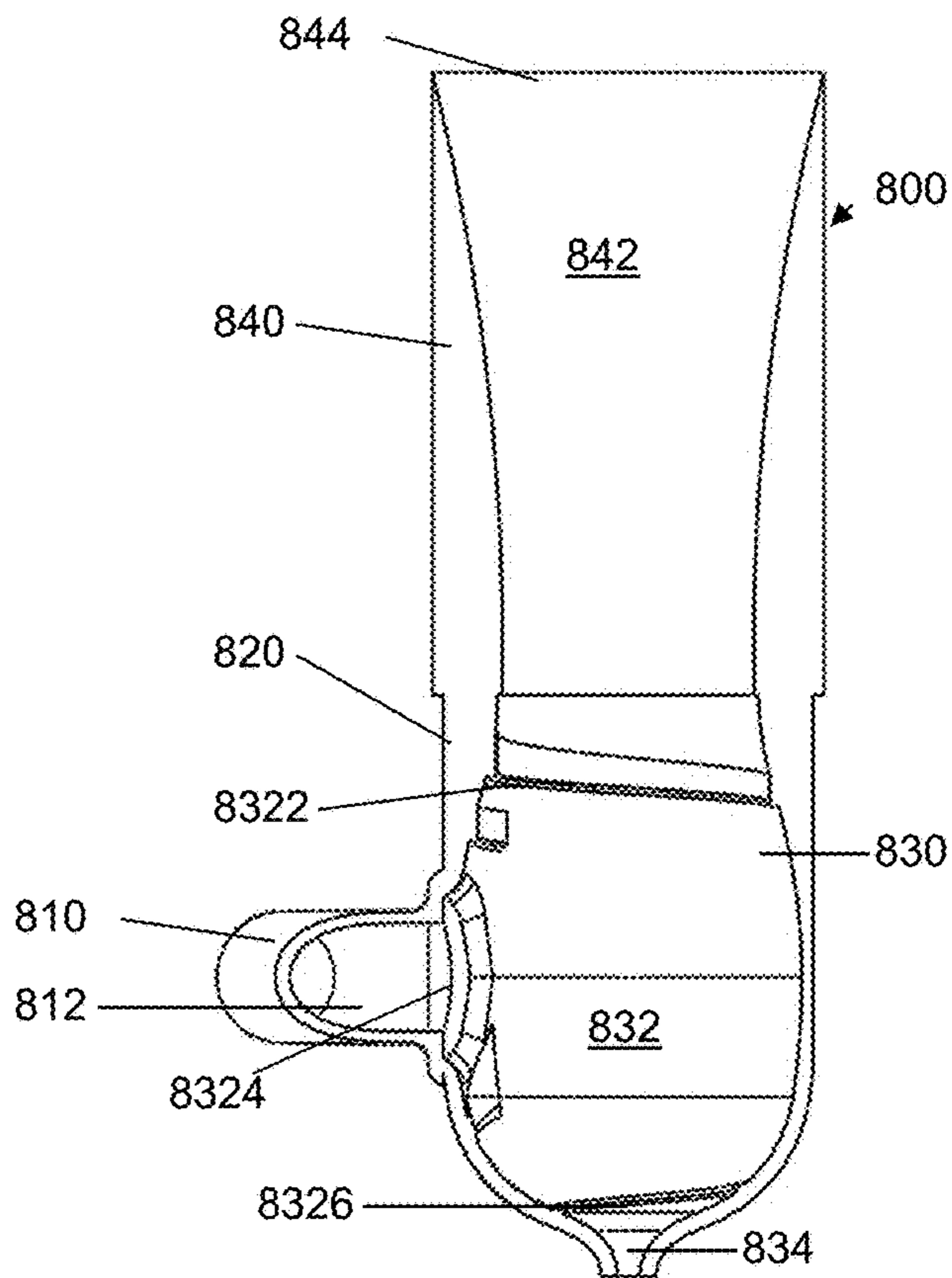
FIG. 5
