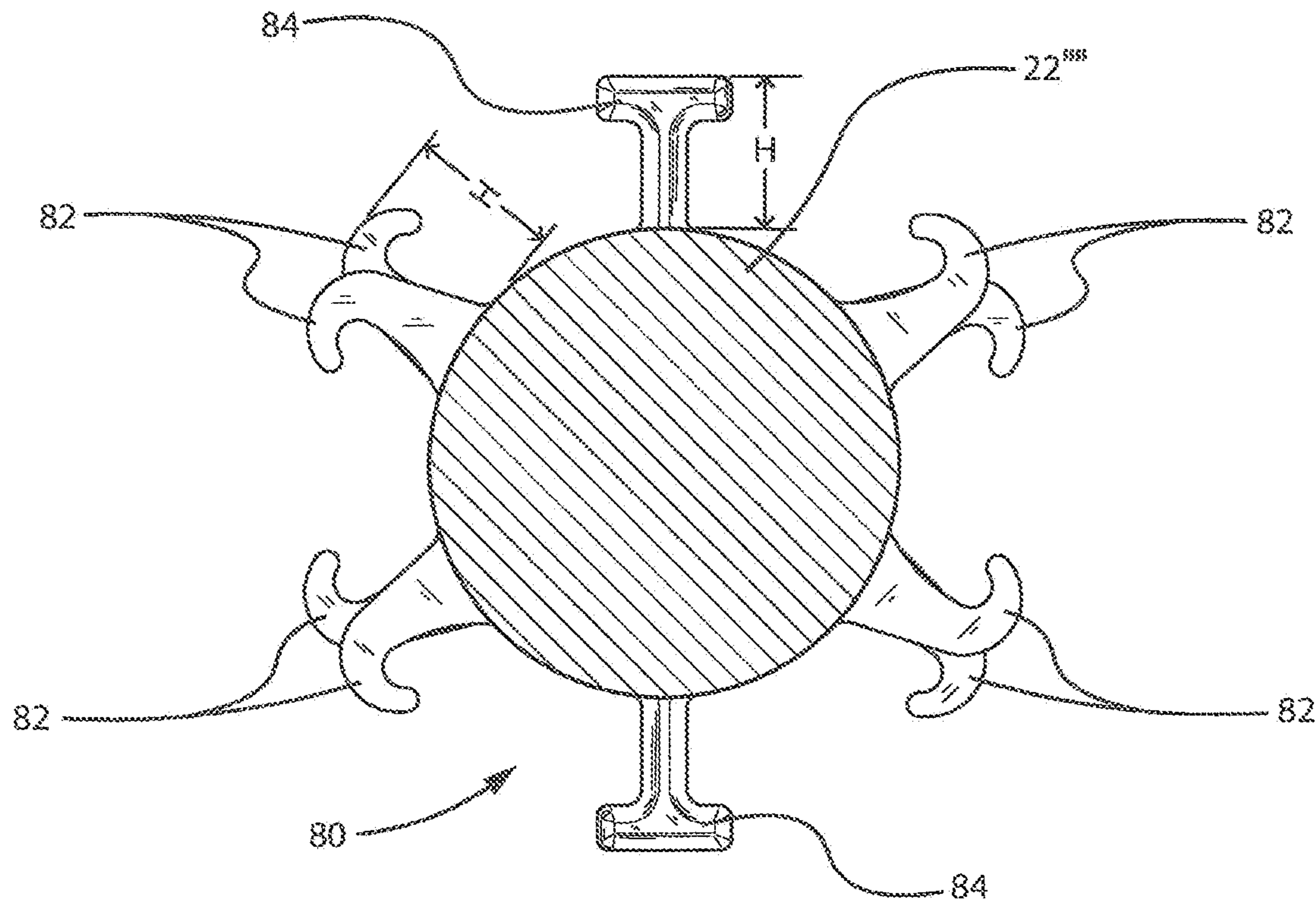
Section B-B FIG. 11
