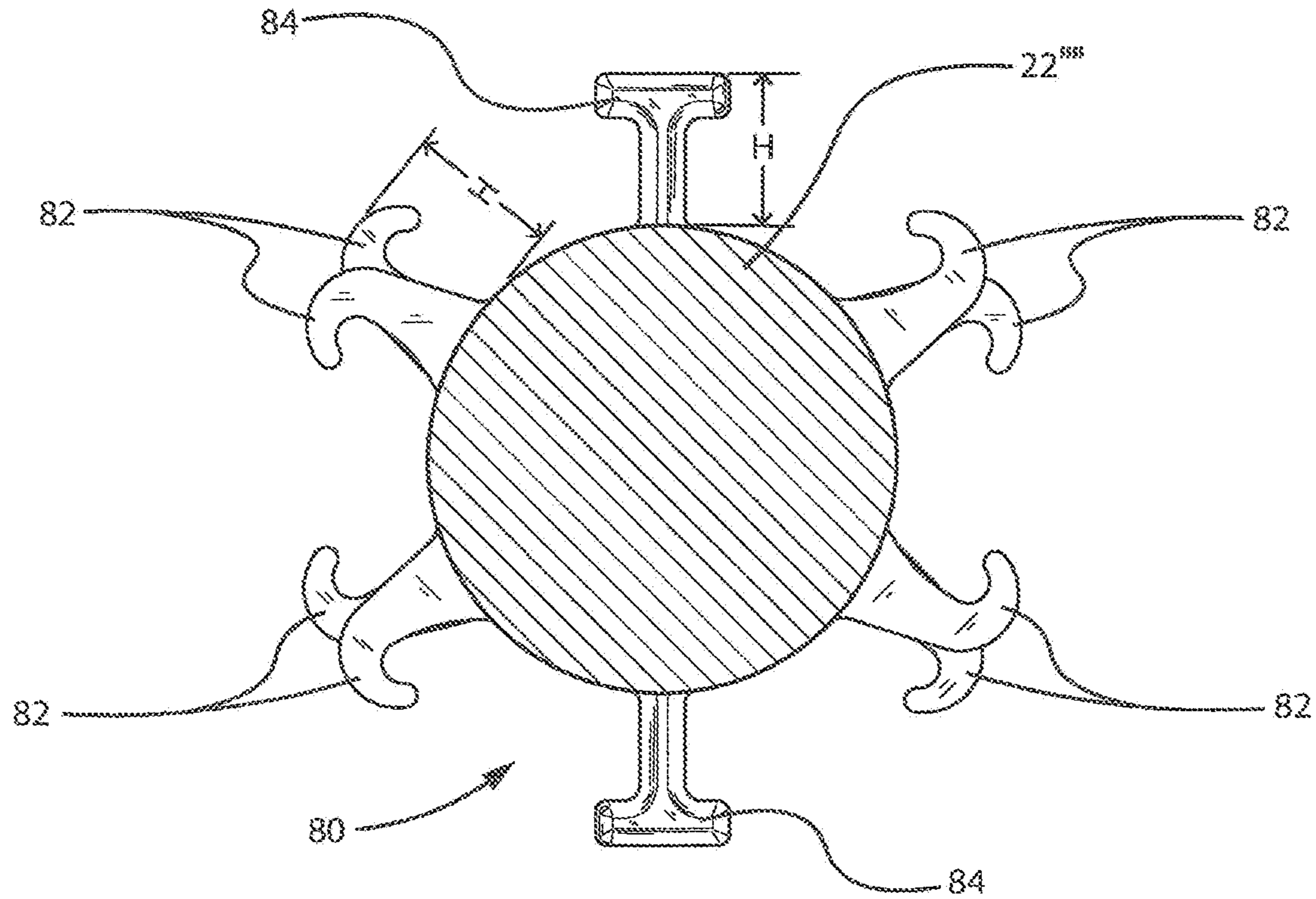
Section B-B FIG. 11
