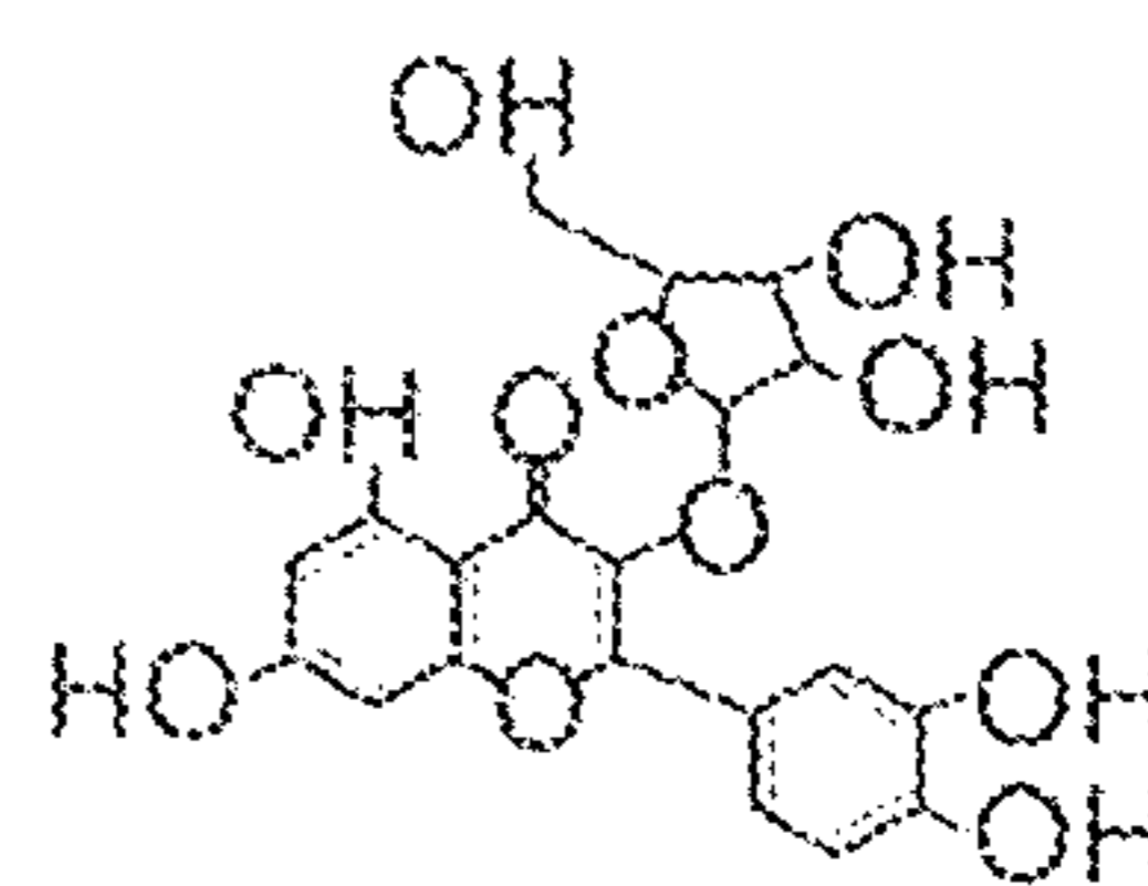
Quercetin 3-arabinofuranoside
