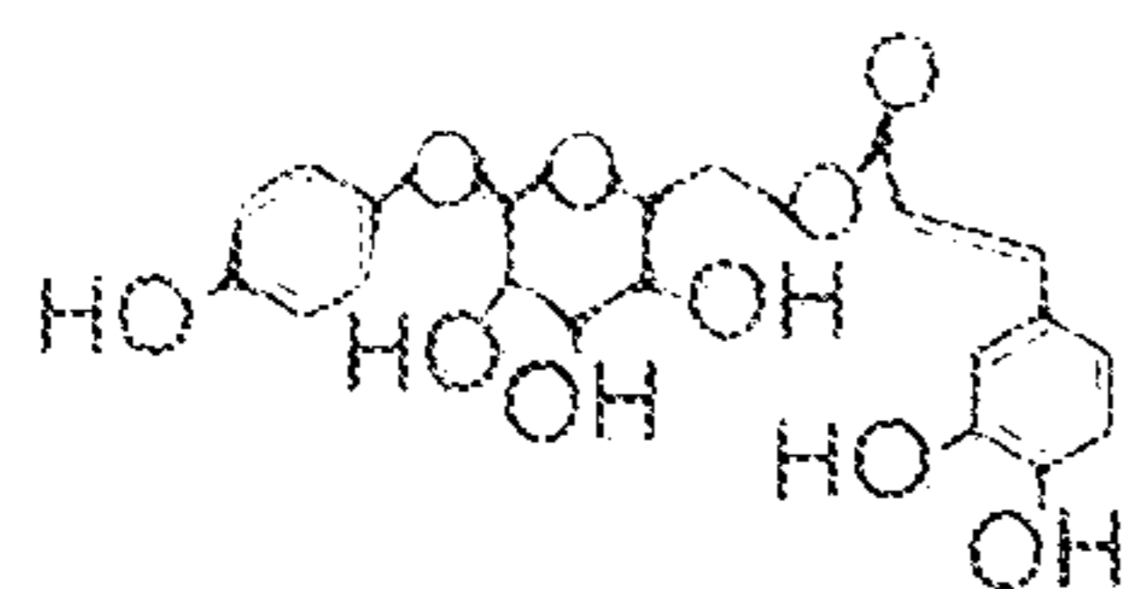
6'-O-trans-Caffeoylarbutin
