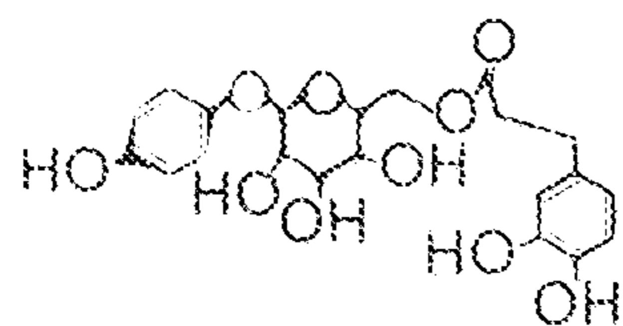
6'-O-trans-Caffeoylarbutin
