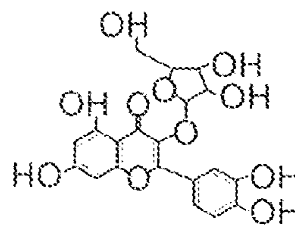
Quercetin 3-arabinofuranoside
