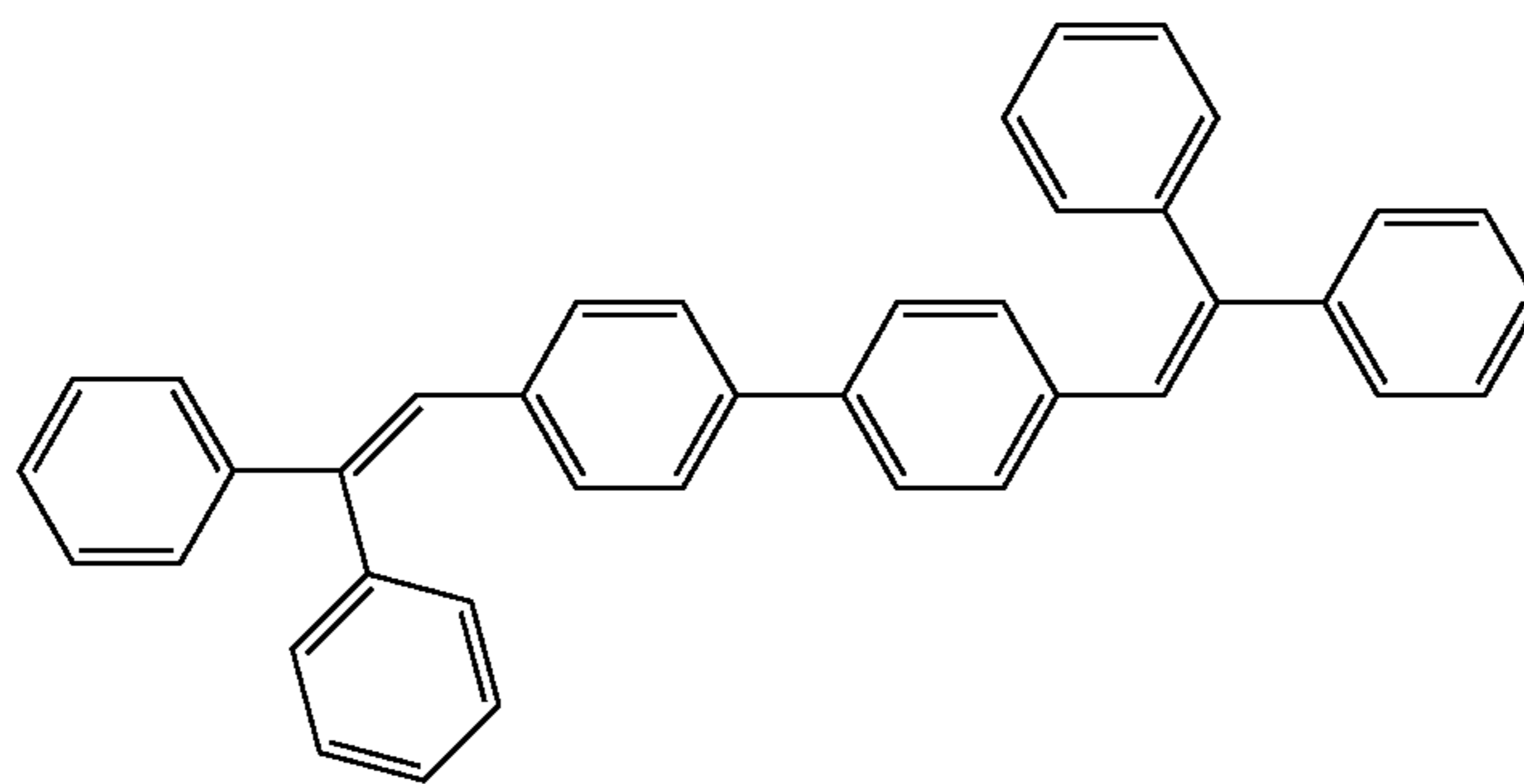
DPVBi
