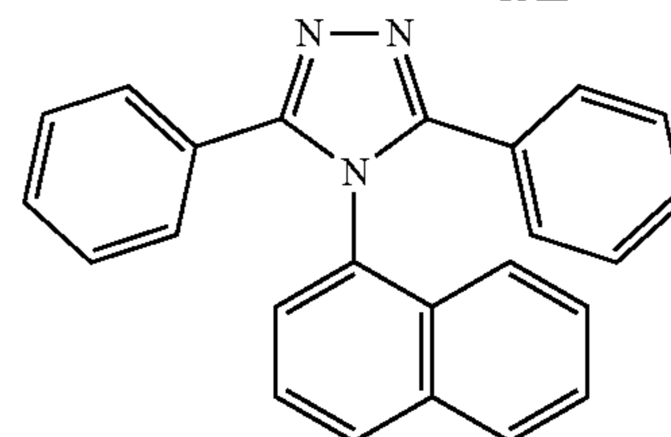
NTAZ
