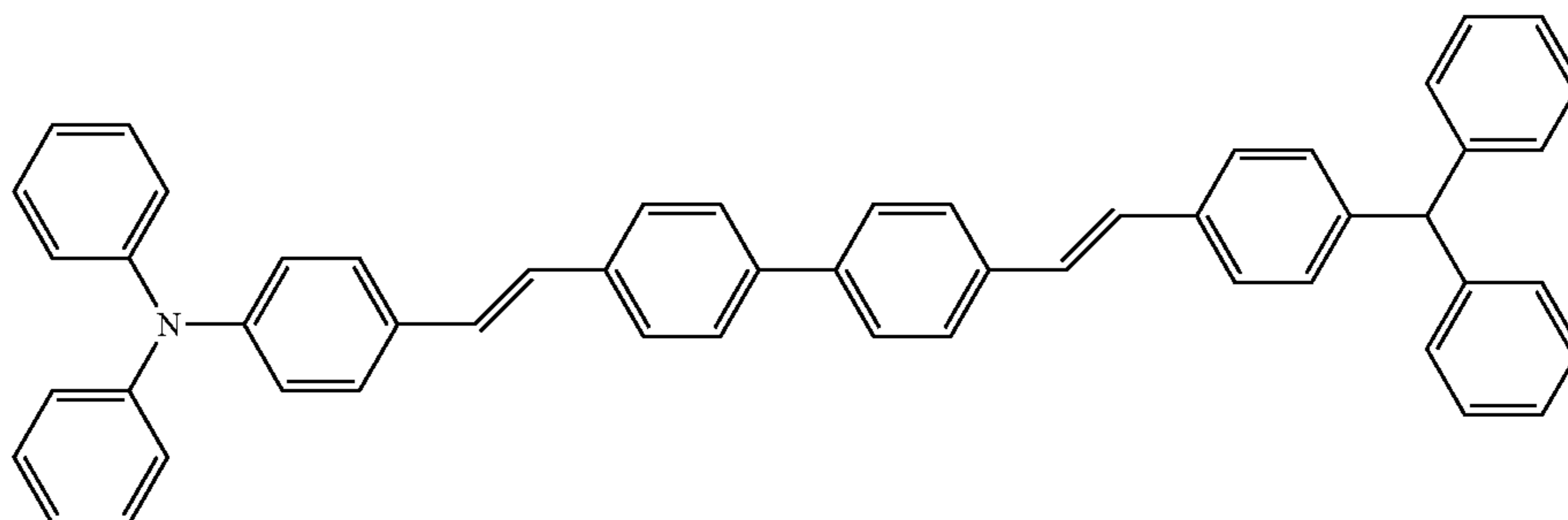
DPAVBi
