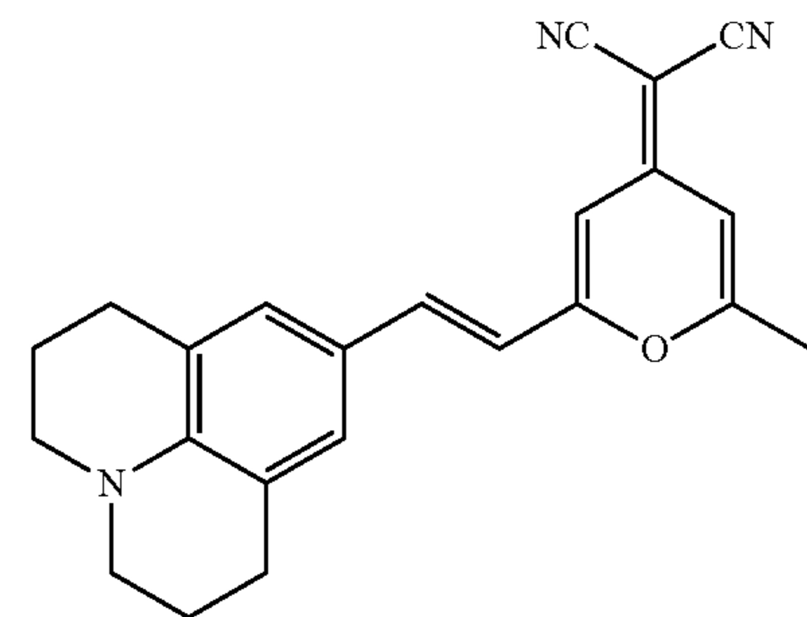
DCM
