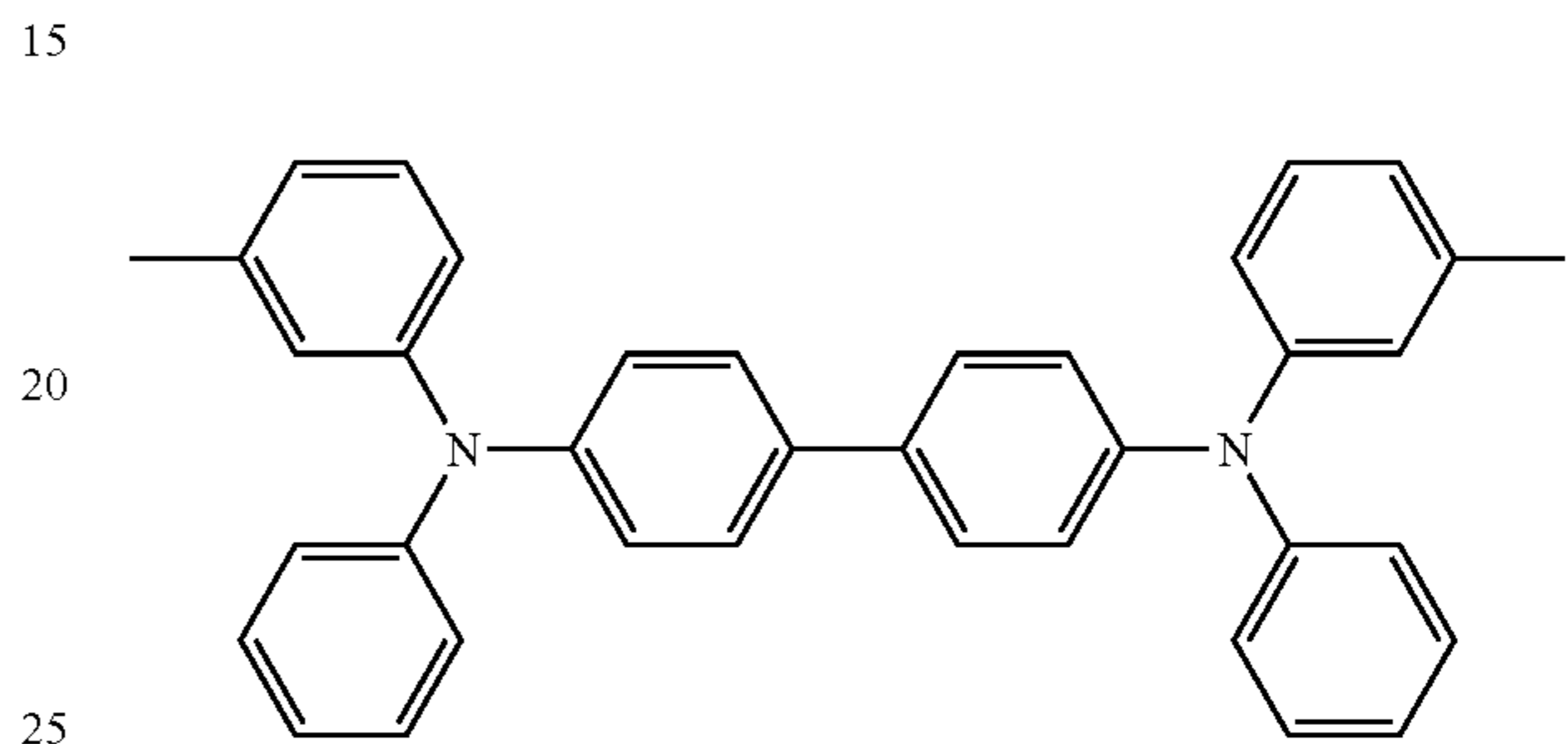
TPD
