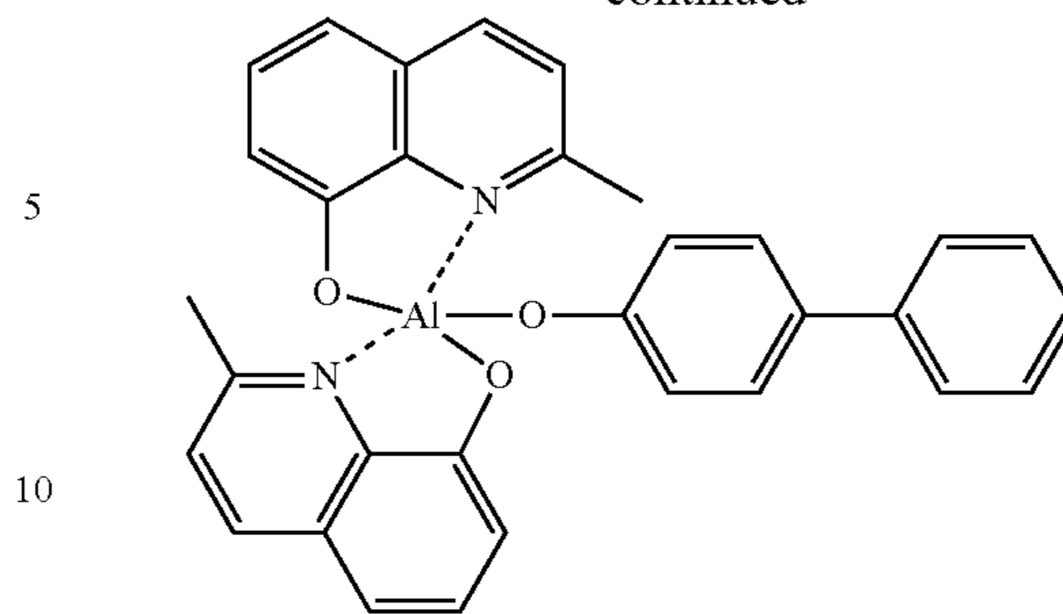
BAlq
