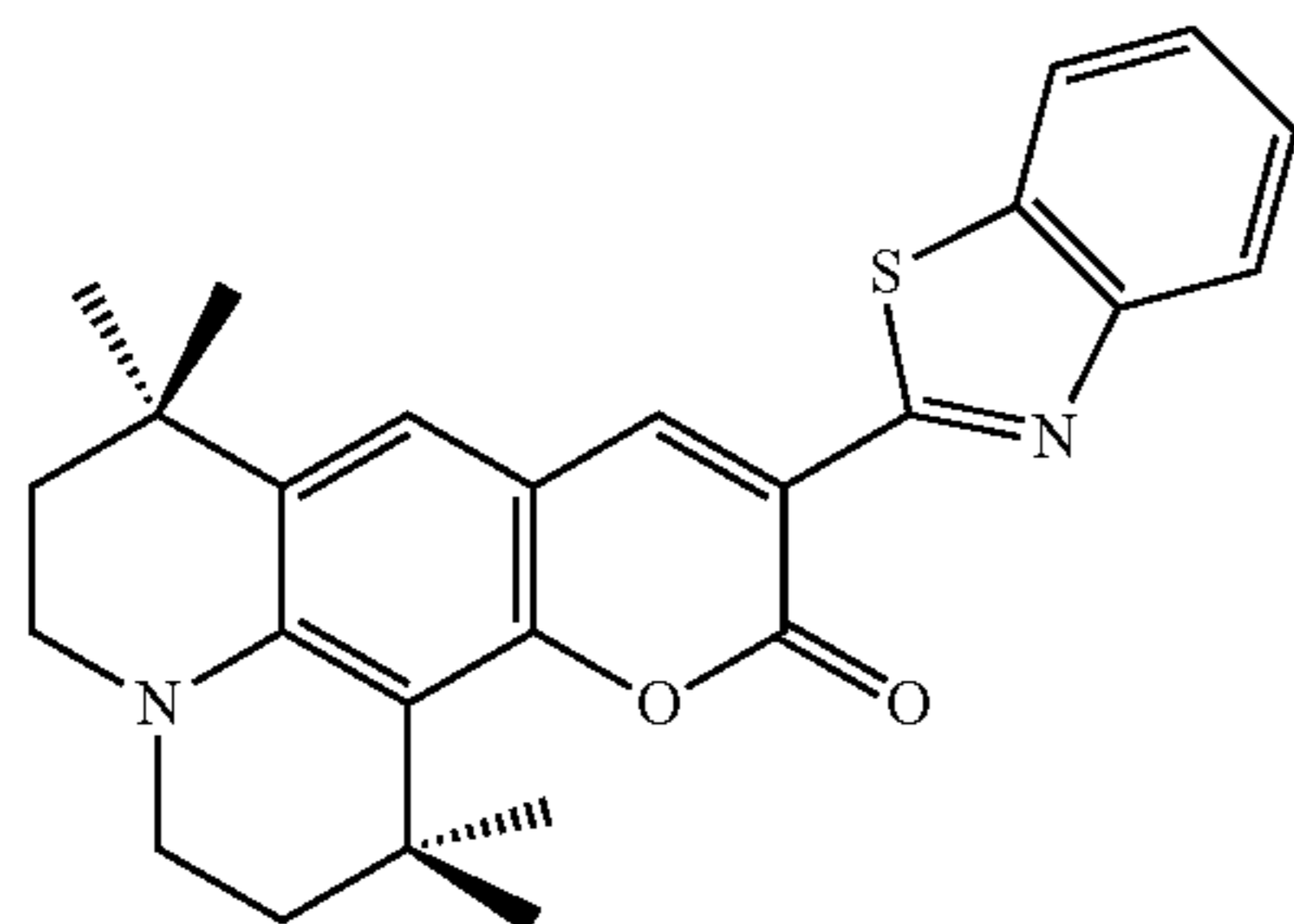
C545T
