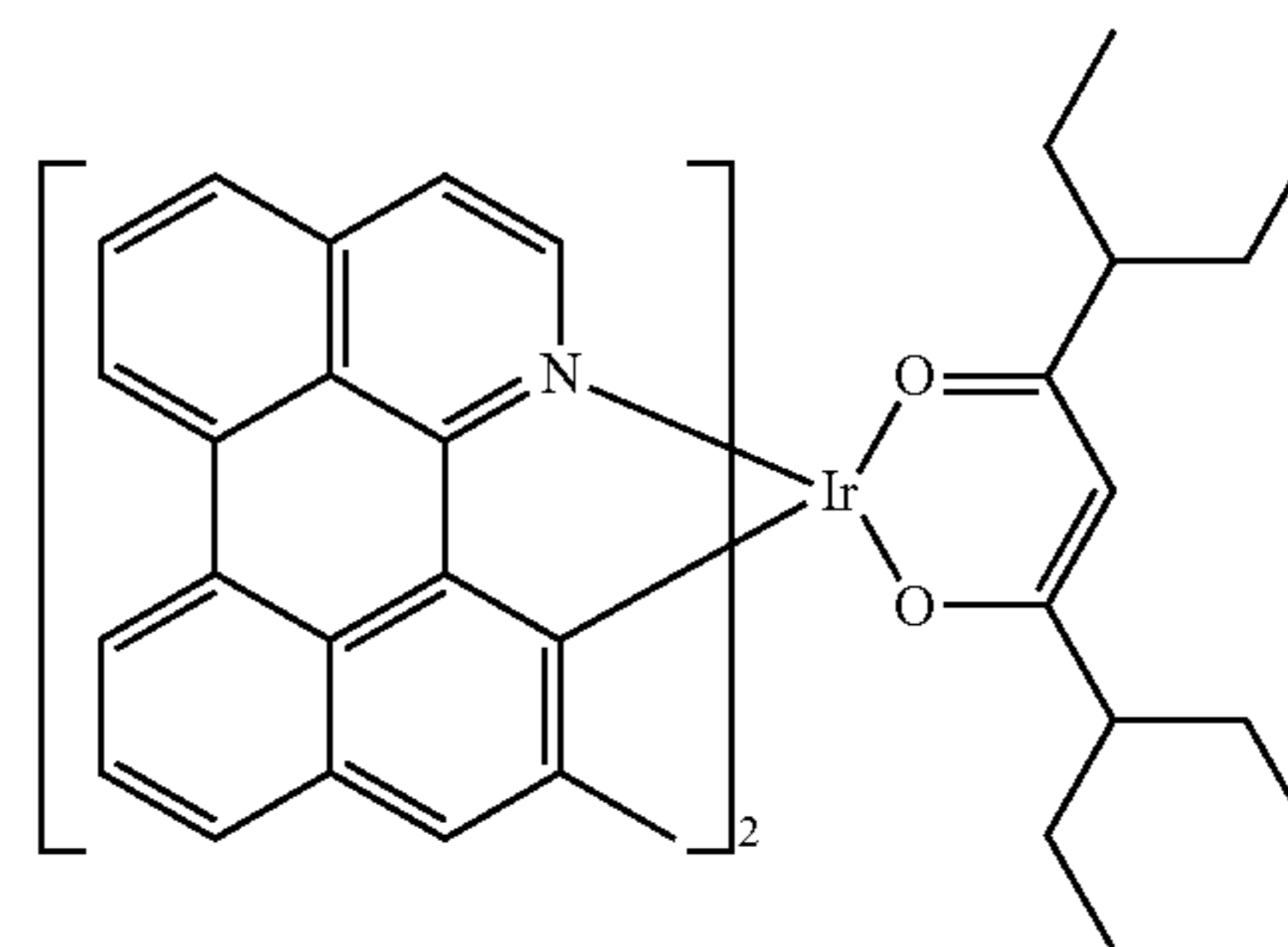
Ir(L_{A85-II})_2L_{B20}
