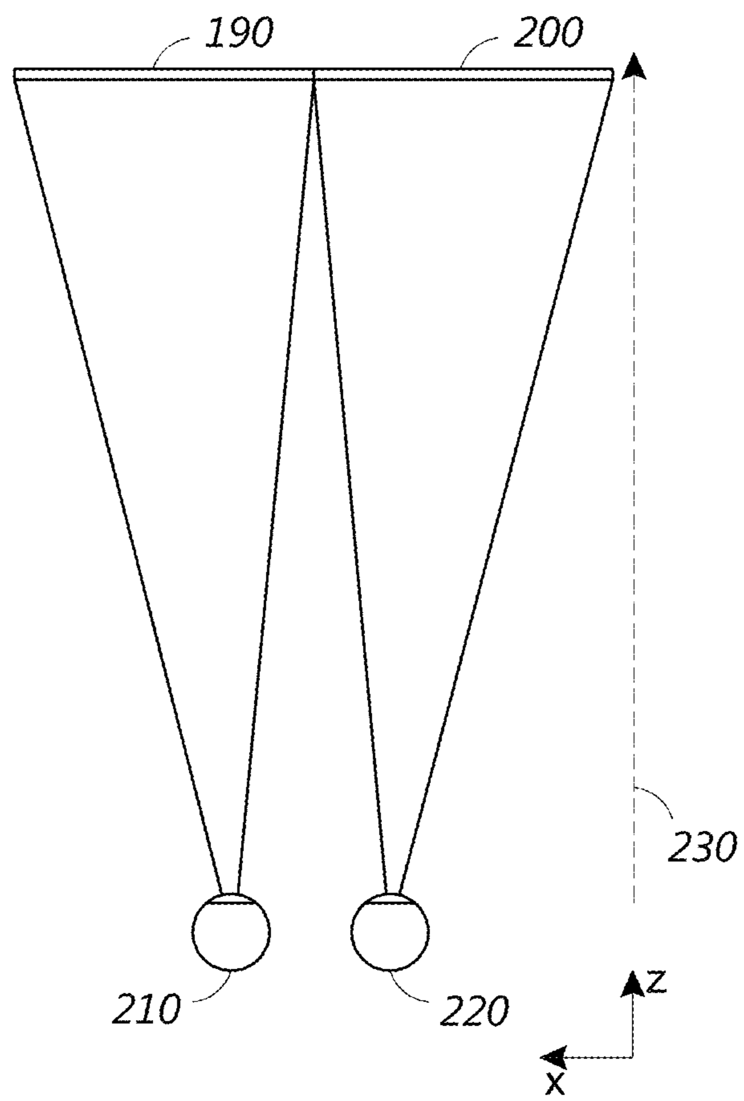
FIG. 2
