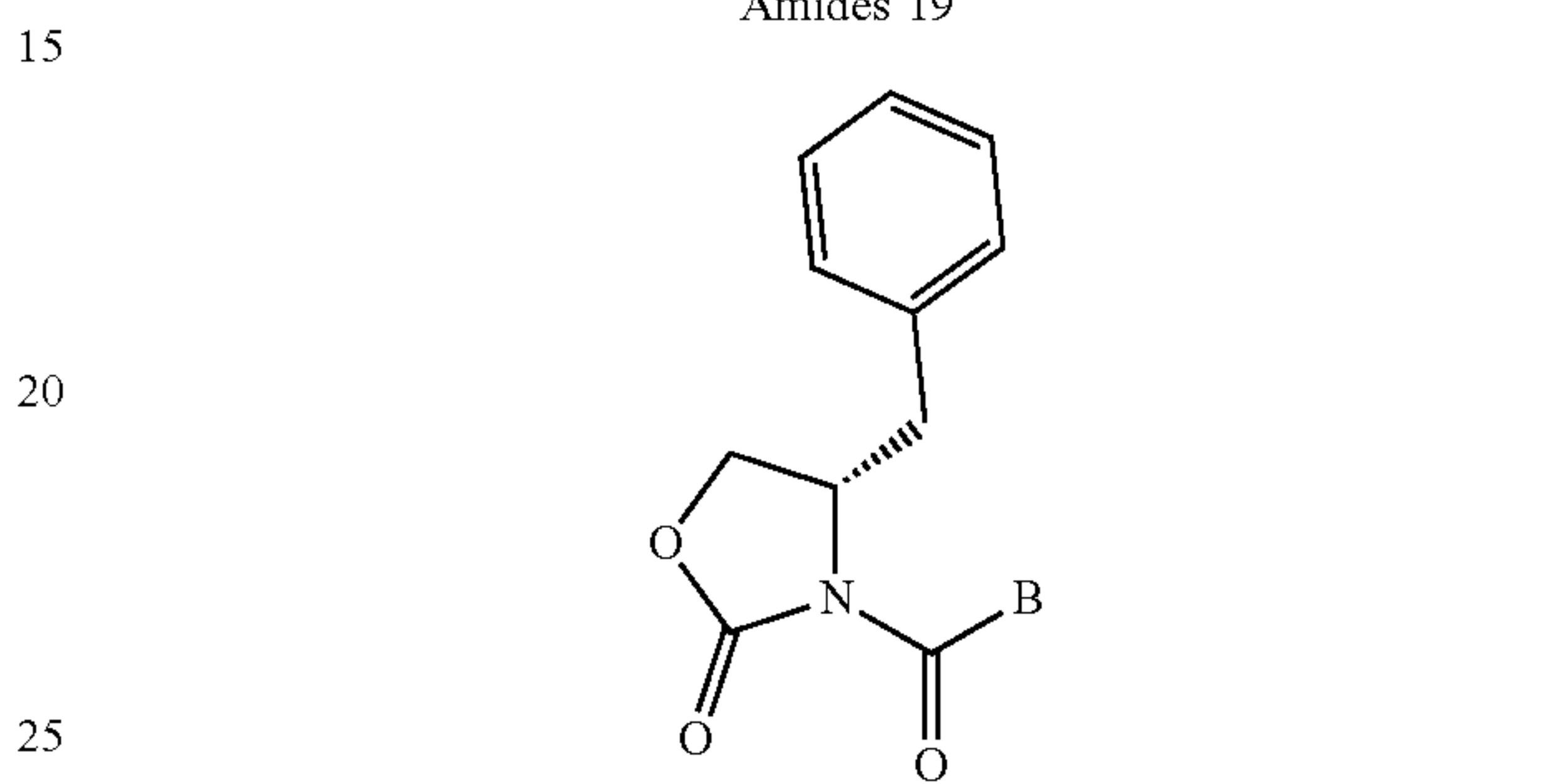
(S)-3-(B-Carbonyl)-4-benzyloxazolidin-2-ones 21
