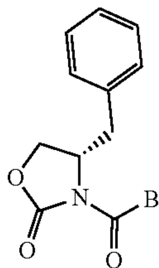
(S)-3-(B-Carbonyl)-4-benzyloxazolidin-2-ones 21
