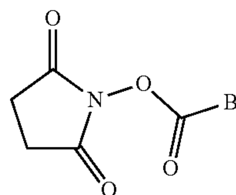
NHS Esters
