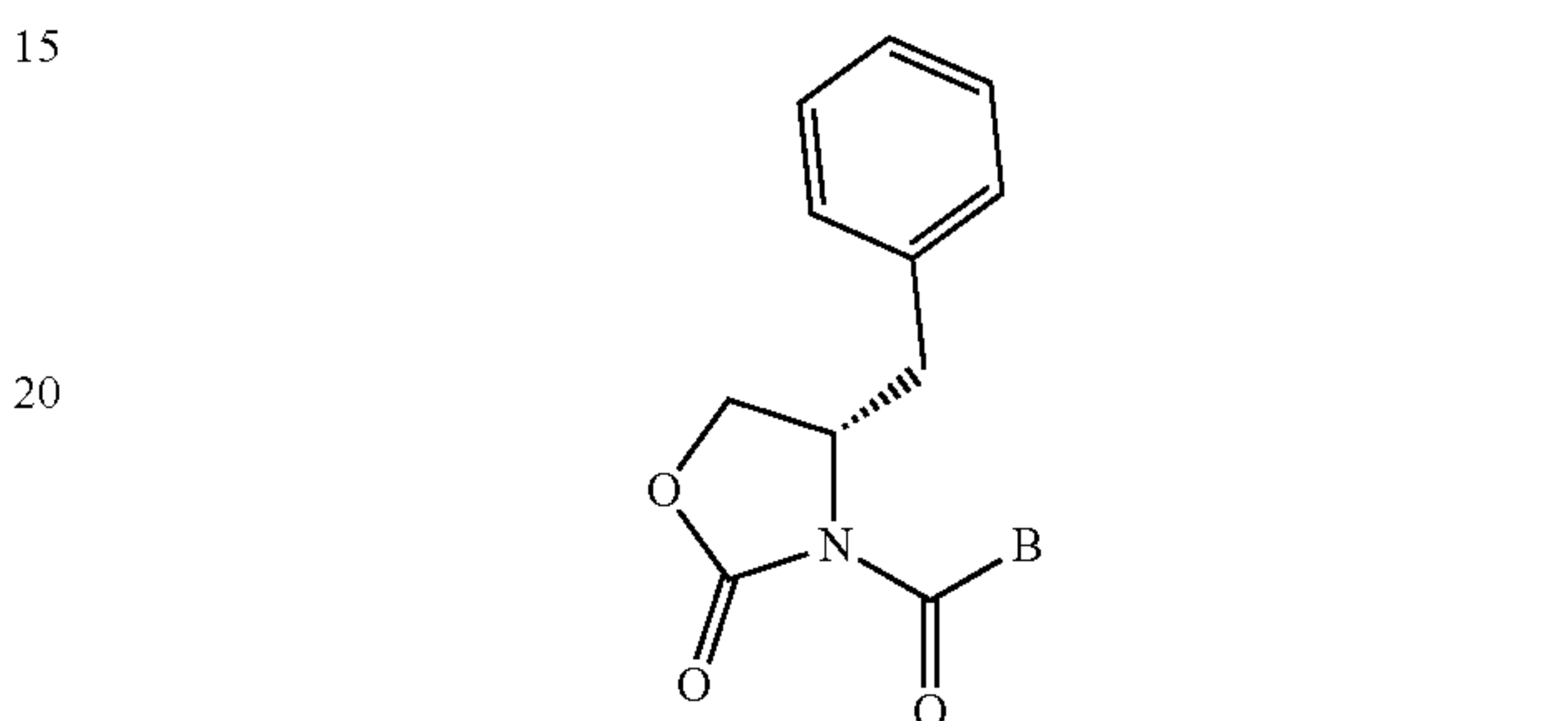
(S)-3-(B-Carbonyl)-4-benzyloxazolidin-2-ones 21
