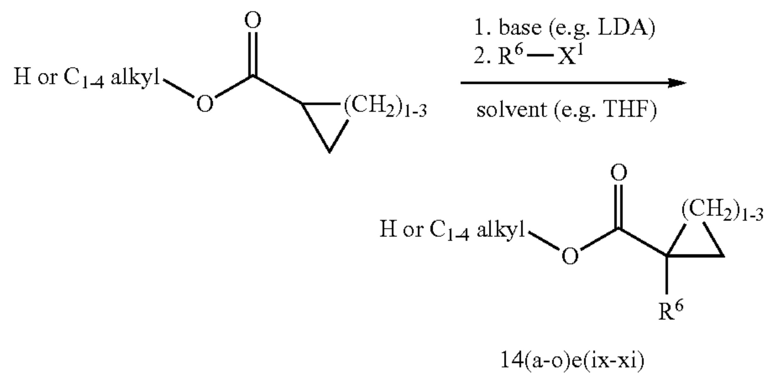
Scheme 7e
