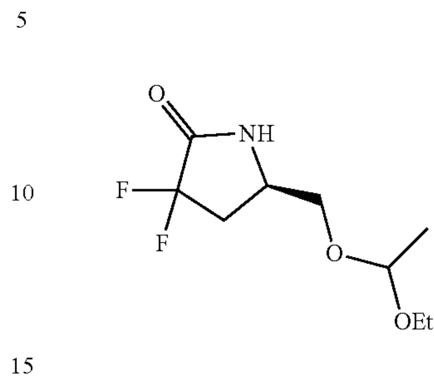
Scheme 3, Step H: Preparation of (5R)-5-((1-ethoxyethoxy)methyl)-3,3-difluoropyrrolidin-2-one (9; PG=EE)
