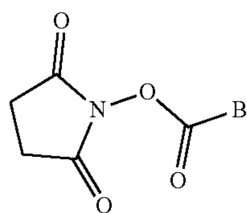
NHS Esters 18
