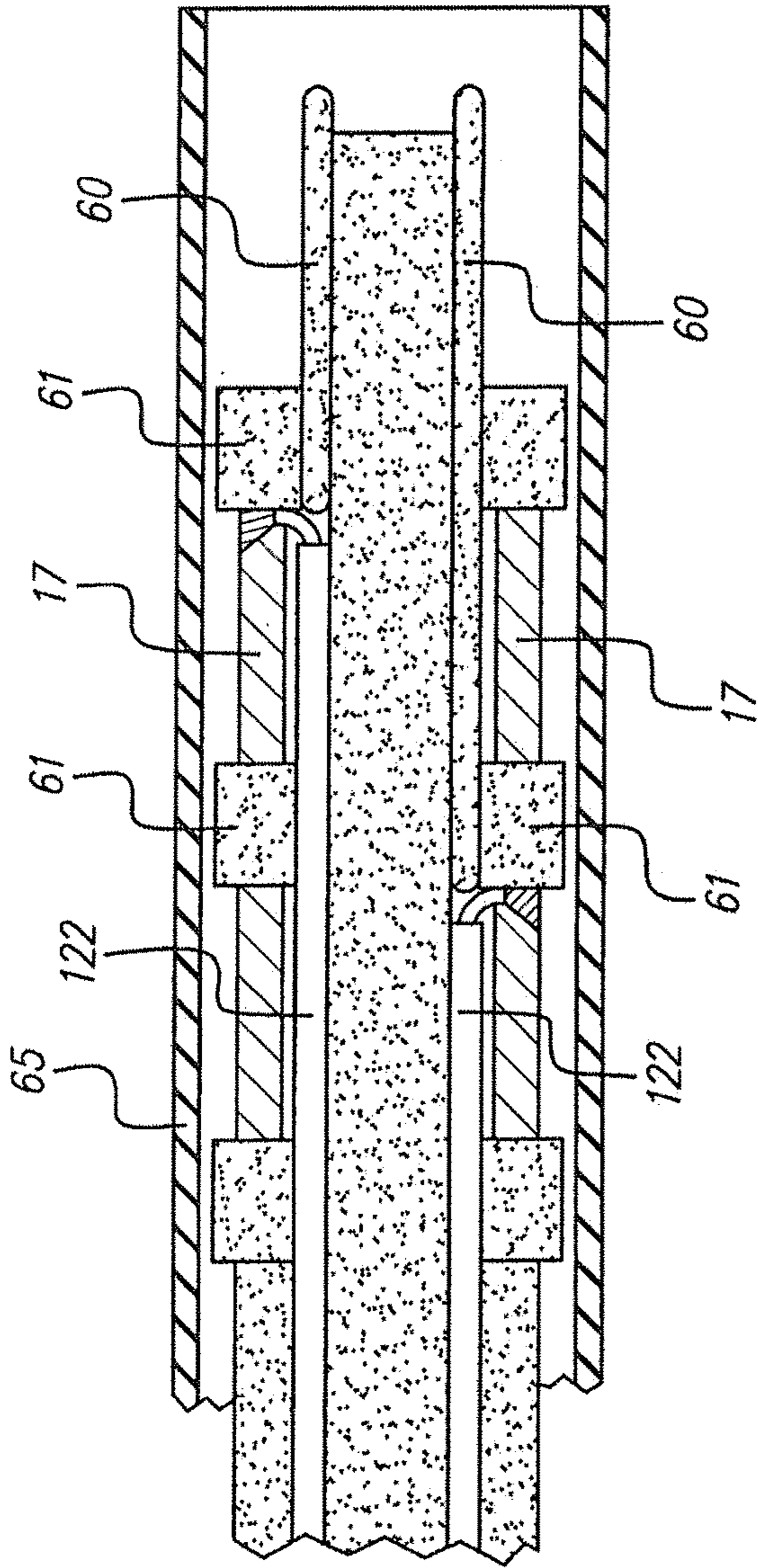
FIG. 6A
