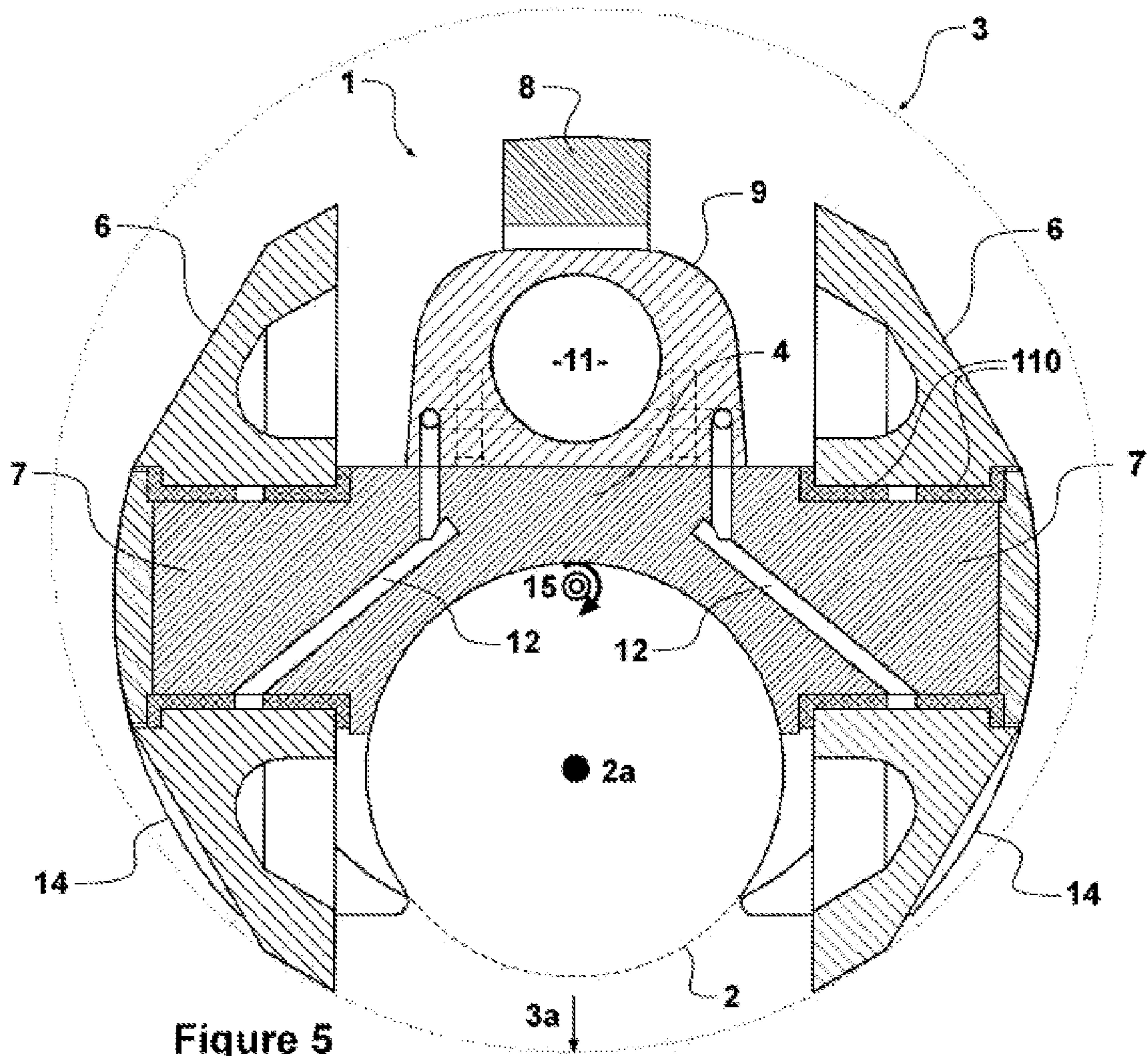
Section A-A
