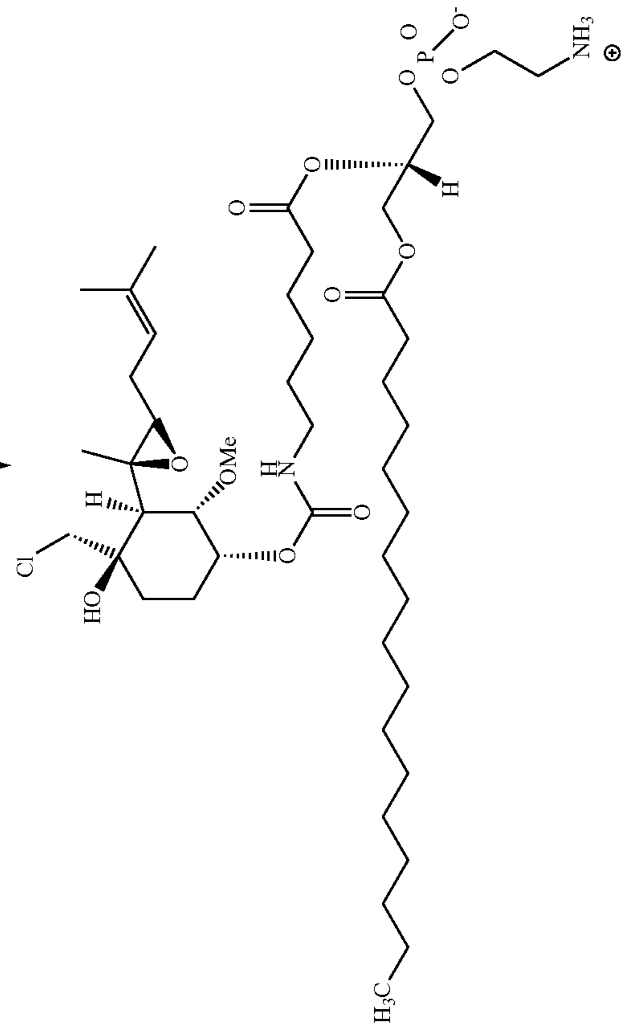
Fumagillin-Prodrug 2
