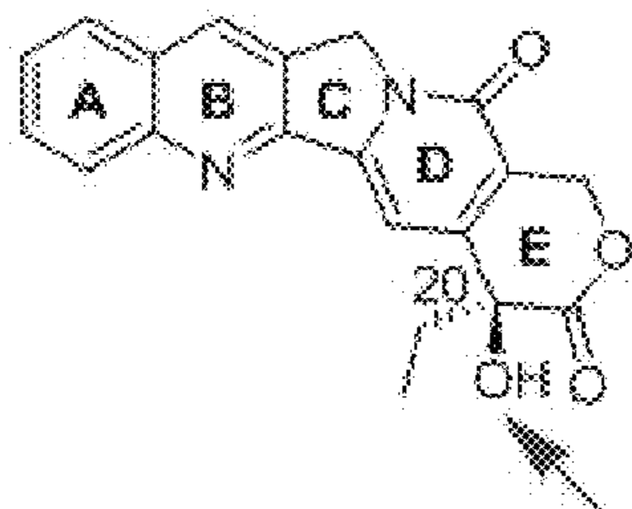
Camptothecin (CPT)
