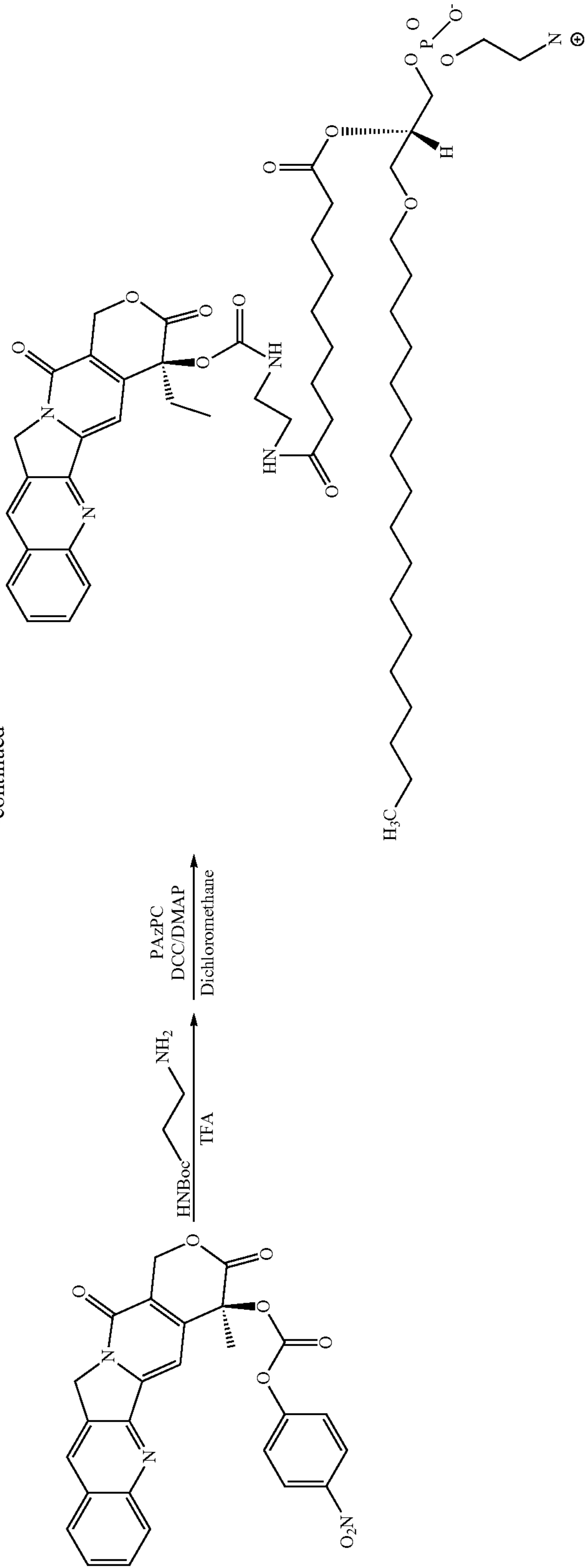
Camptothecin Prodrug 2
