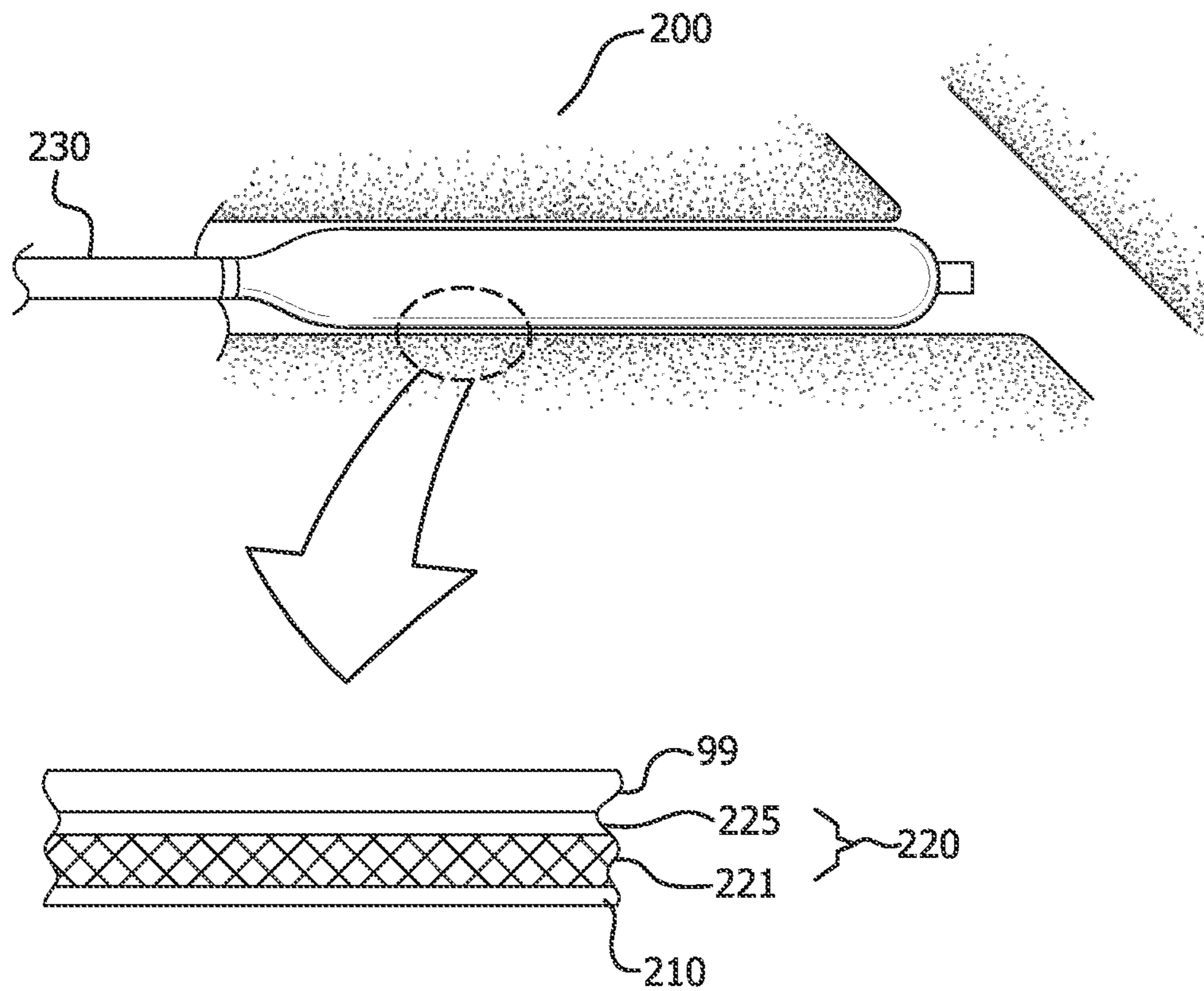
FIG. 2F
