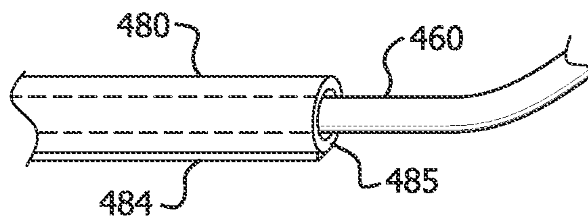
FIG. 4C-1
