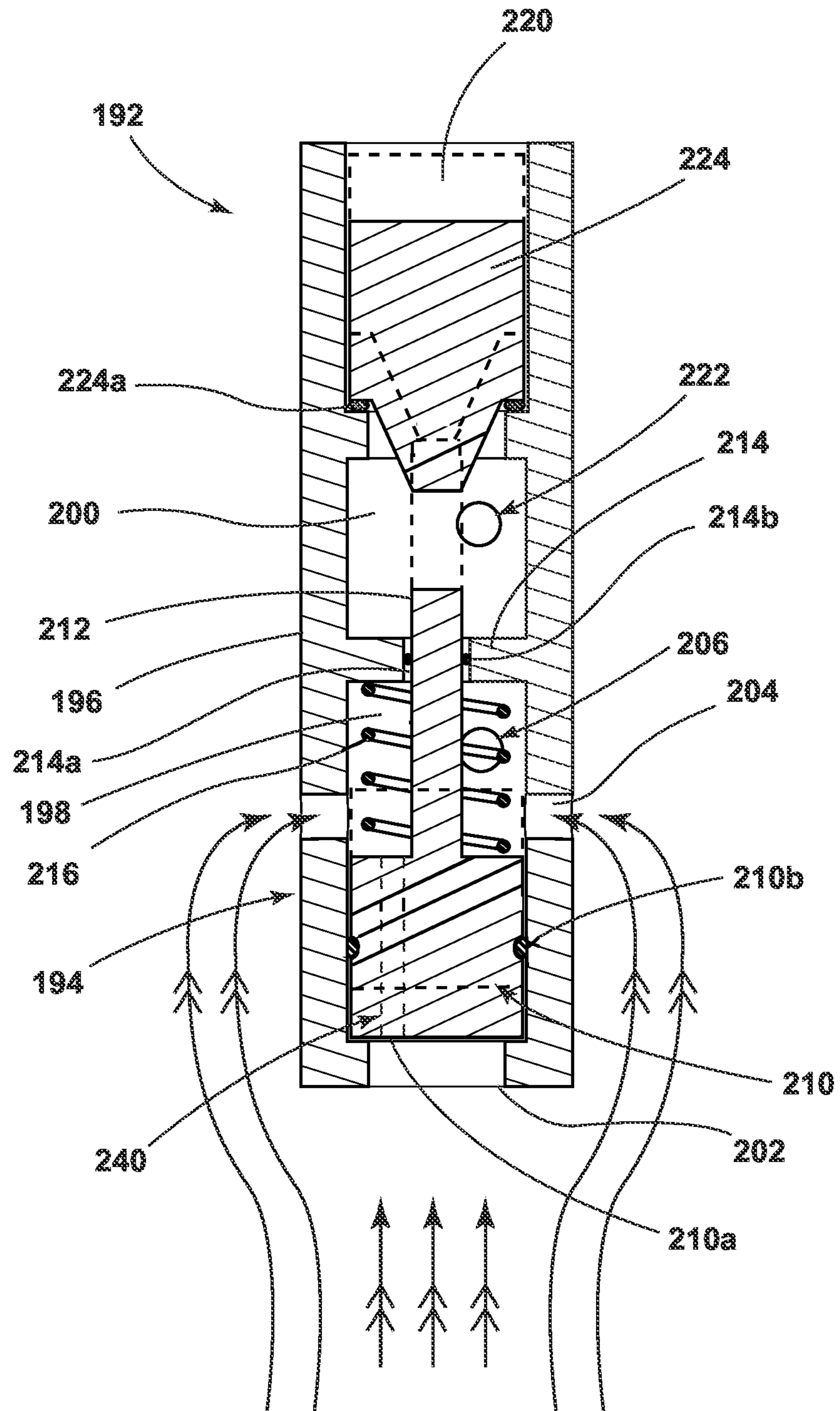
FIG. 15
