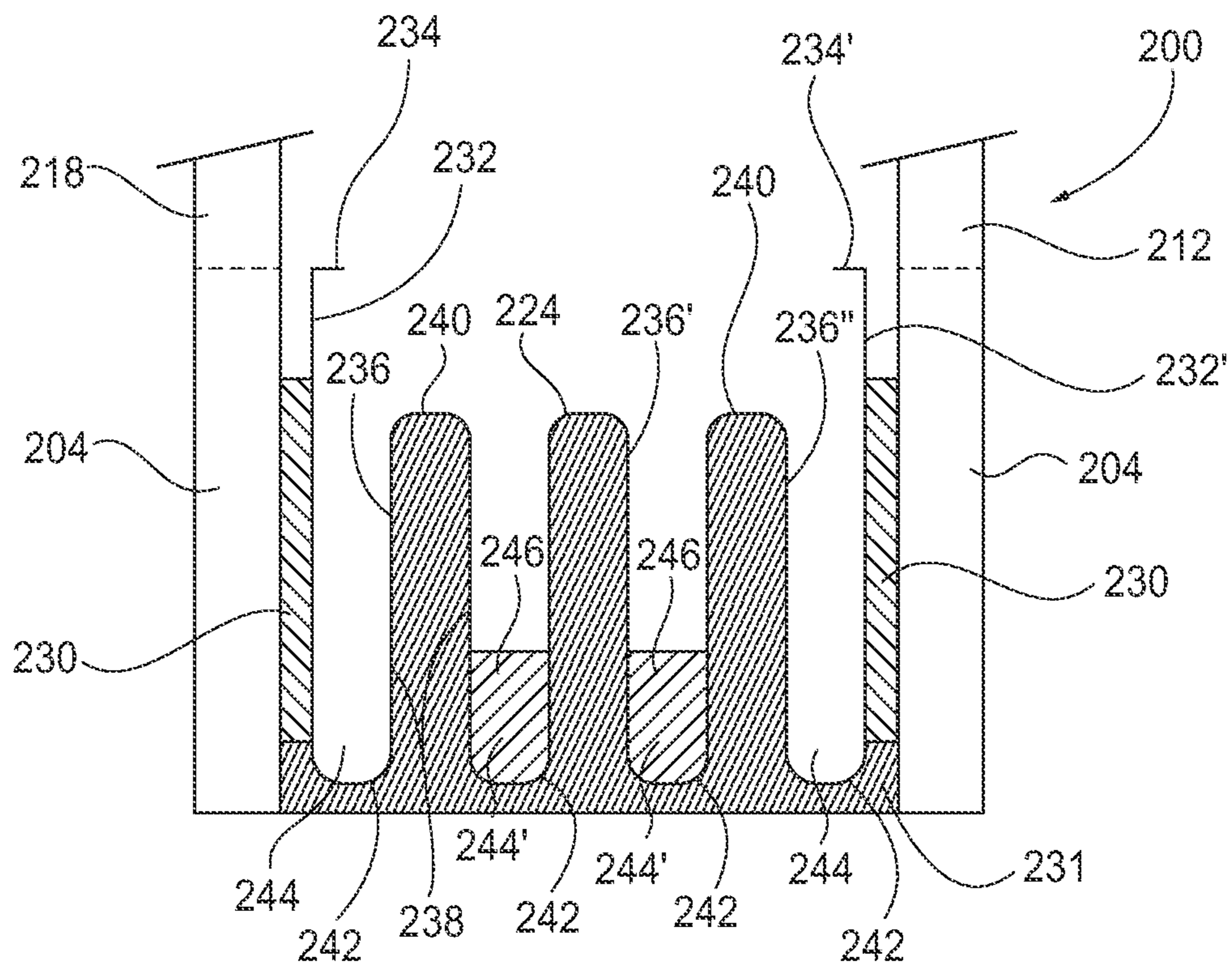
FIG. 3C
