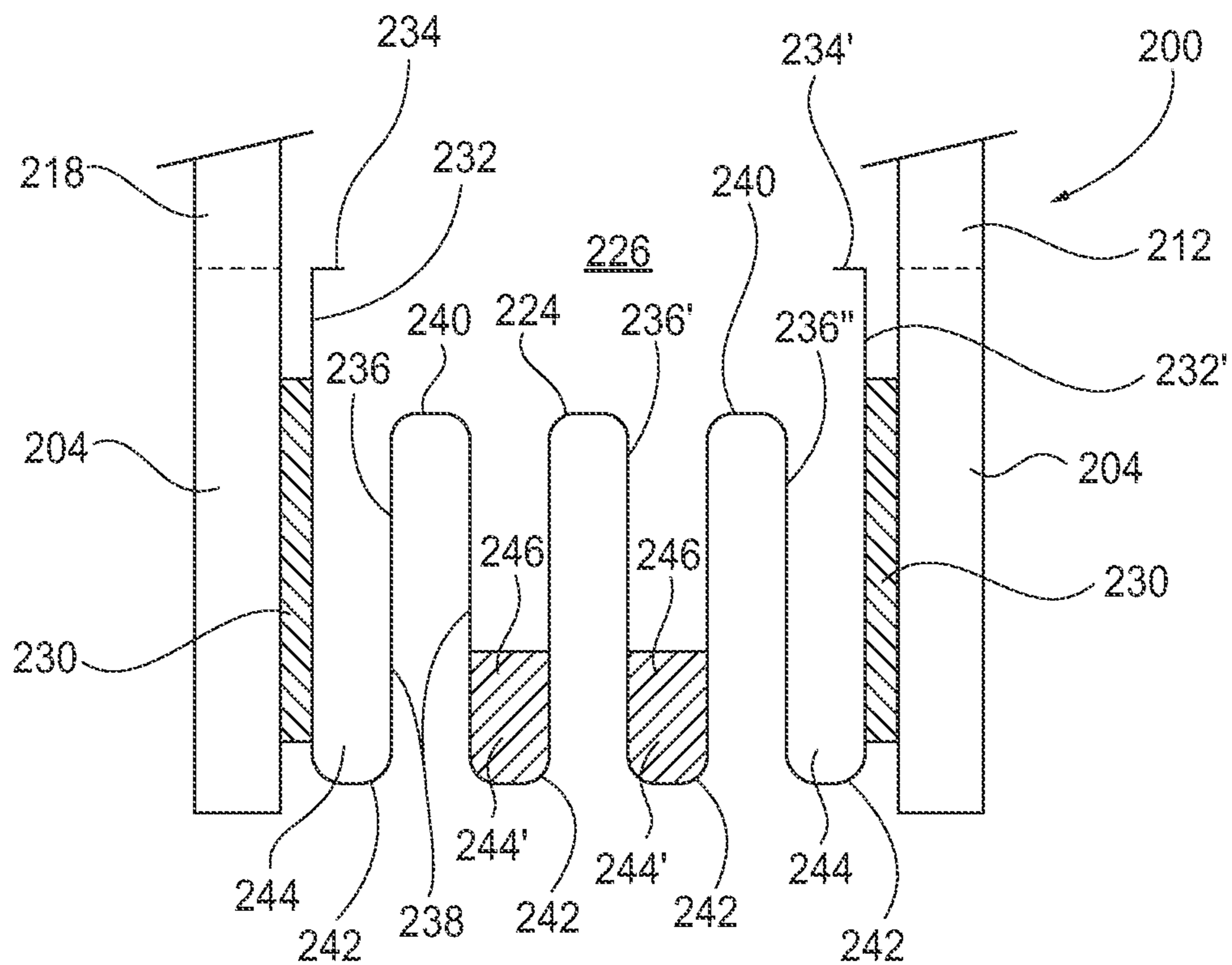
FIG. 3A
