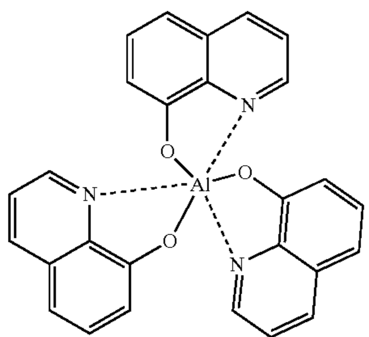
Alq 3
