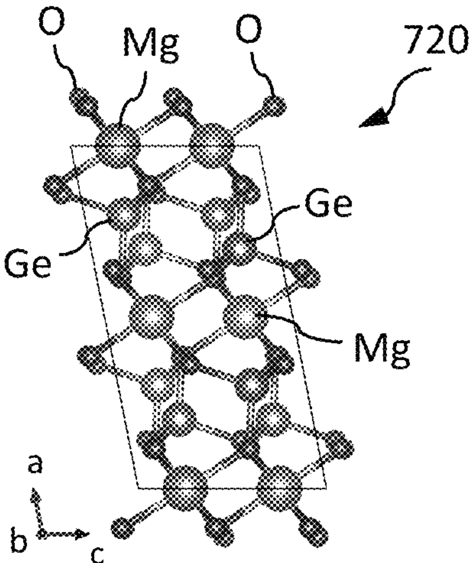
MgGeO 3 (C2/c)
