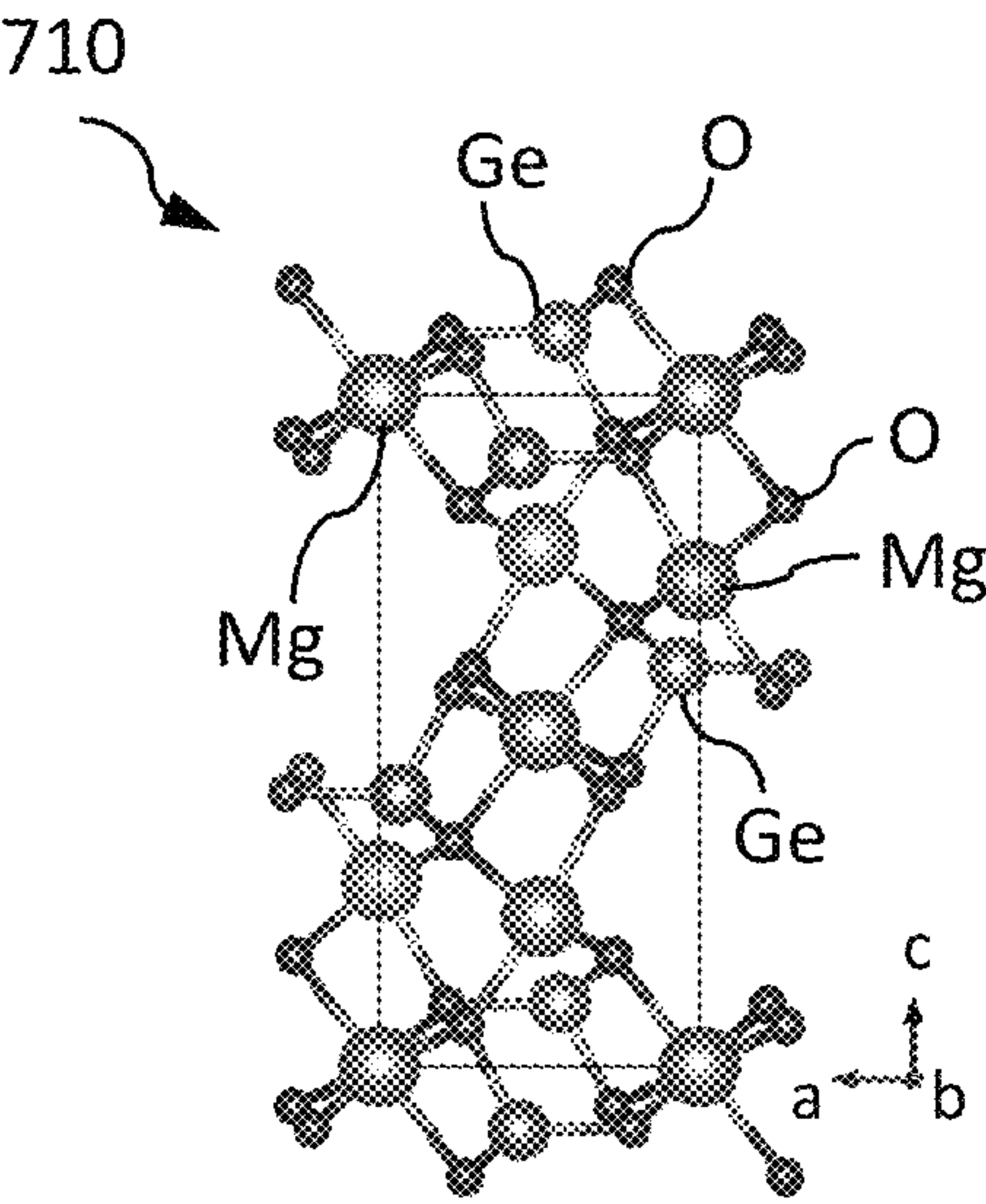
Mg 2 GeO 4 (Pnma)
