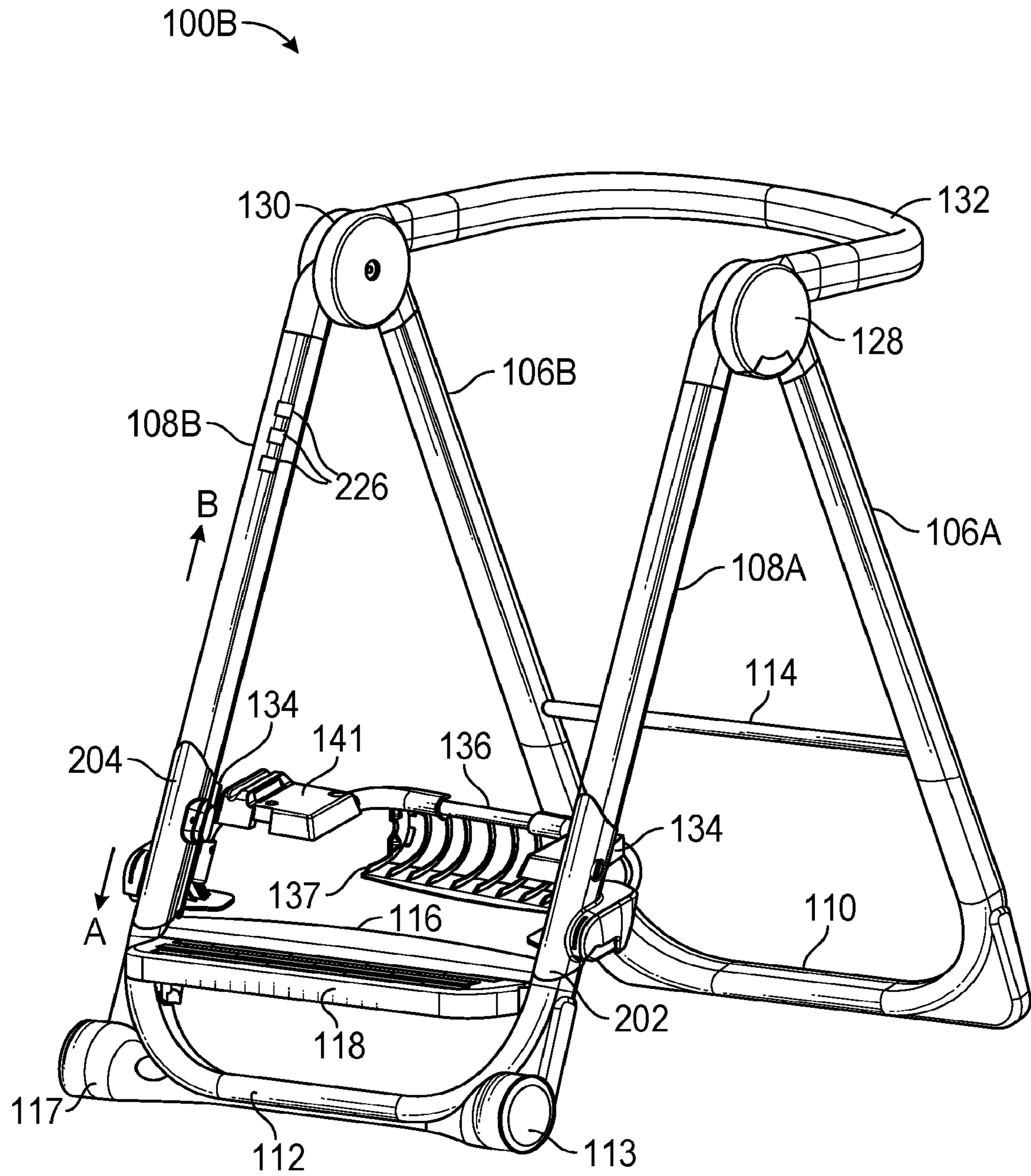
FIG. 2A
