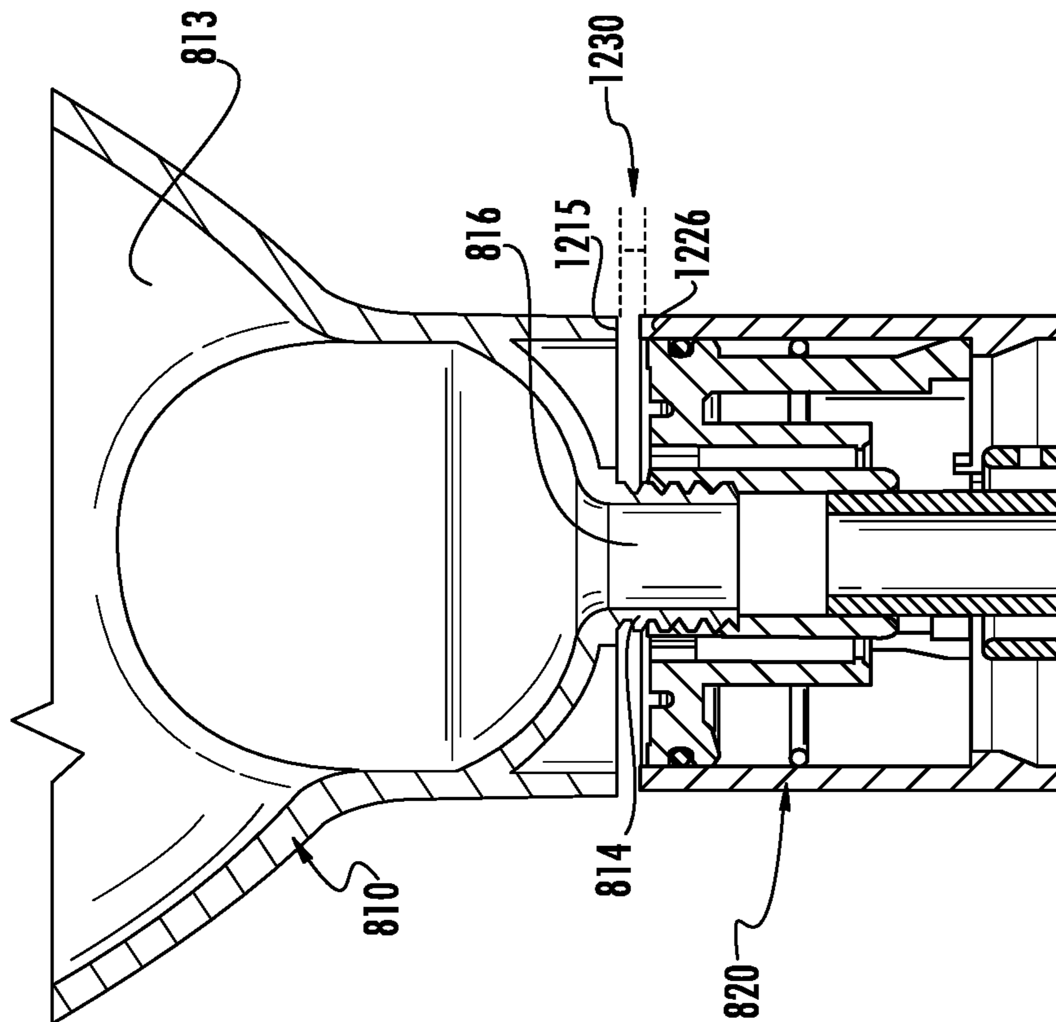
FIG. 12A
