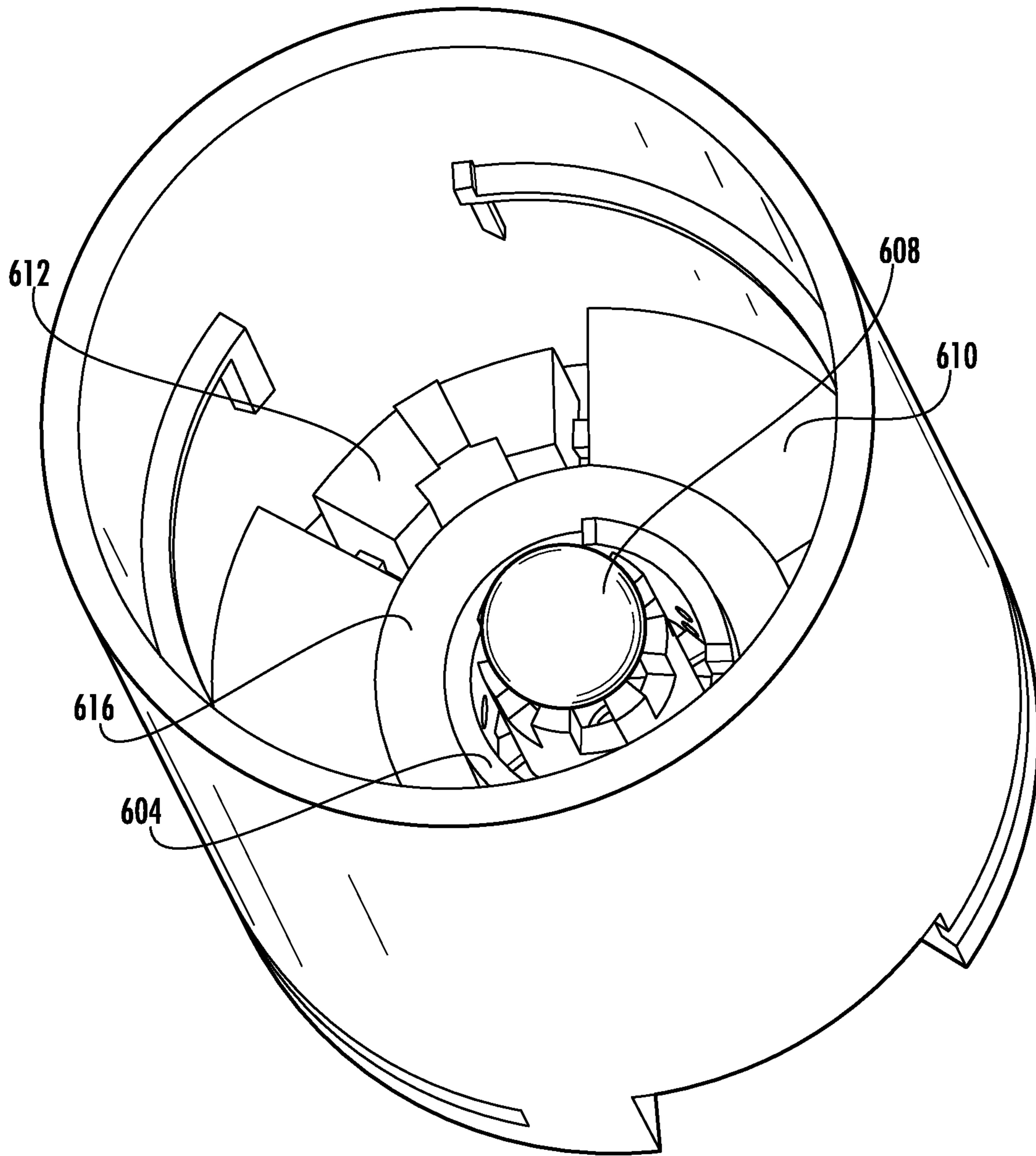
FIG. 6C
