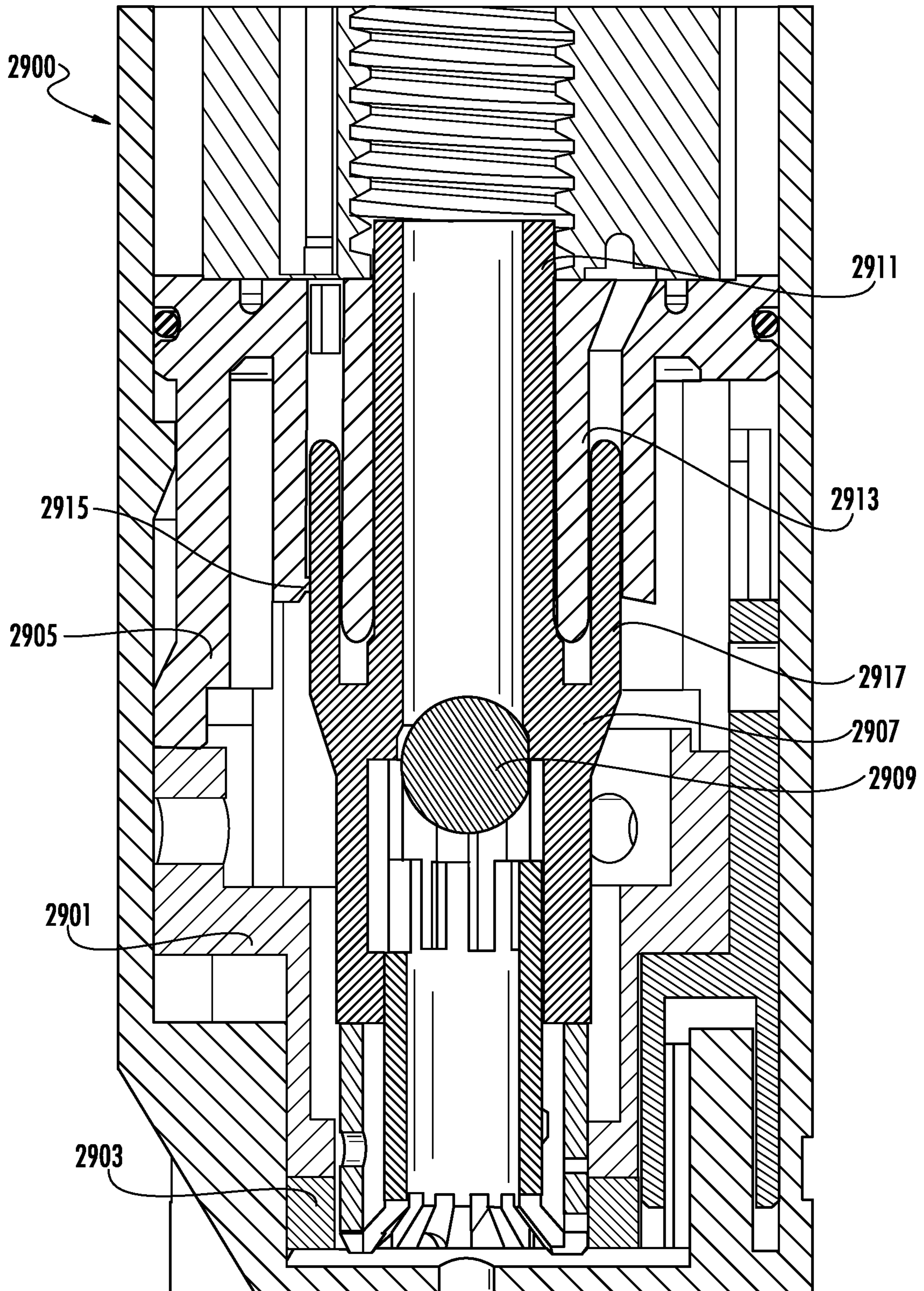
FIG. 29A
