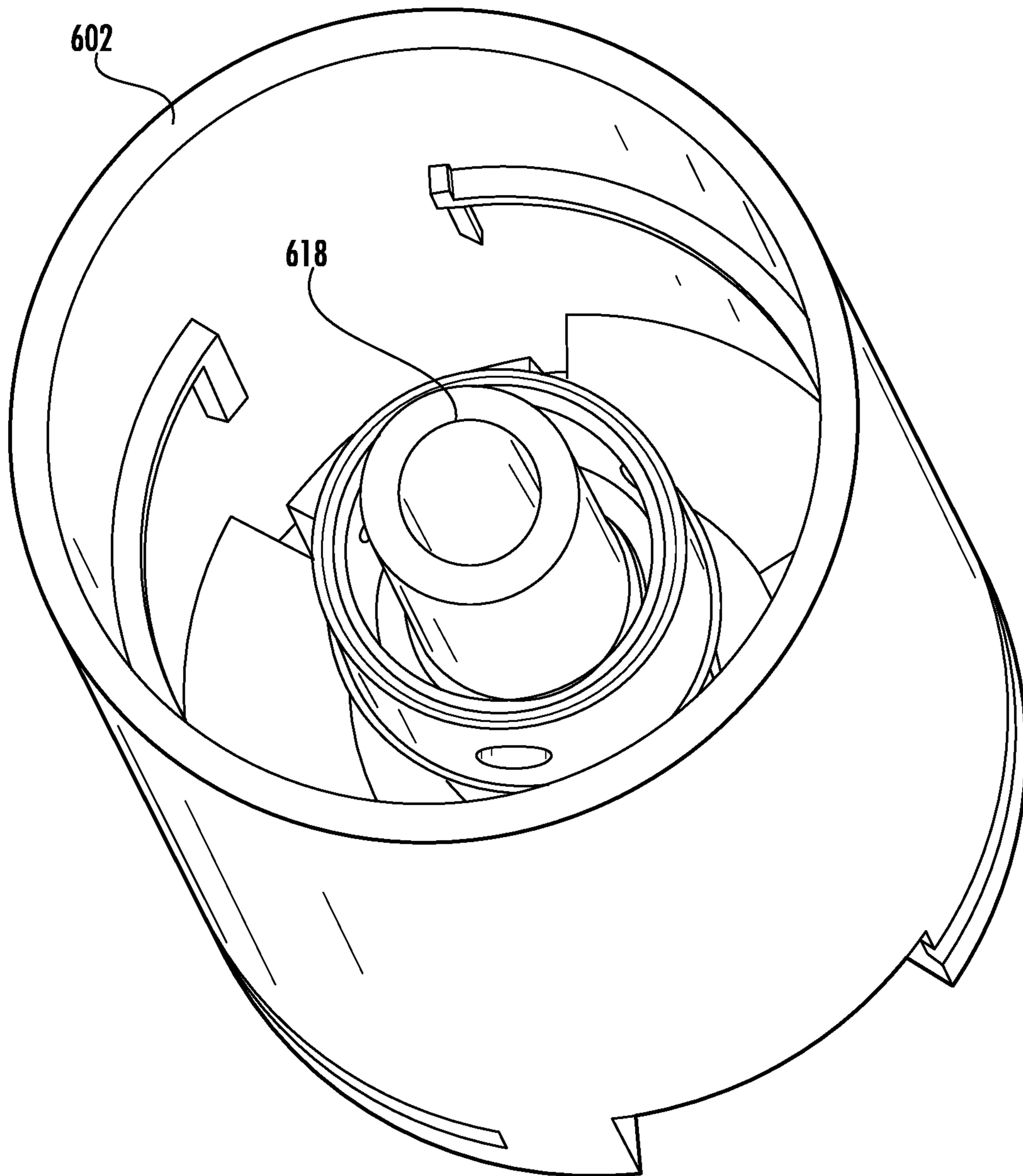
FIG. 6E
