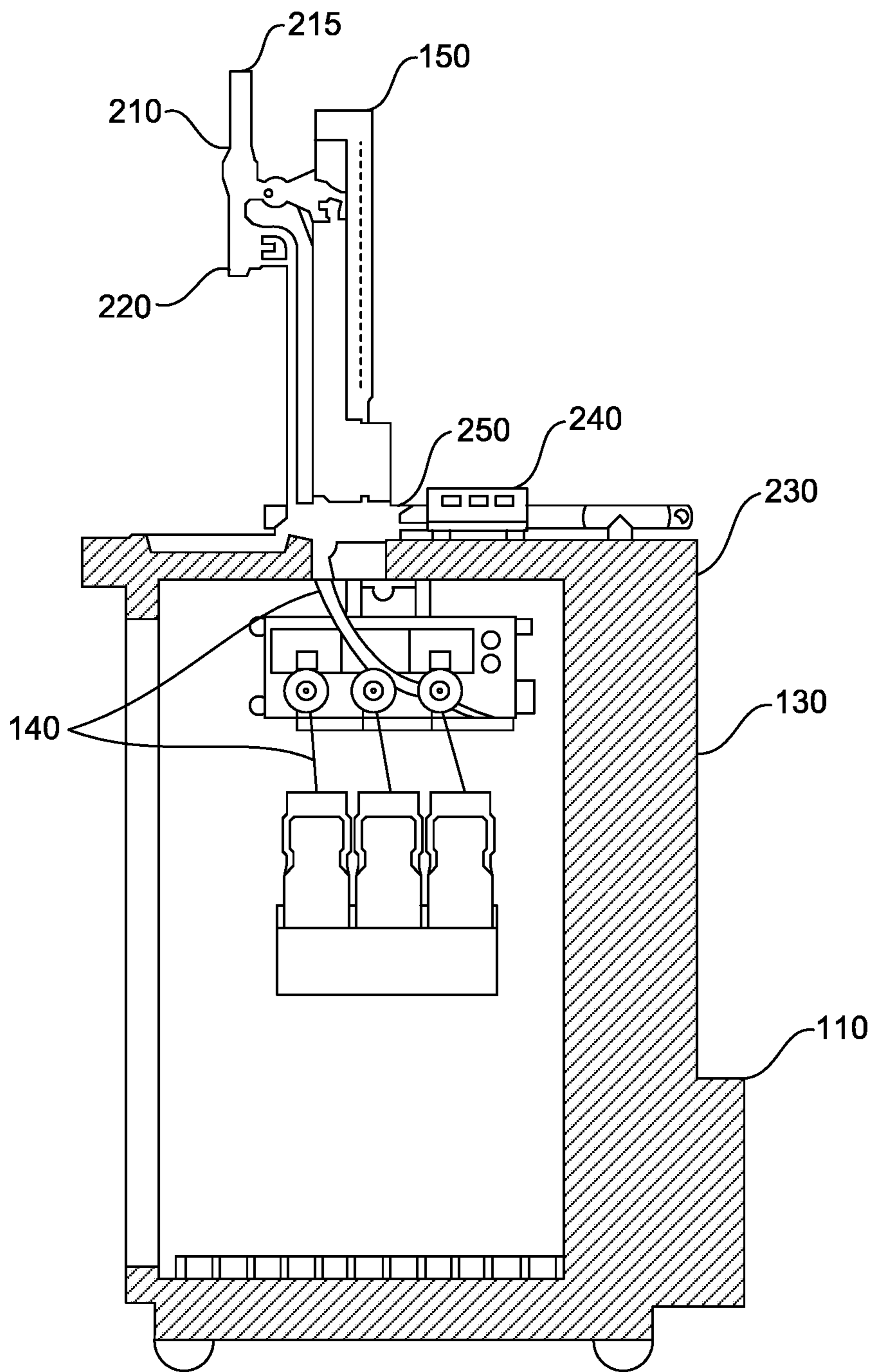
SECTION A-A
