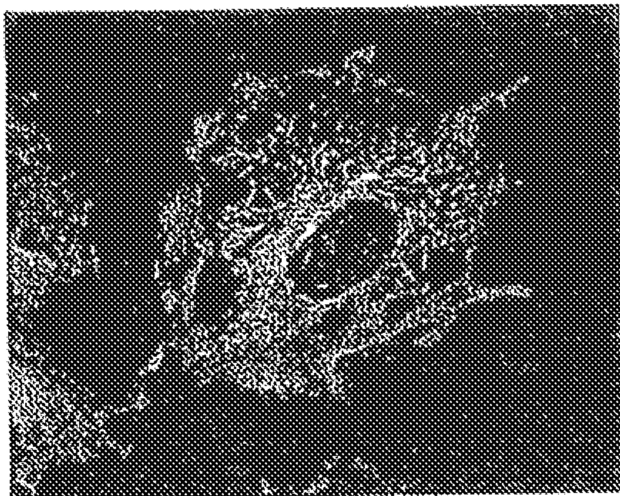
AAG 7 500nM
