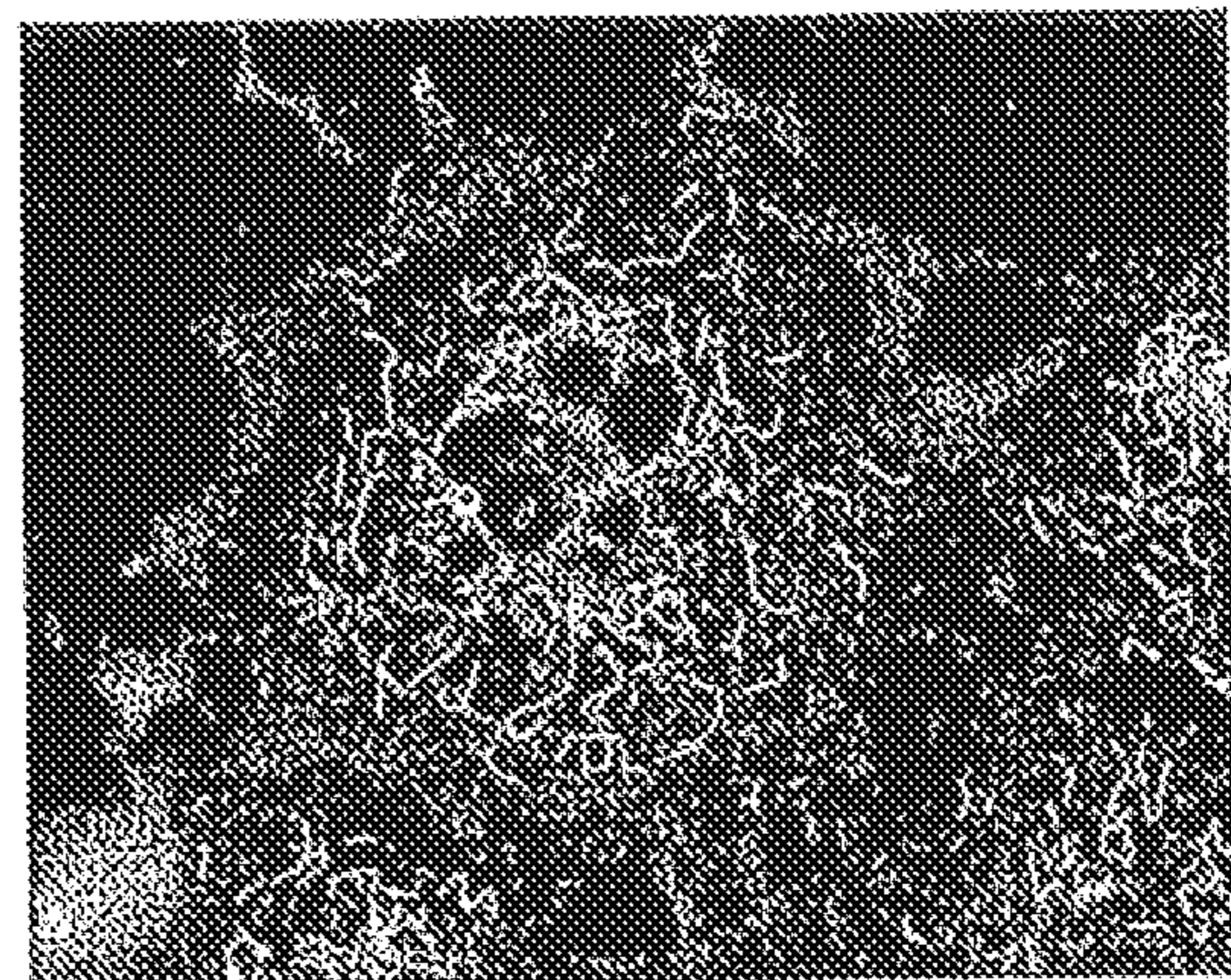
AAG 16 40nM
