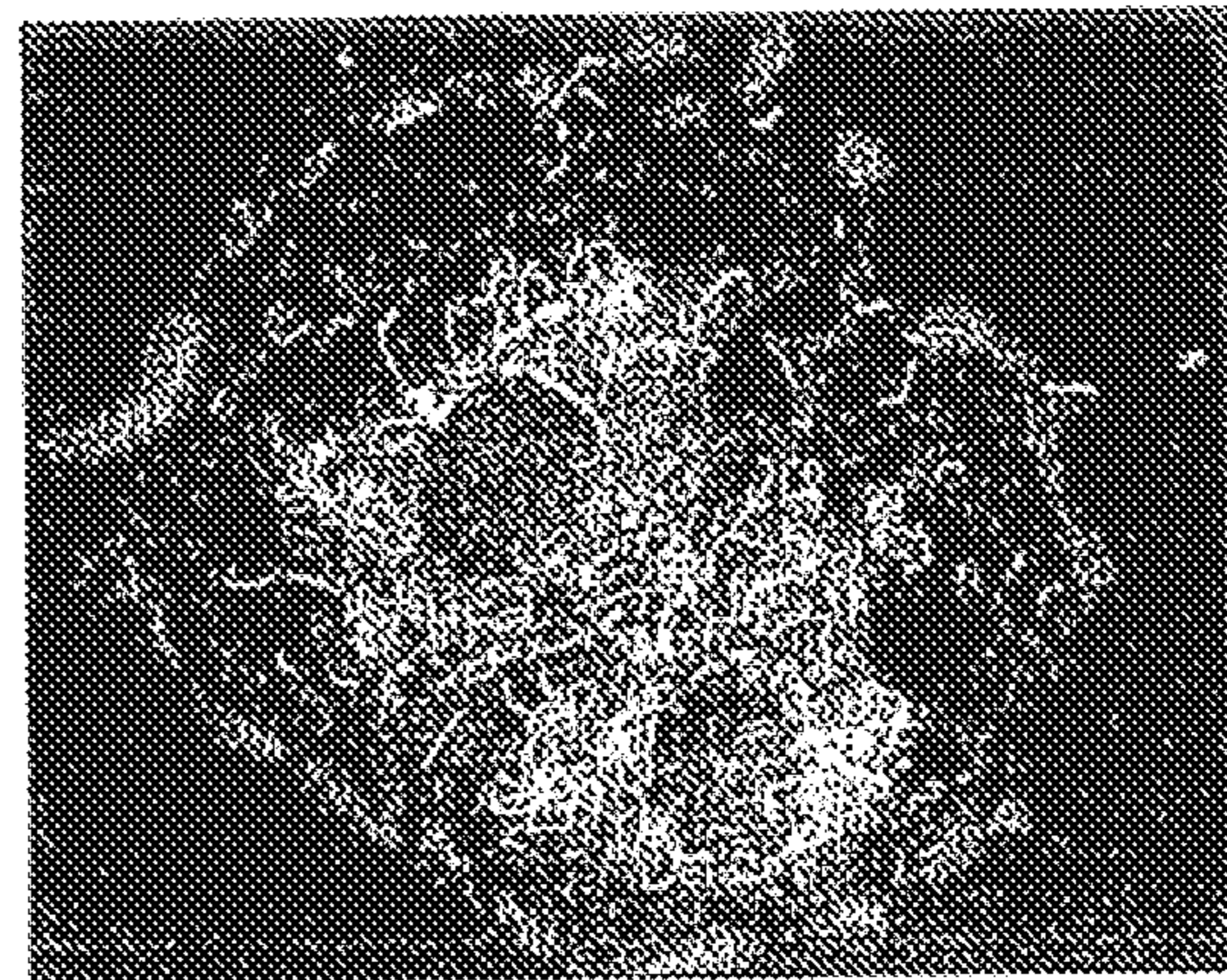
AAG 1 250nM
