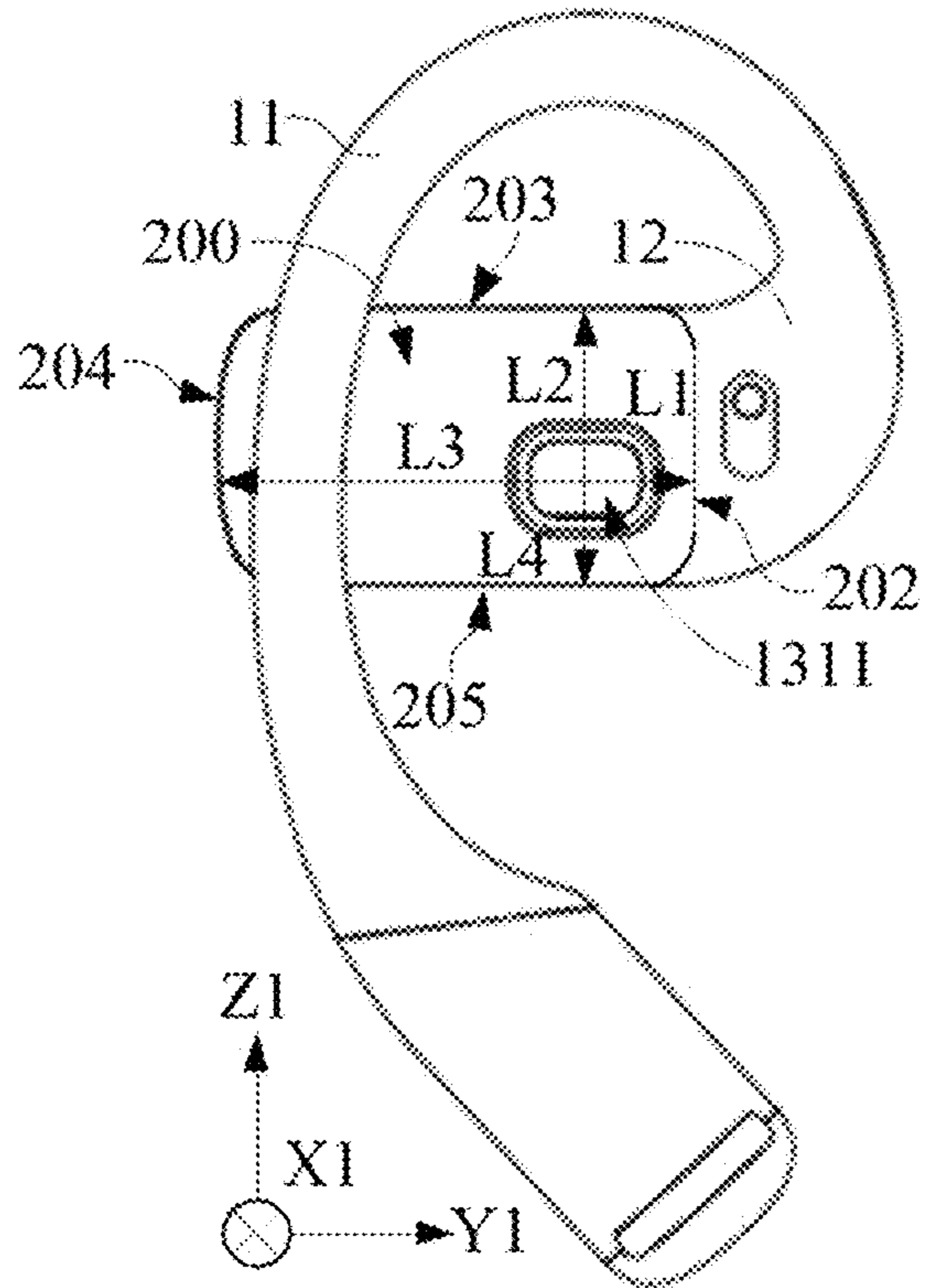
FIG. 54
