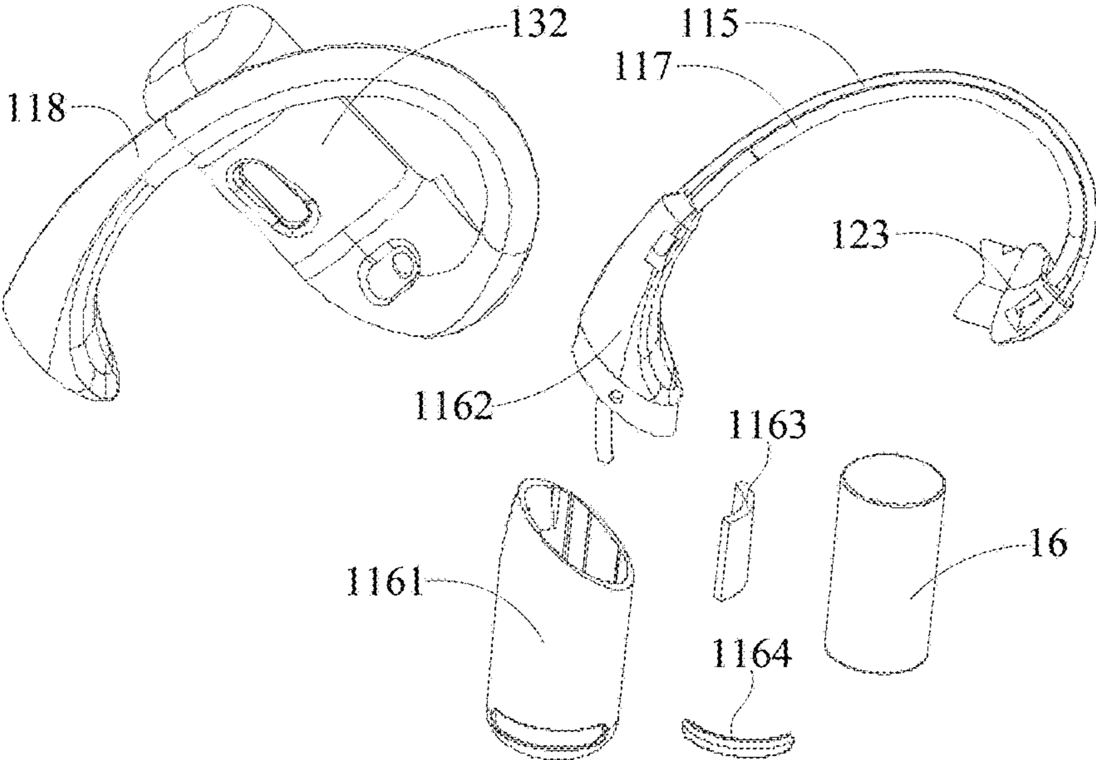
FIG. 33
