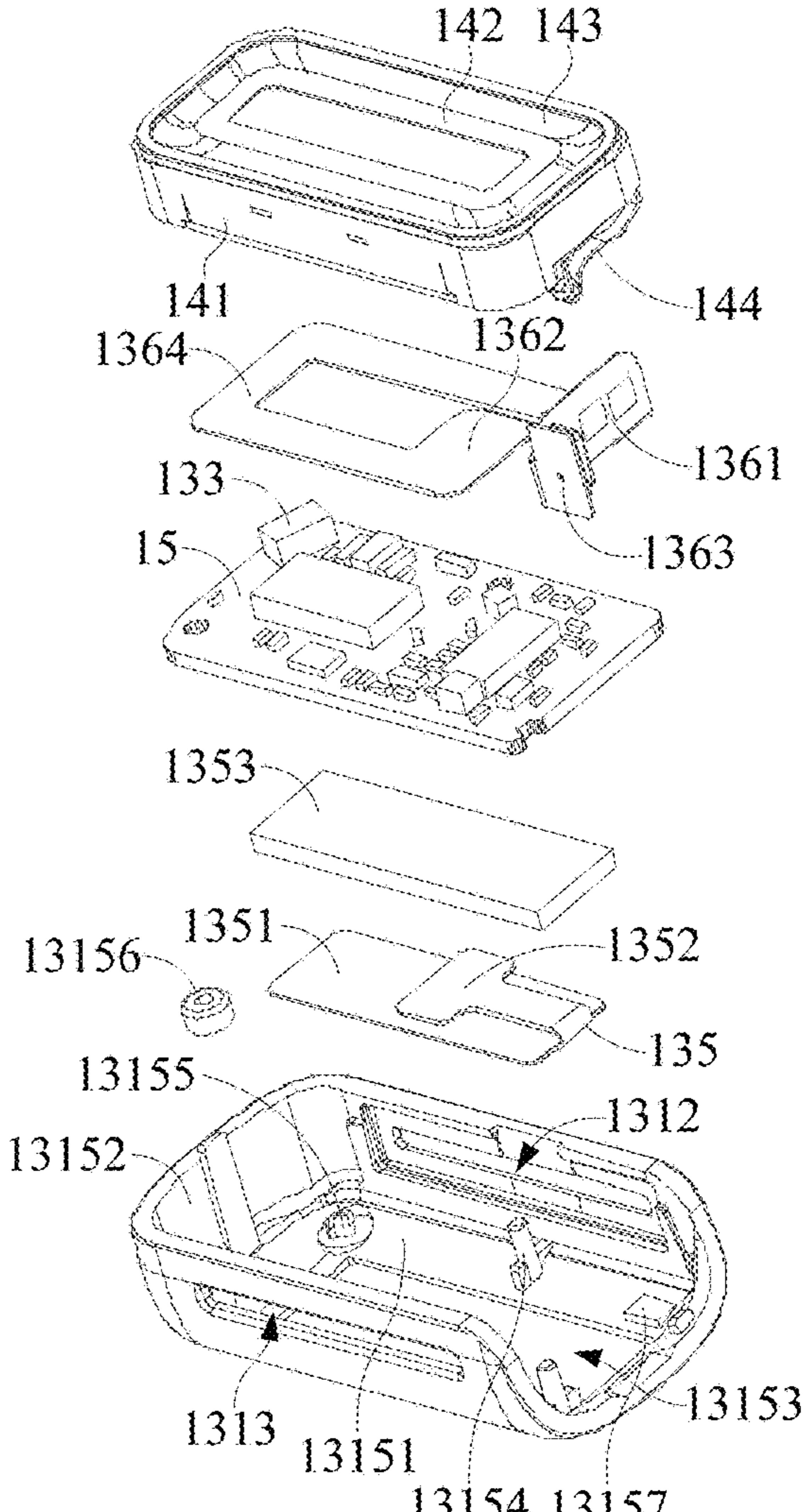
FIG. 35
