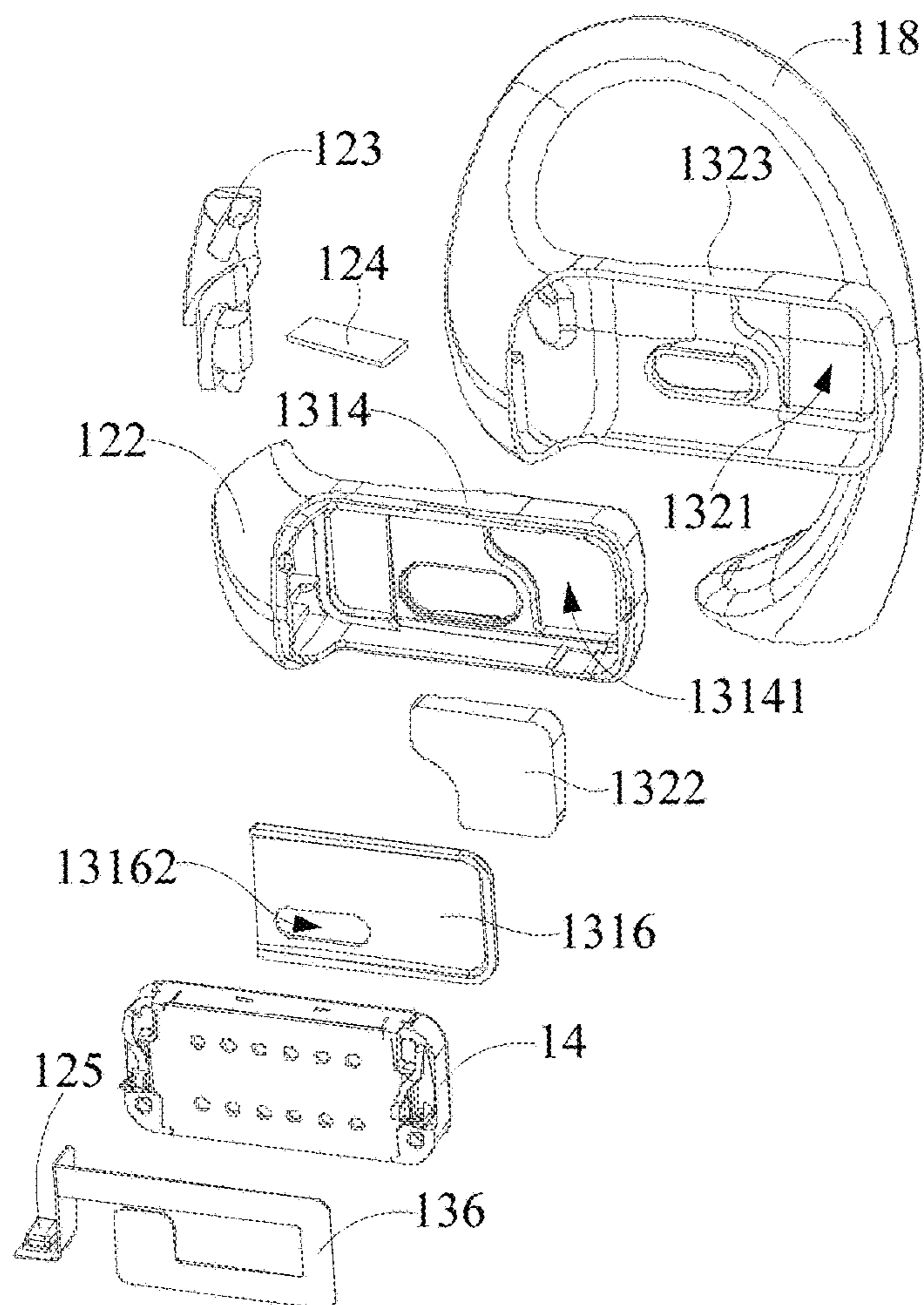
FIG. 41
