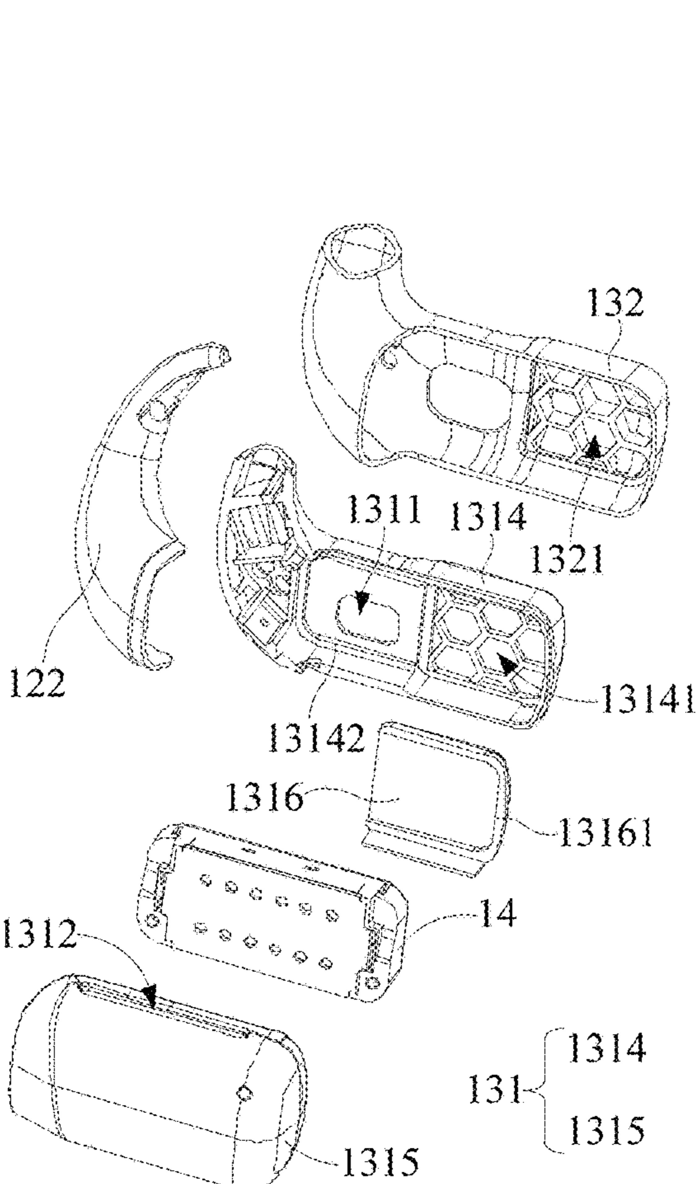
FIG. 34
