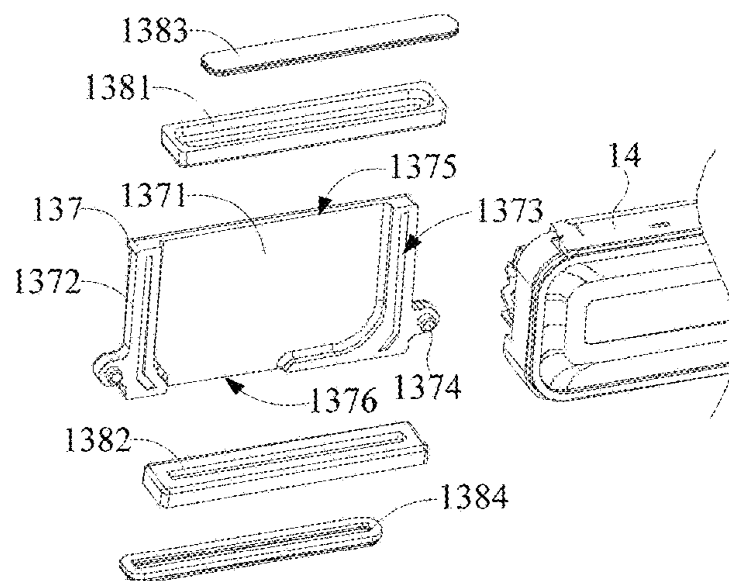
FIG. 44
