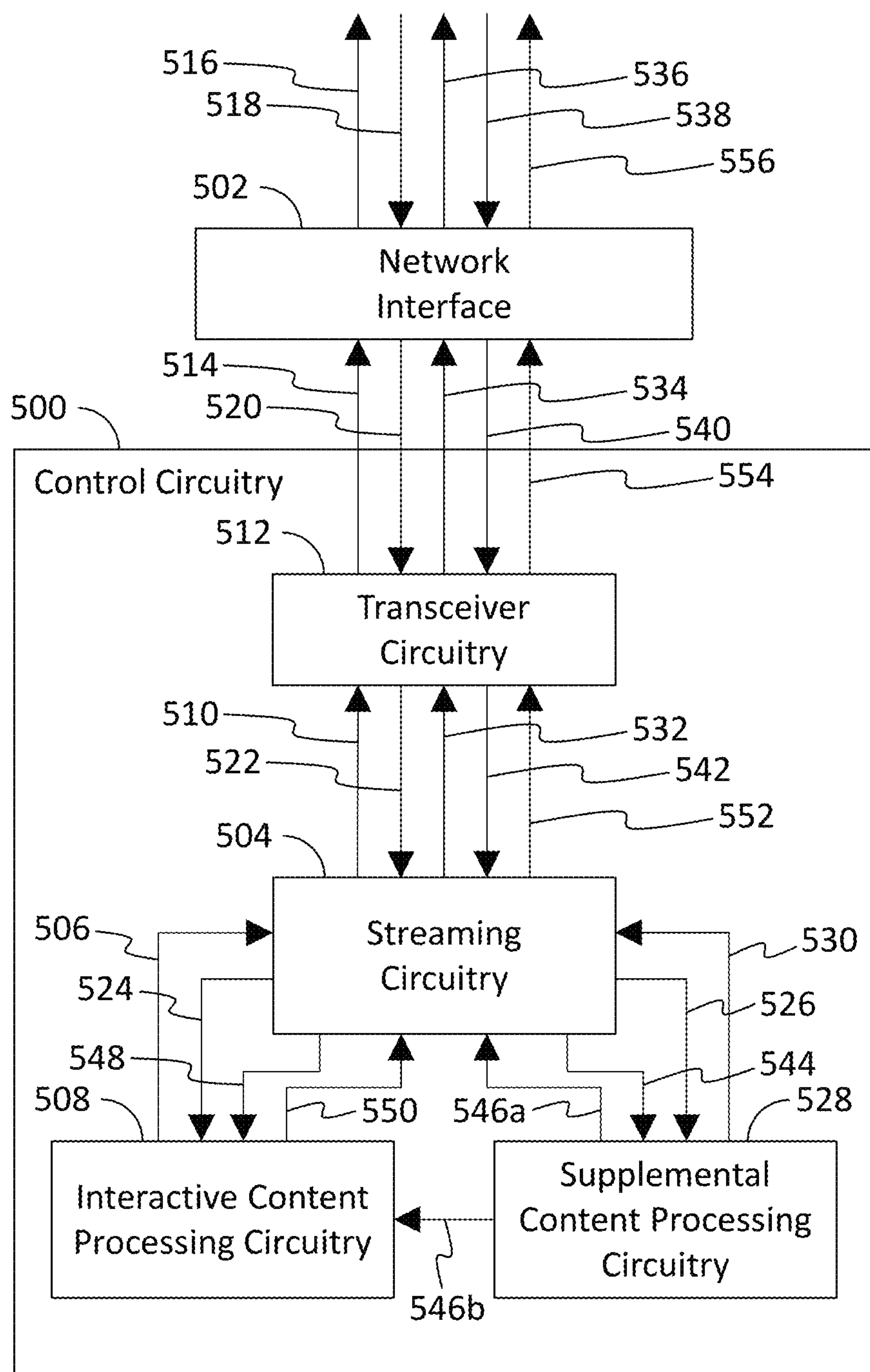
FIG. 5
