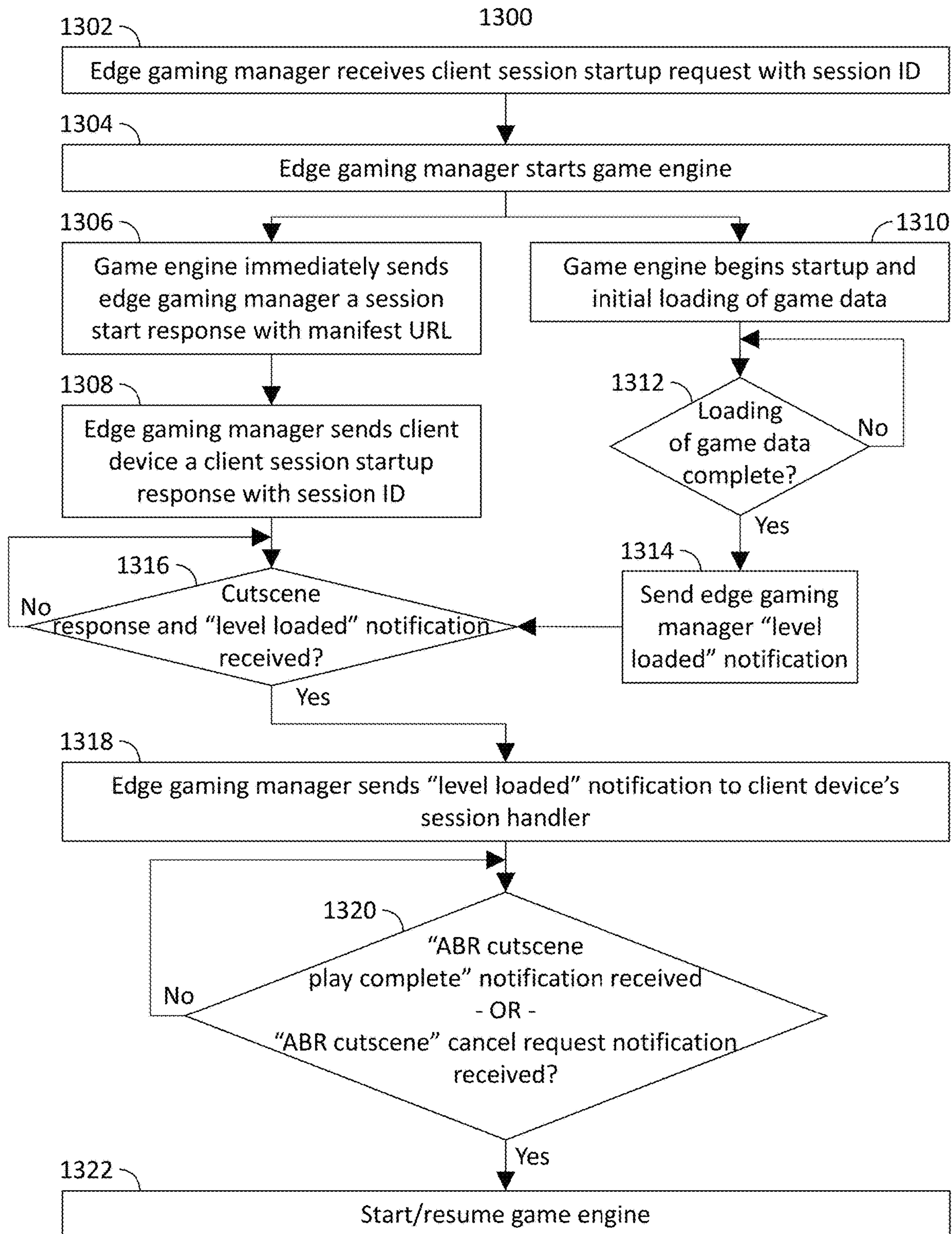
FIG. 13
