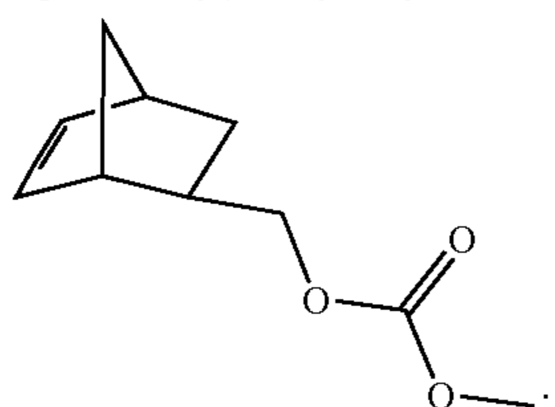
(bicyclo[2.2.1]hept-5-en-2-yl)methyl methyl carbonate (NBMeCarb)
