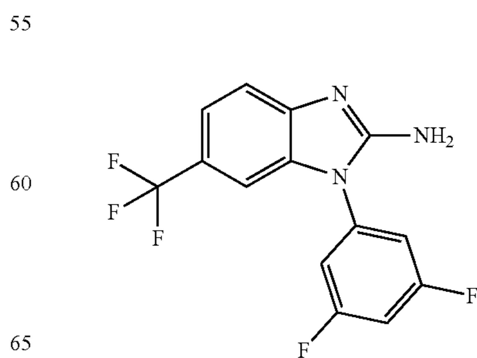
1-(3,5-difluorophenyl)-6-(trifluoromethyl)-1H-benzo[d]imidazol-2-amine
