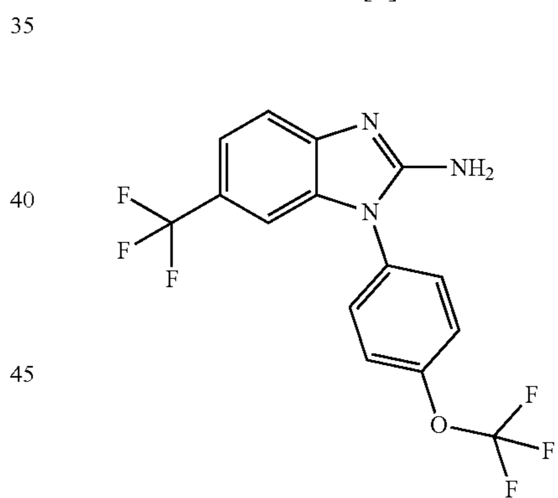
1-(4-(trifluoromethoxy)phenyl)-6-(trifluoromethyl)-1H-benzo[d]imidazol-2-amine
