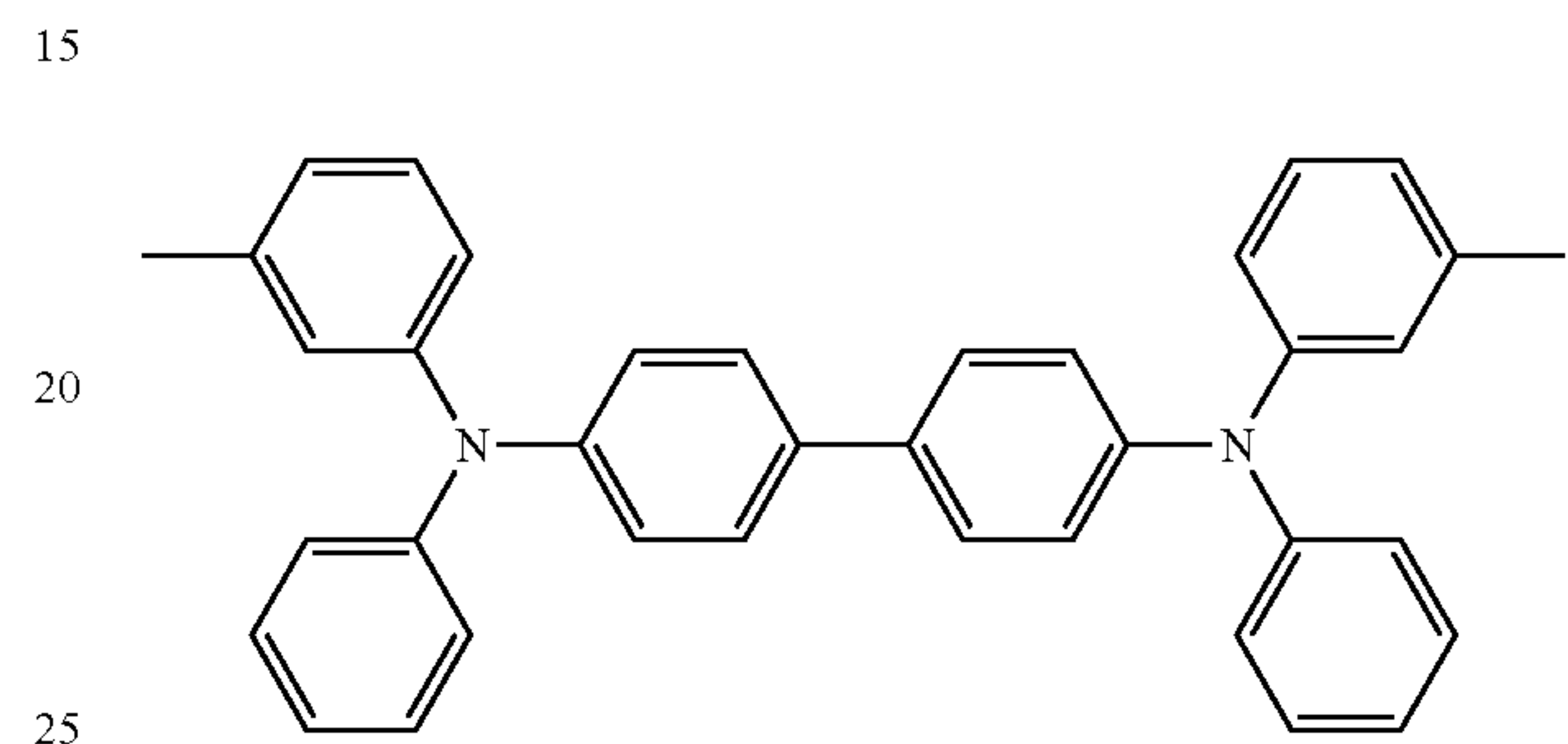
TPD
