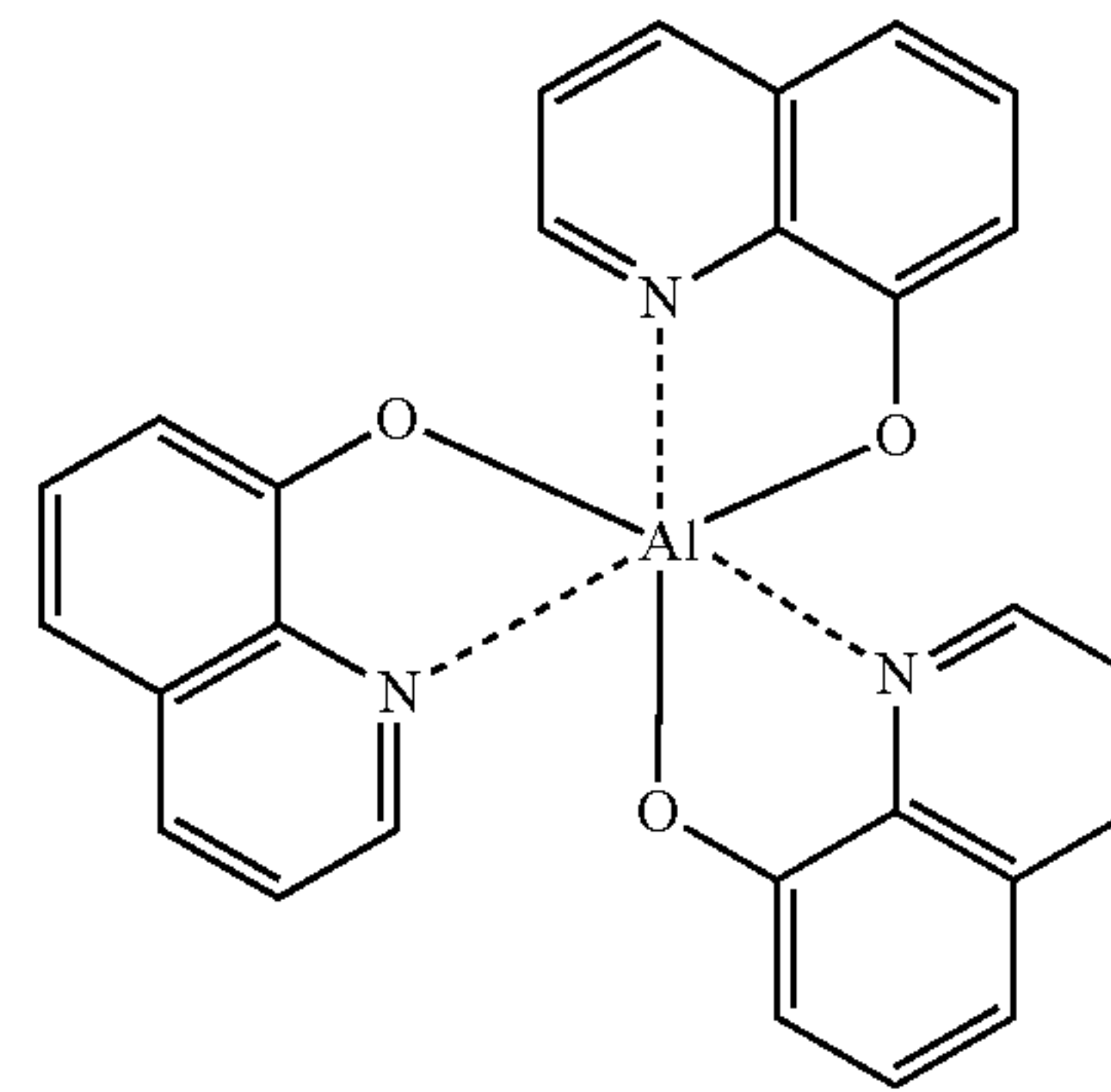
Alq 3
