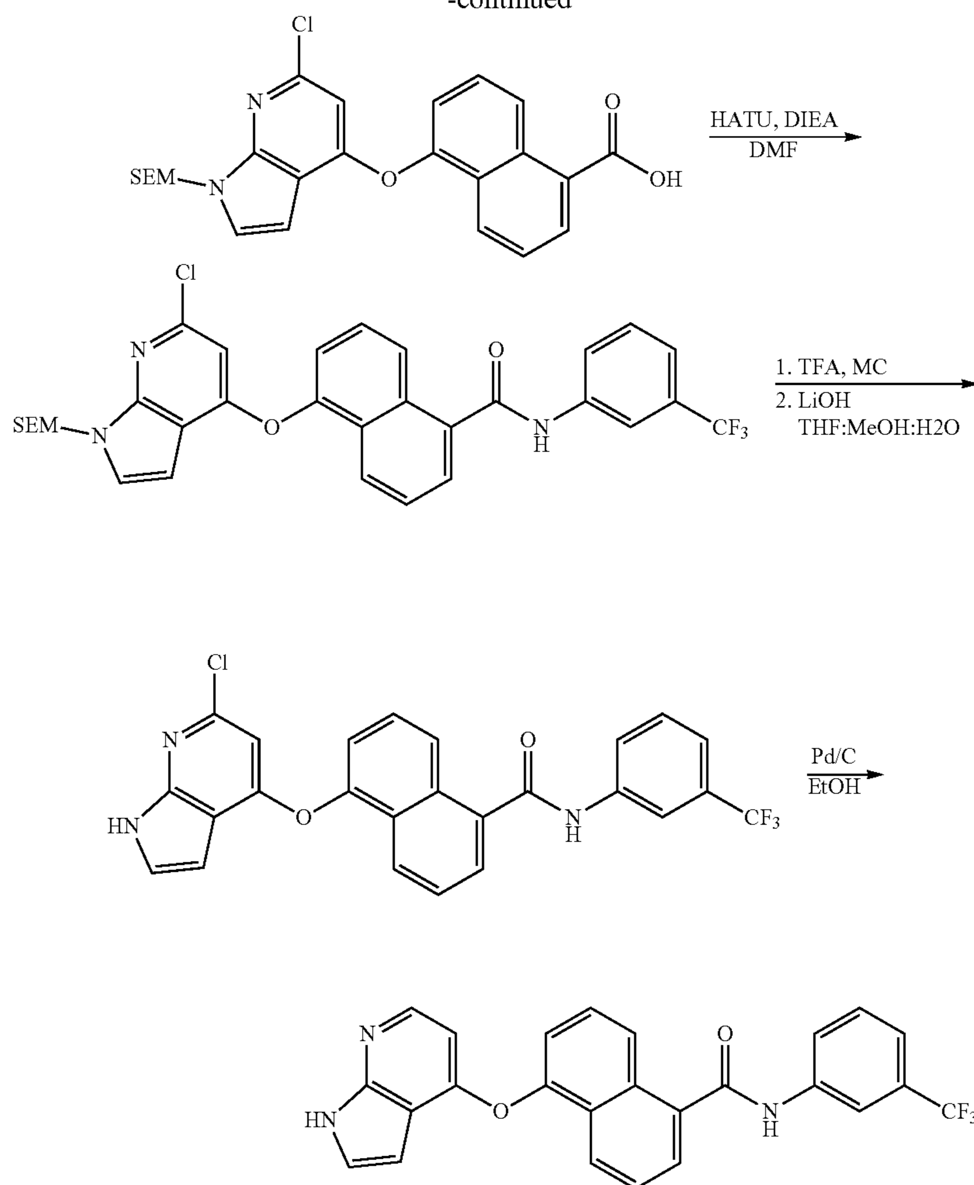
A. 5-(6-chloro-1-((2-(trimethylsilyl)ethoxy)methyl)-1H-pyrrolo[2,3-b]pyridin-4-yloxy)-1-naphthoic Acid
