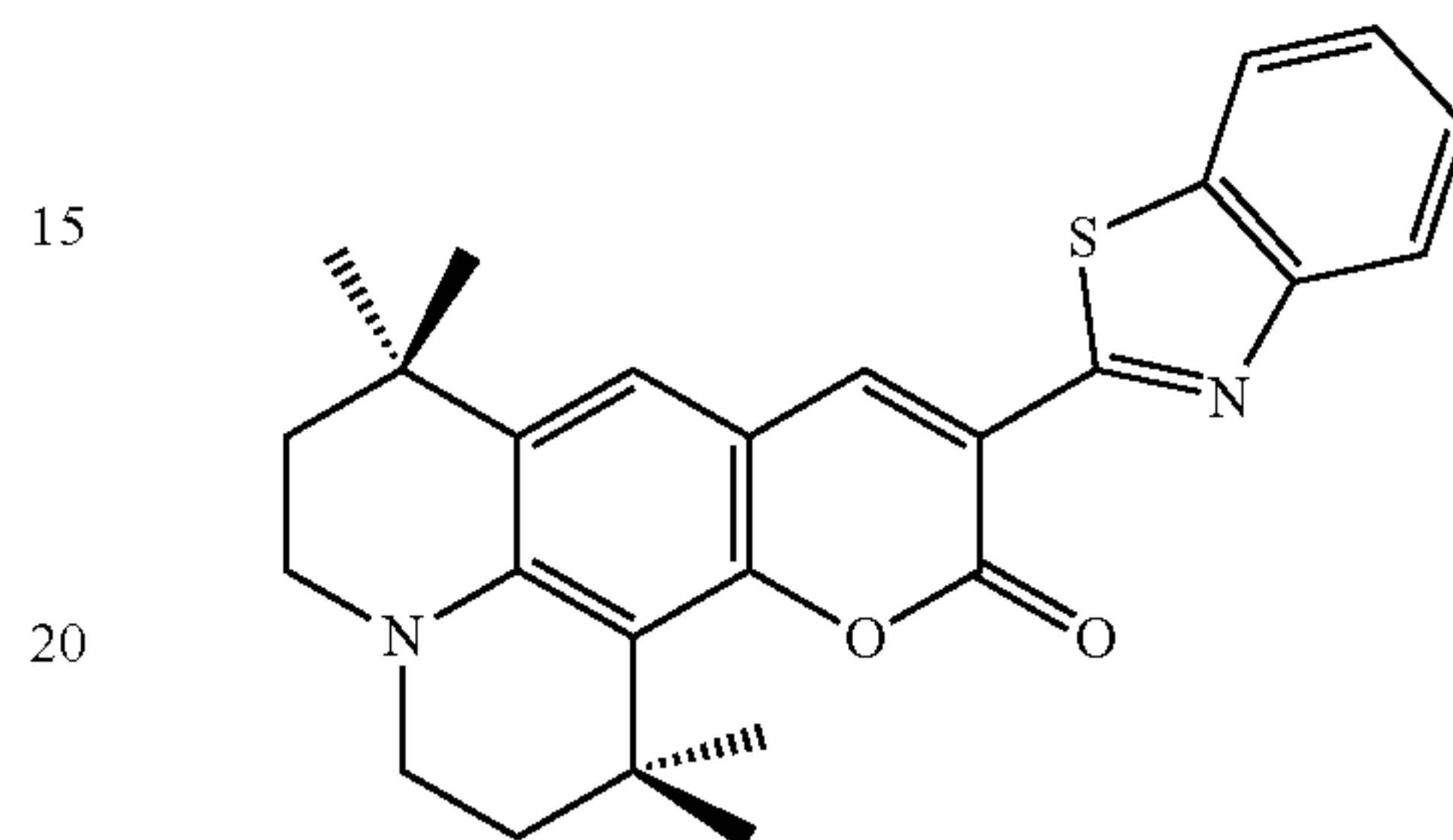
C545T
