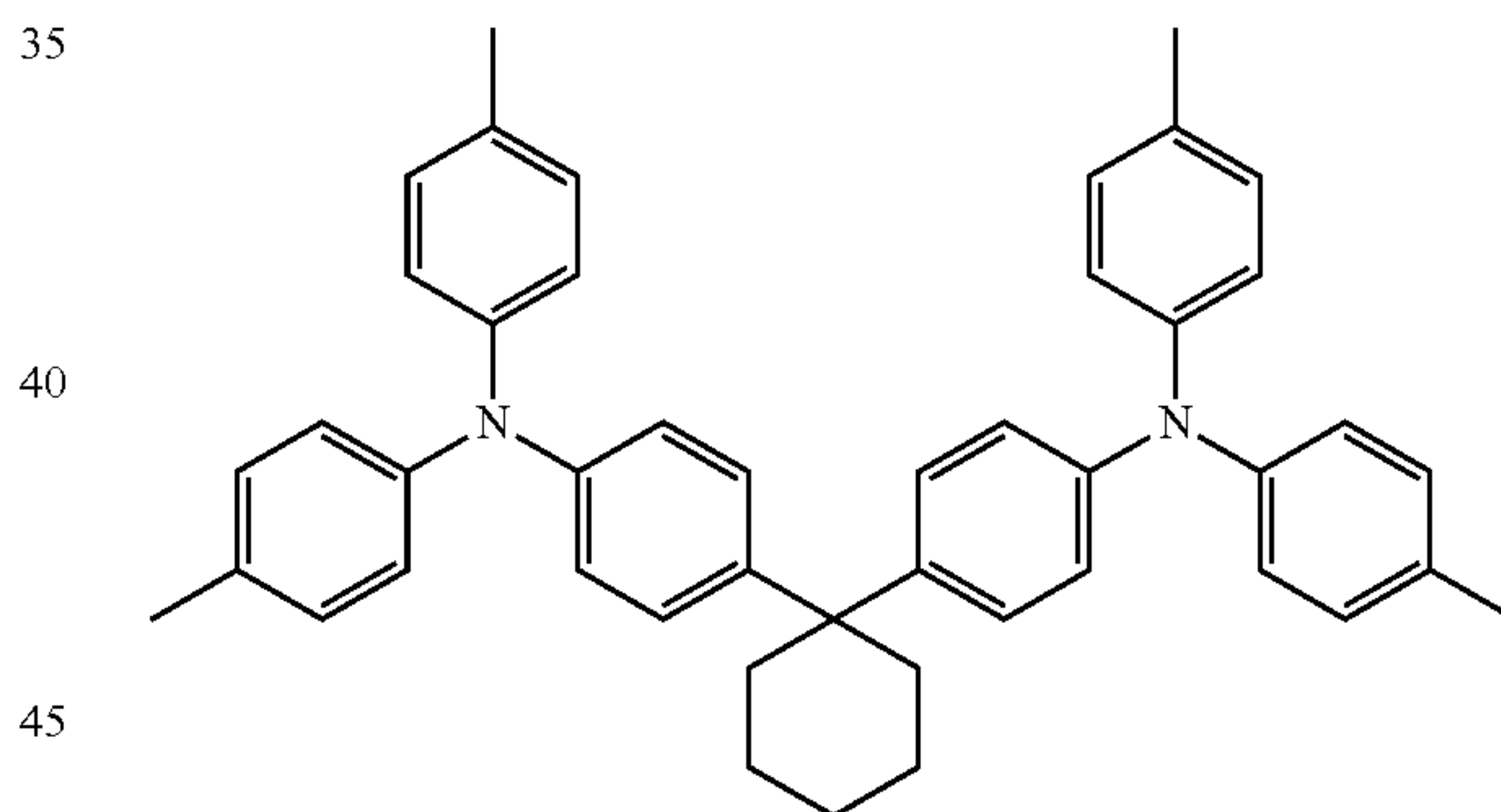
TAPC
