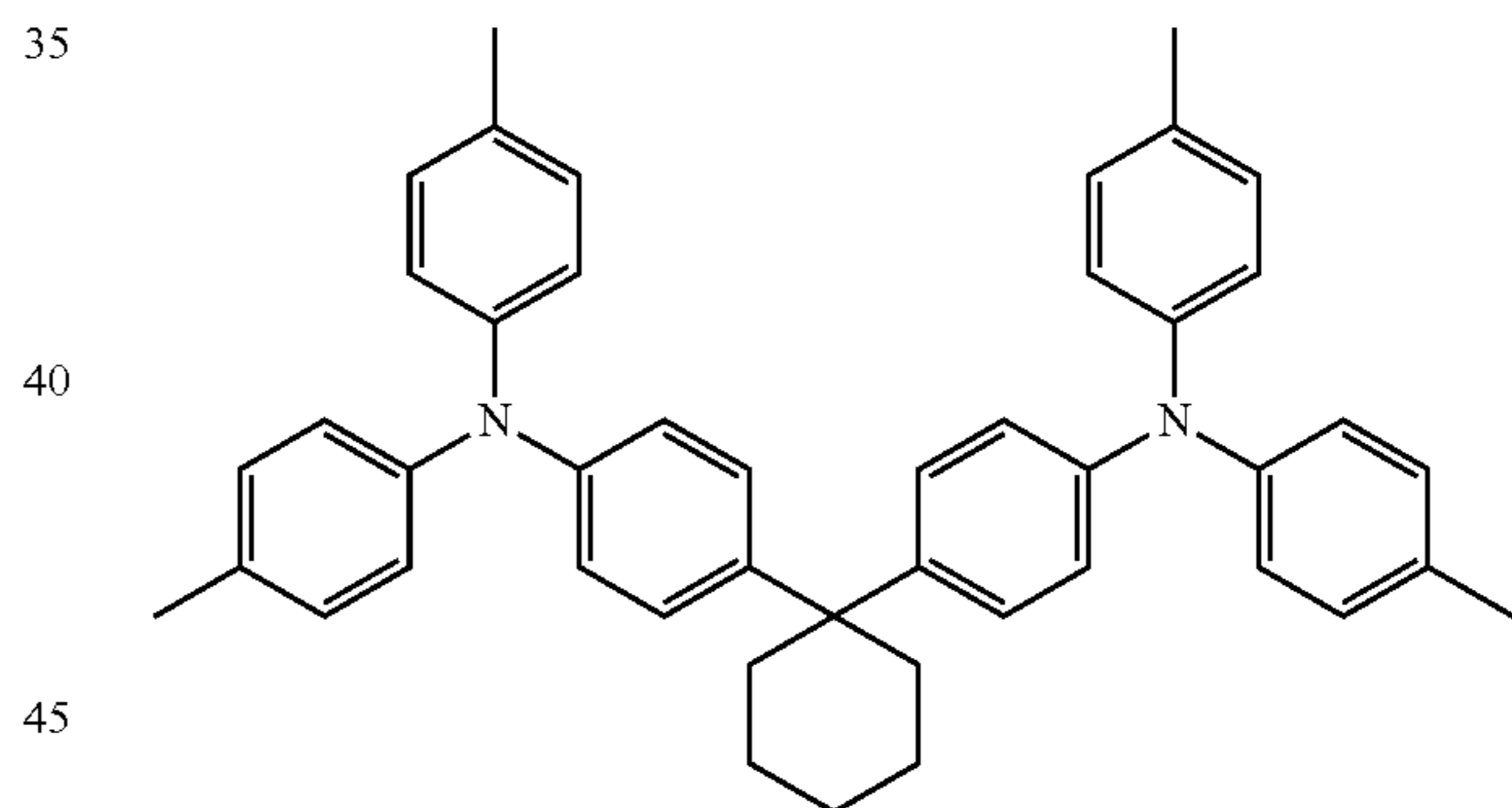
TAPC
