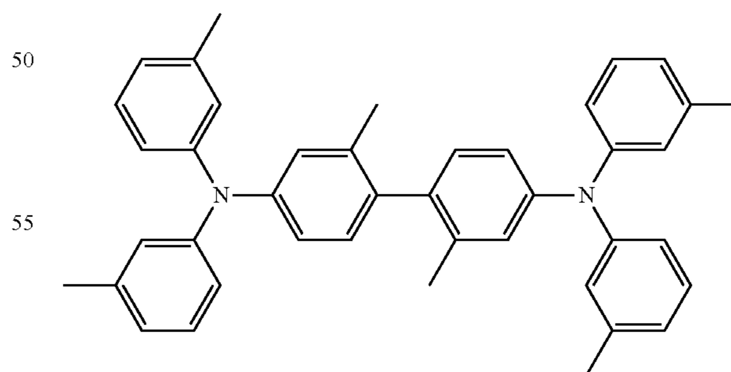
HMTPD
