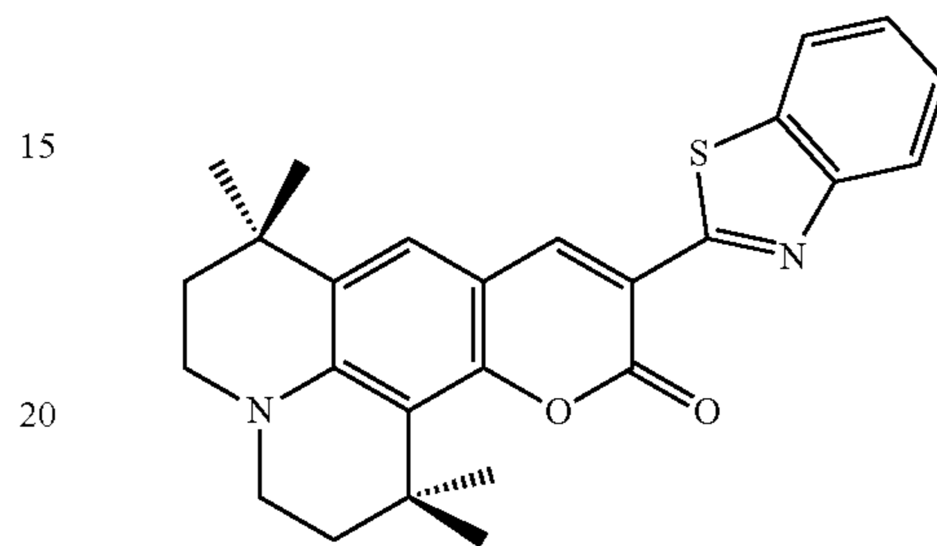
C545T
