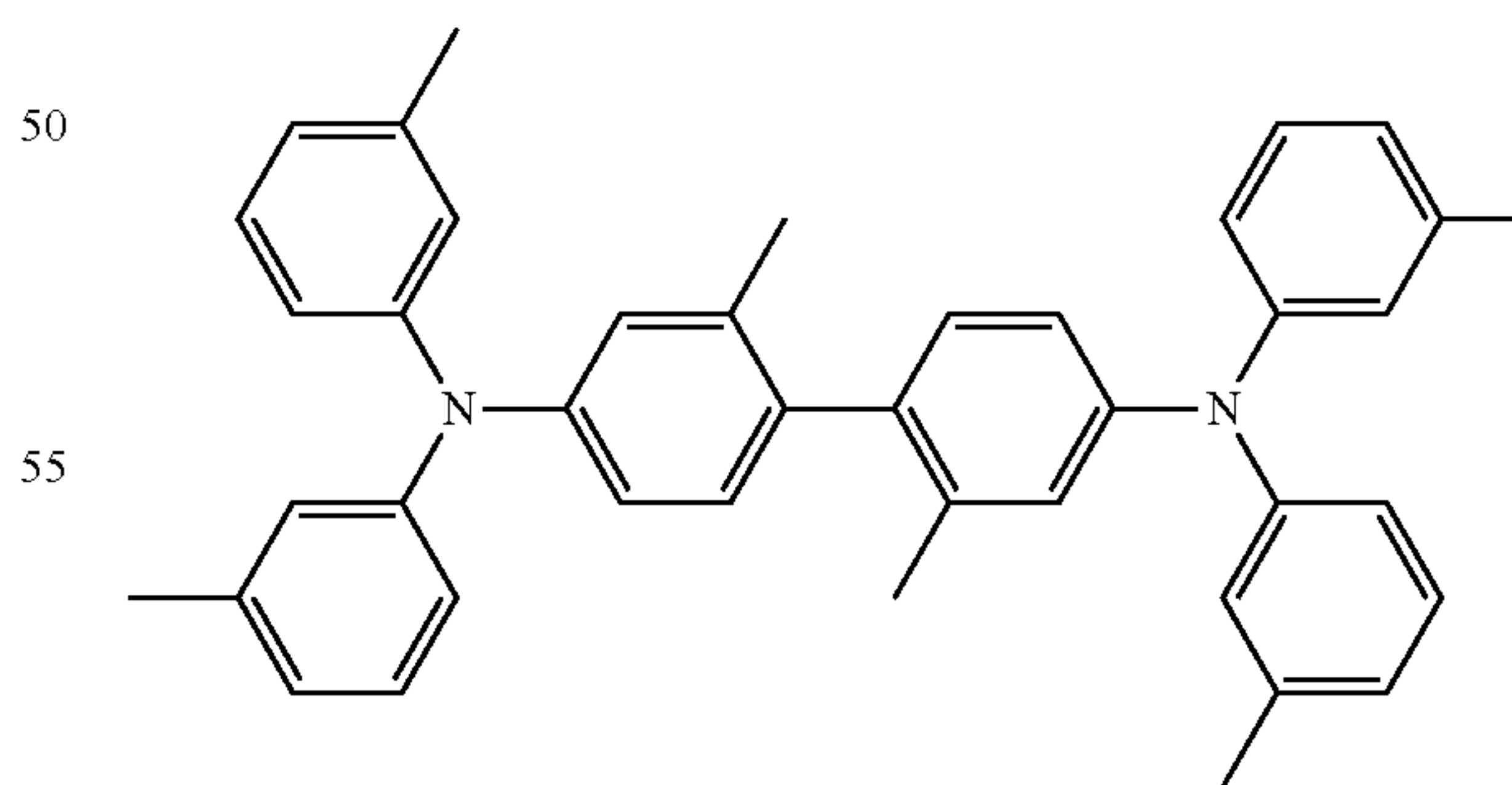
HMTPD
