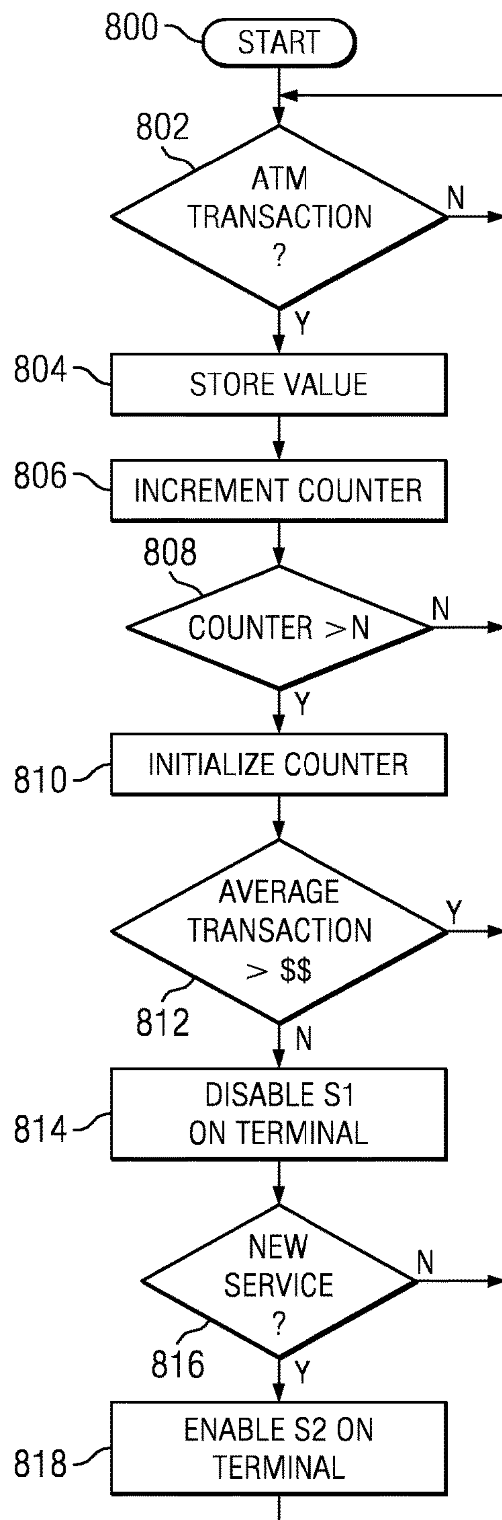
FIG. 8
