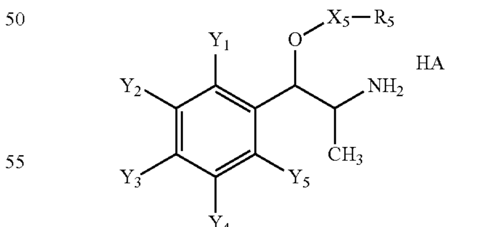
Structure CS-6
