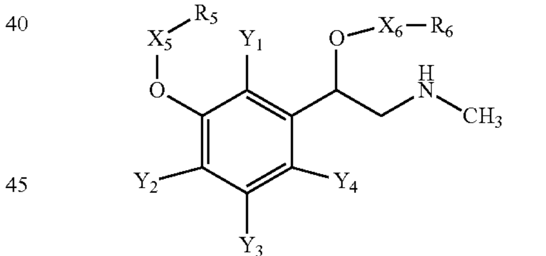
Structure CS-5
