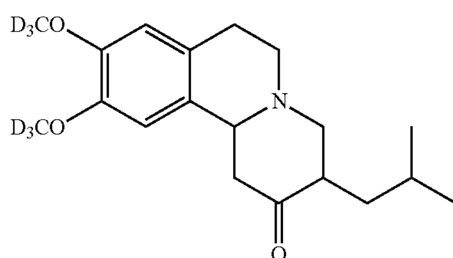
d_6 -Tetrabenazine (Deutetrabenazine)
