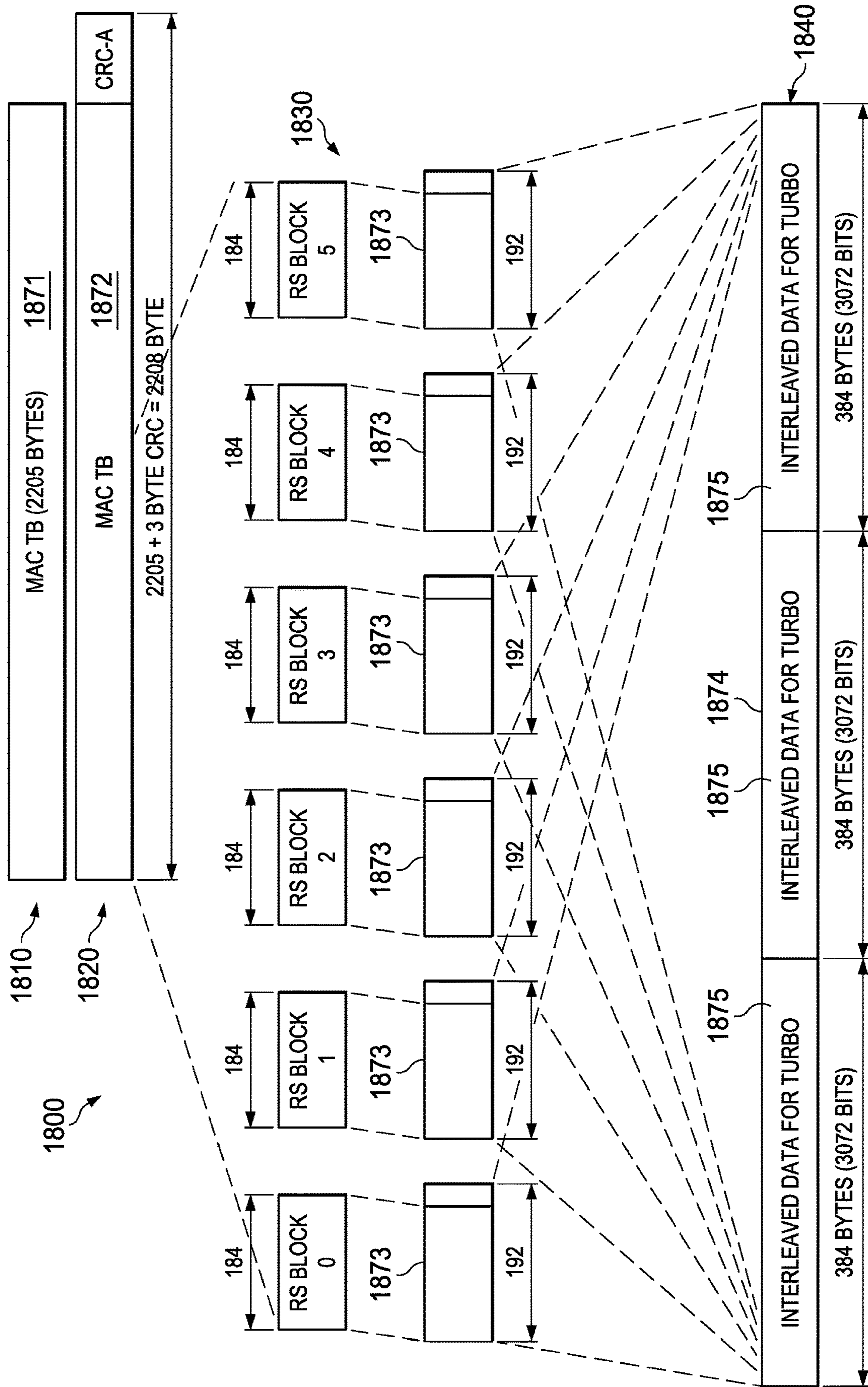
FIG. 18
