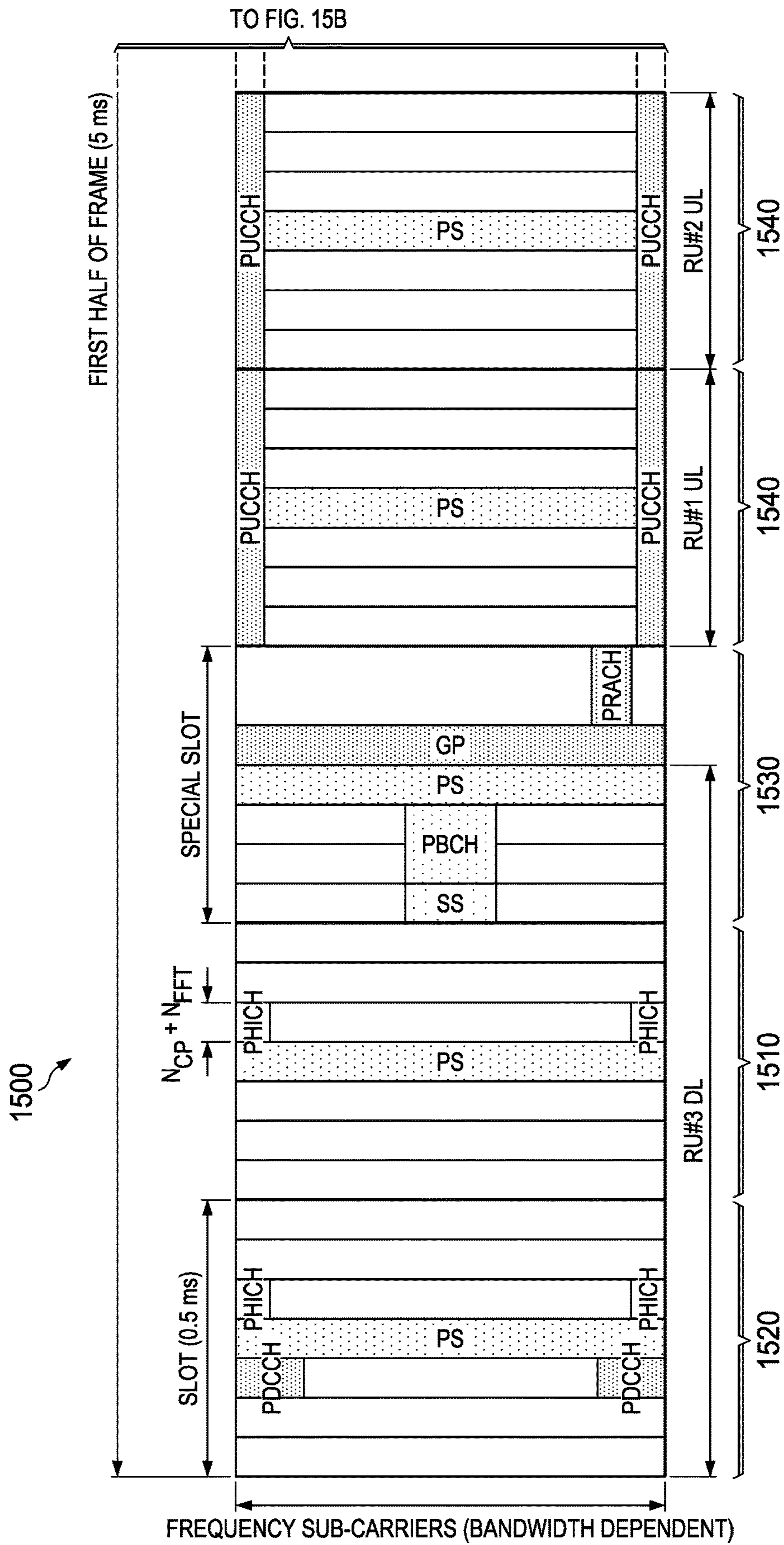
FIG. 15A
