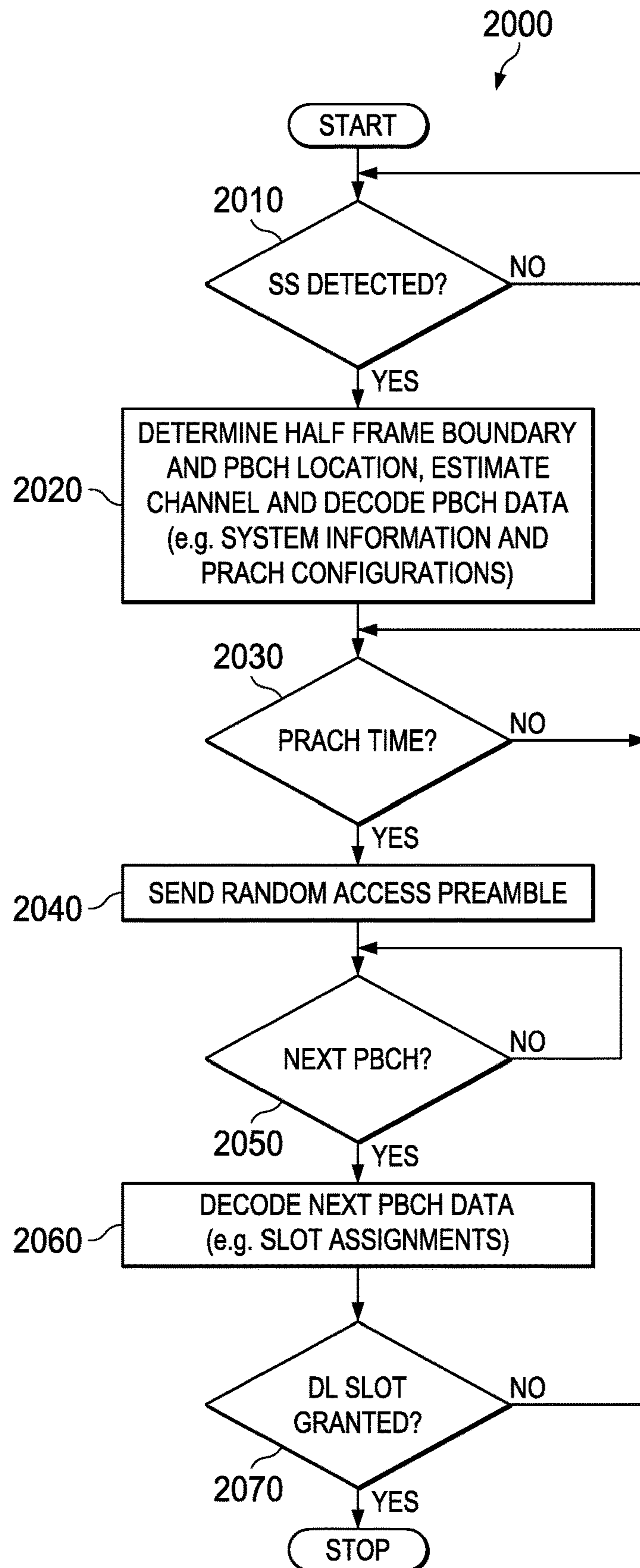
FIG. 20
