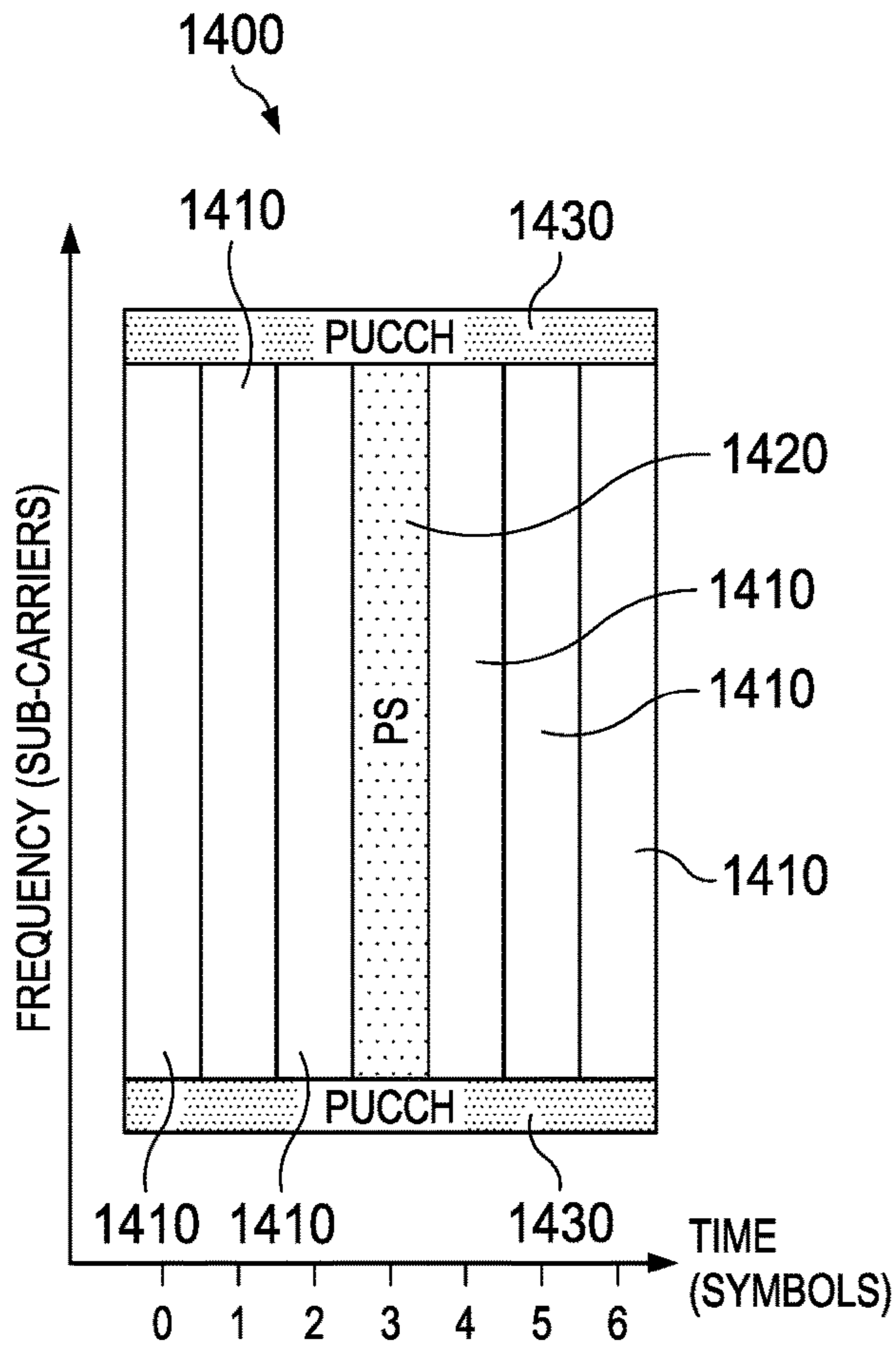
FIG. 14A
