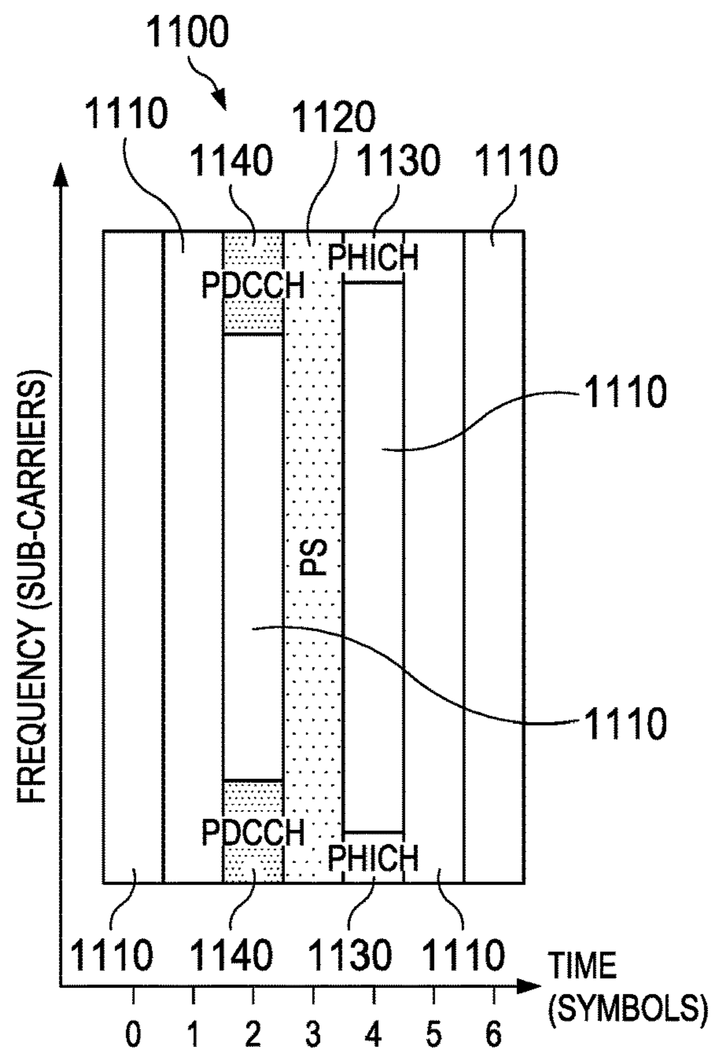
FIG. 11
