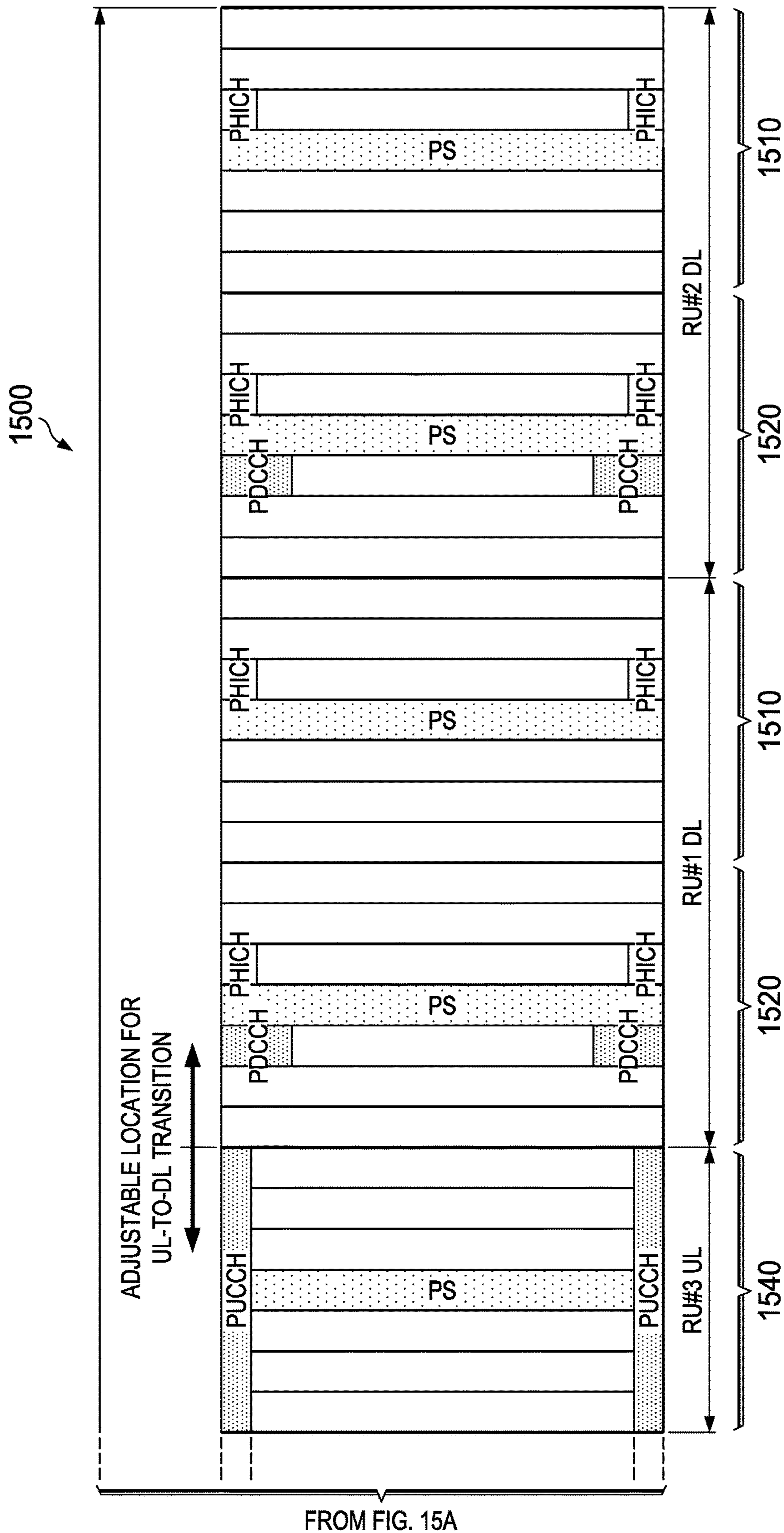
FIG. 15B
