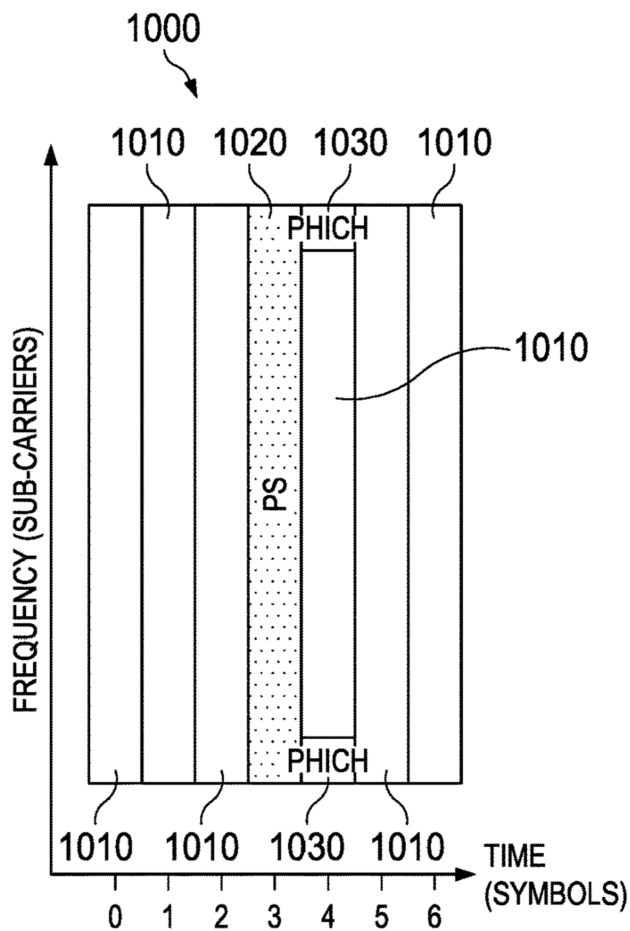
FIG. 10
