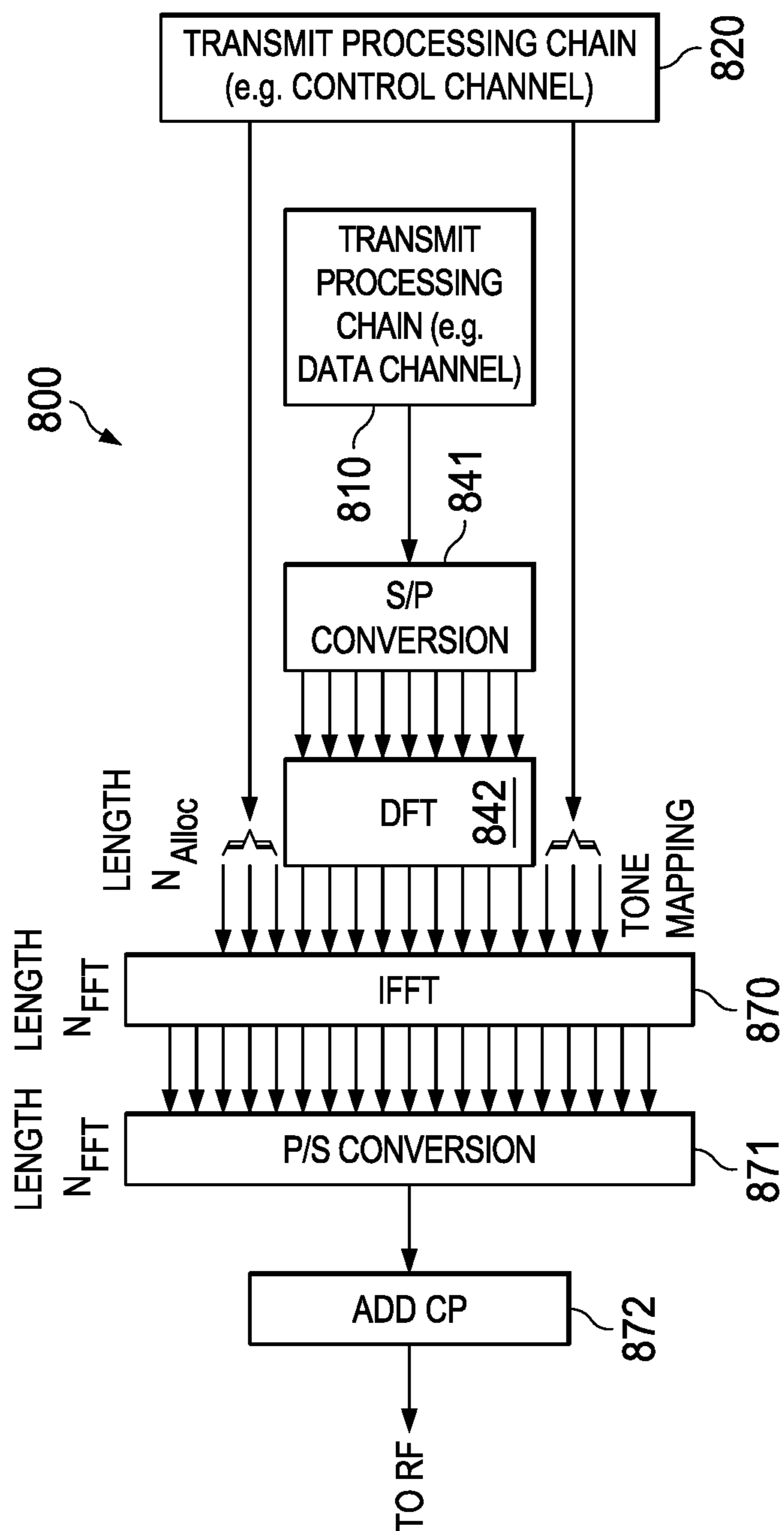
FIG. 8
