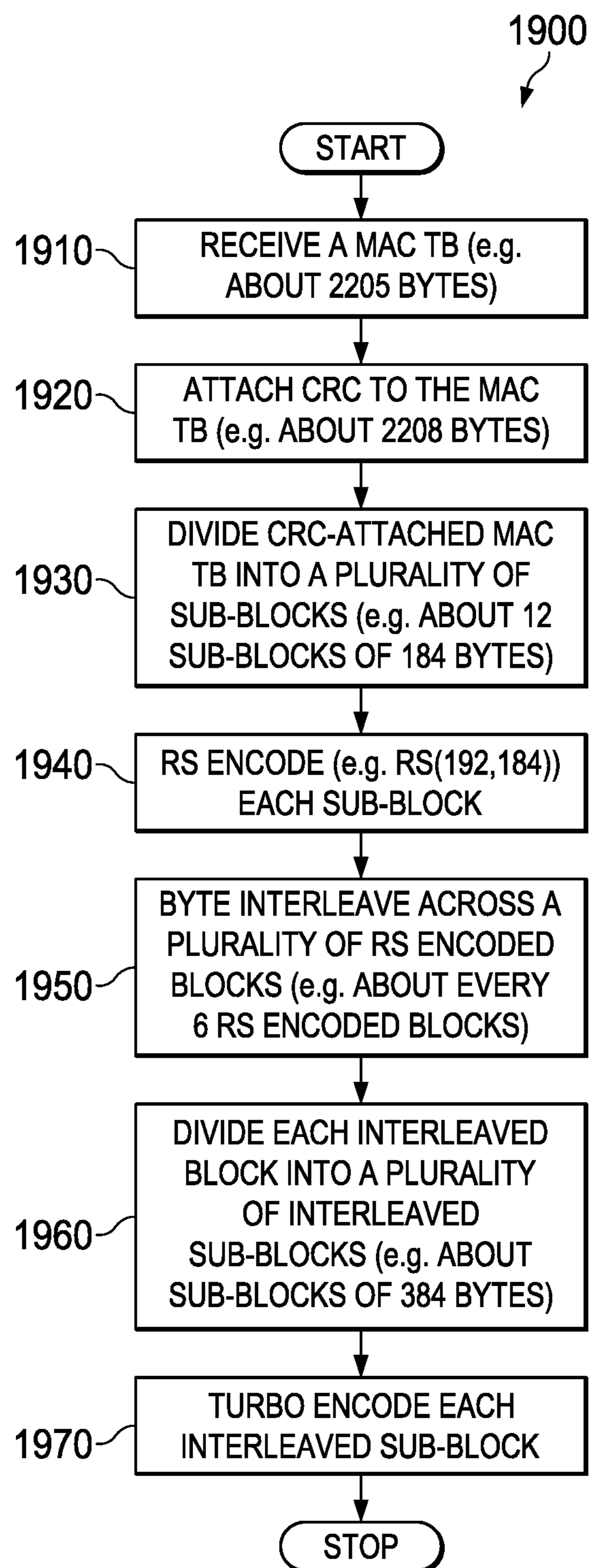
FIG. 19
