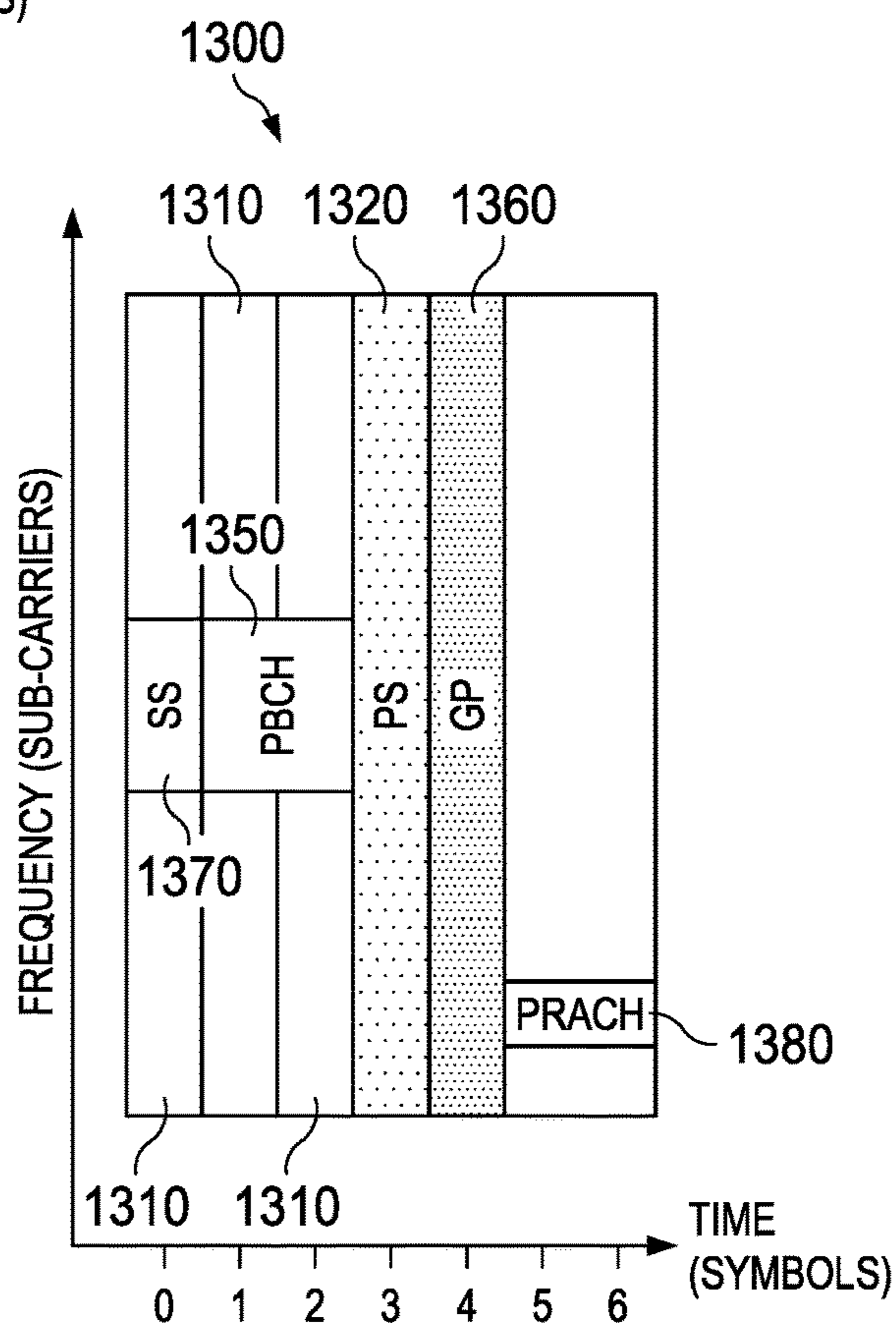
FIG. 13
