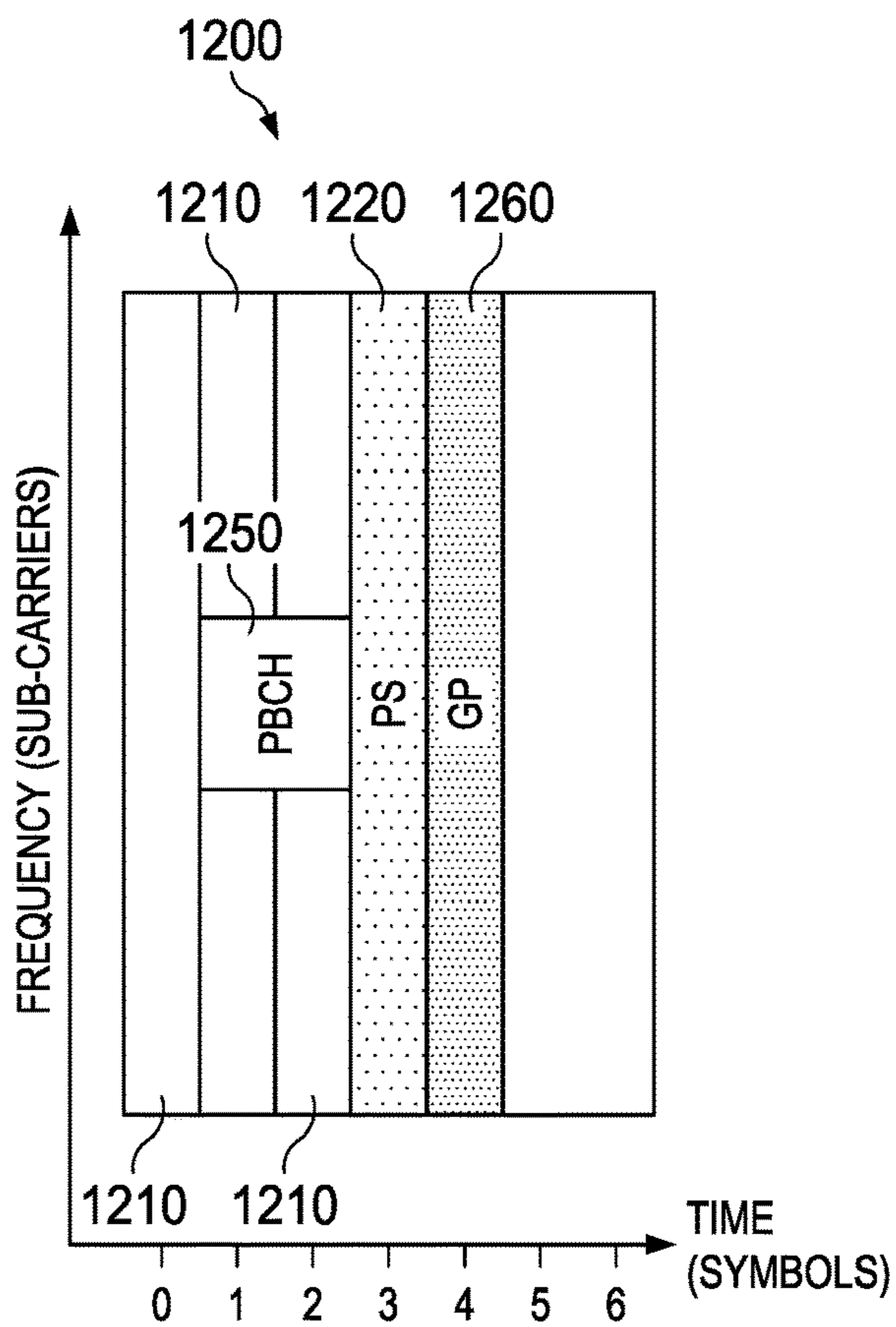
FIG. 12
