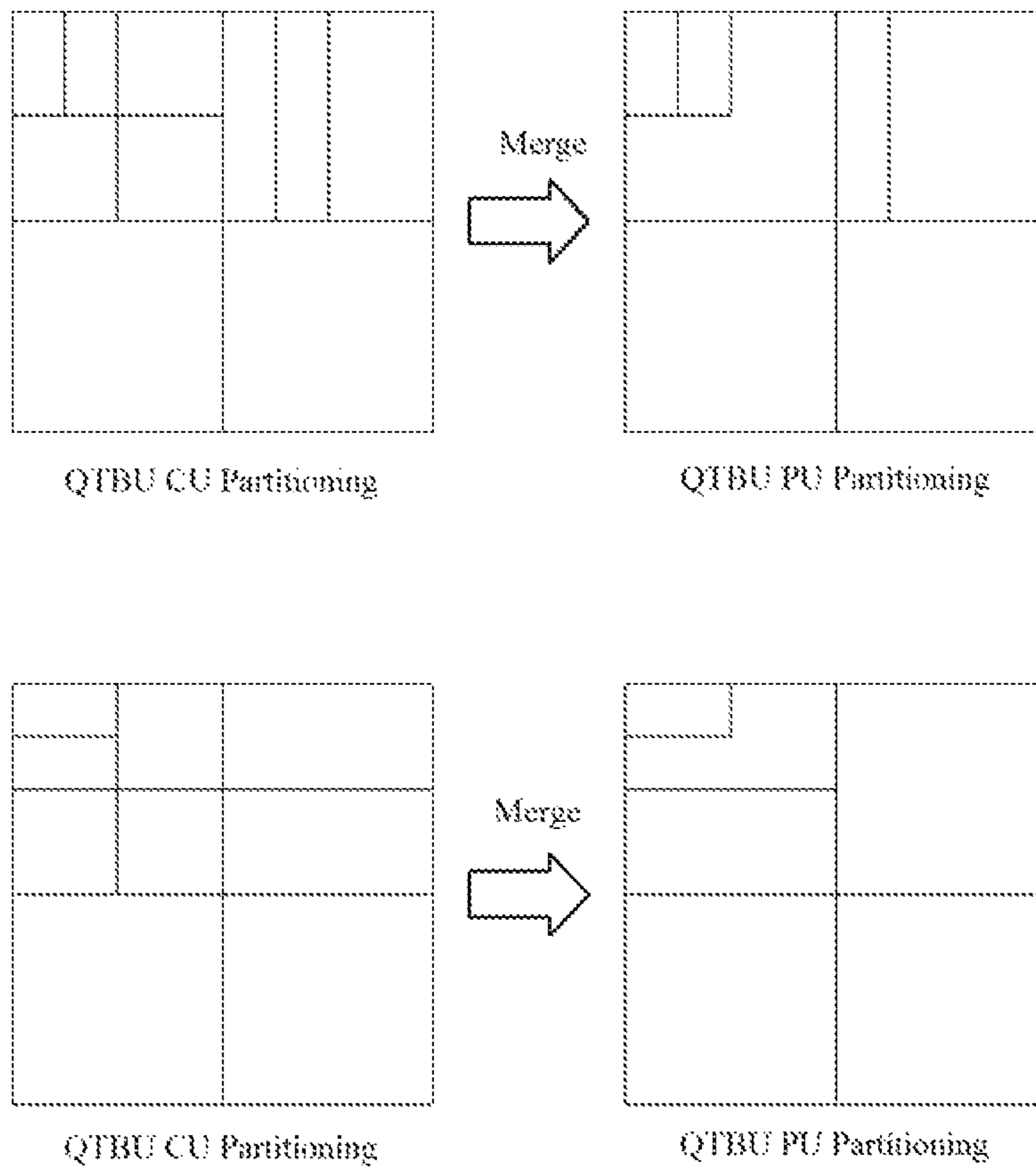
FIG. 13
