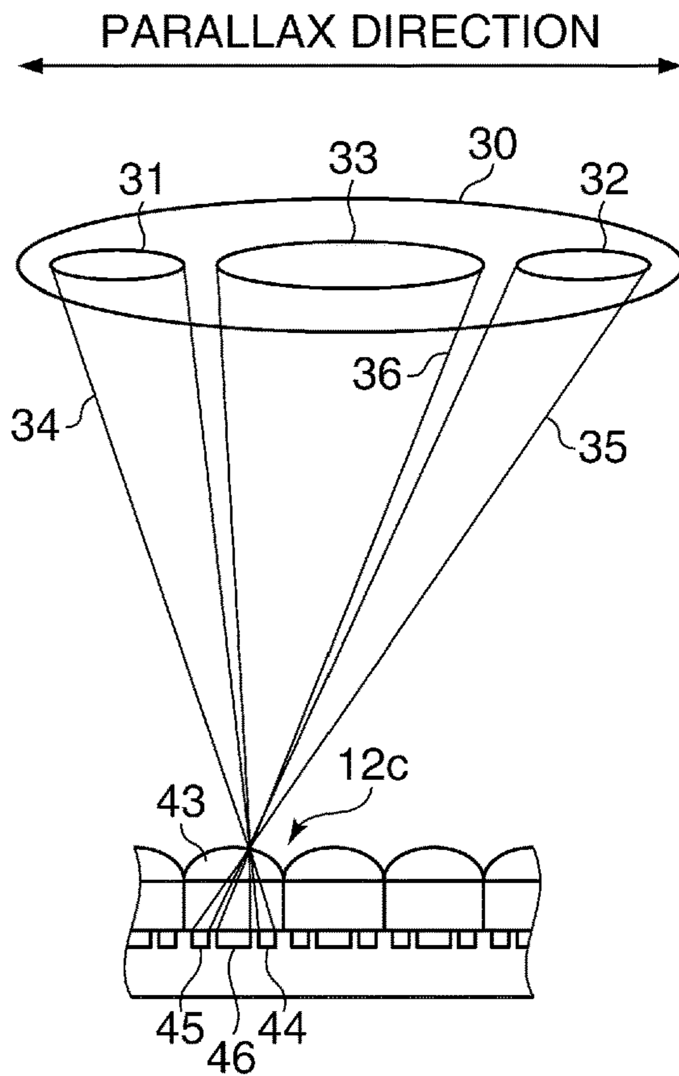
FIG. 3C
