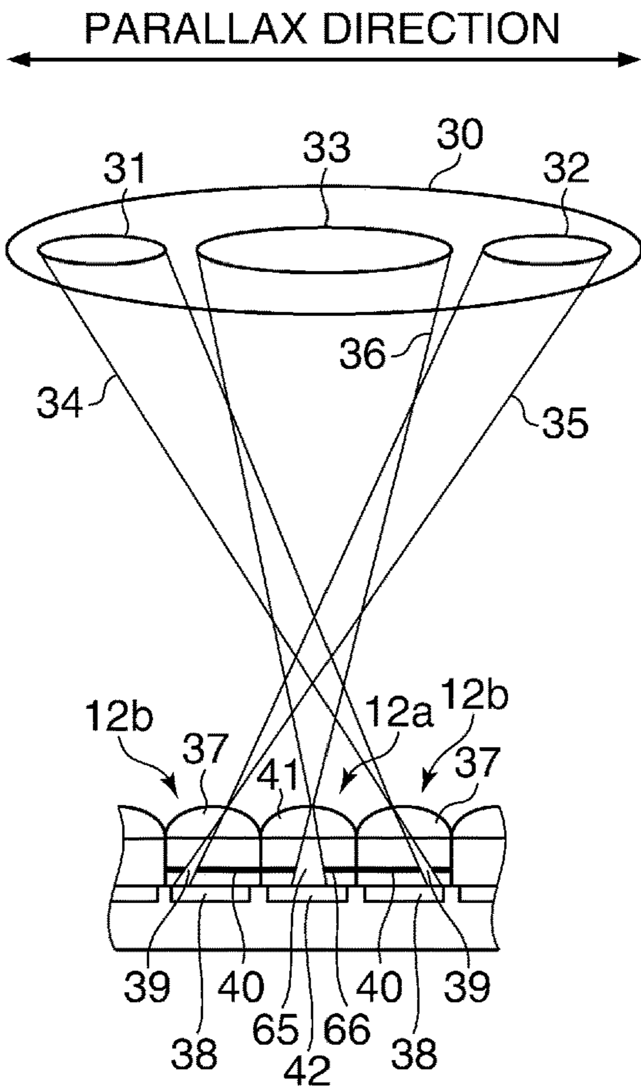
FIG. 3A
