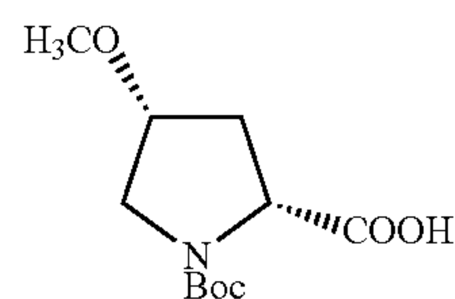
36a (+)-isomer
