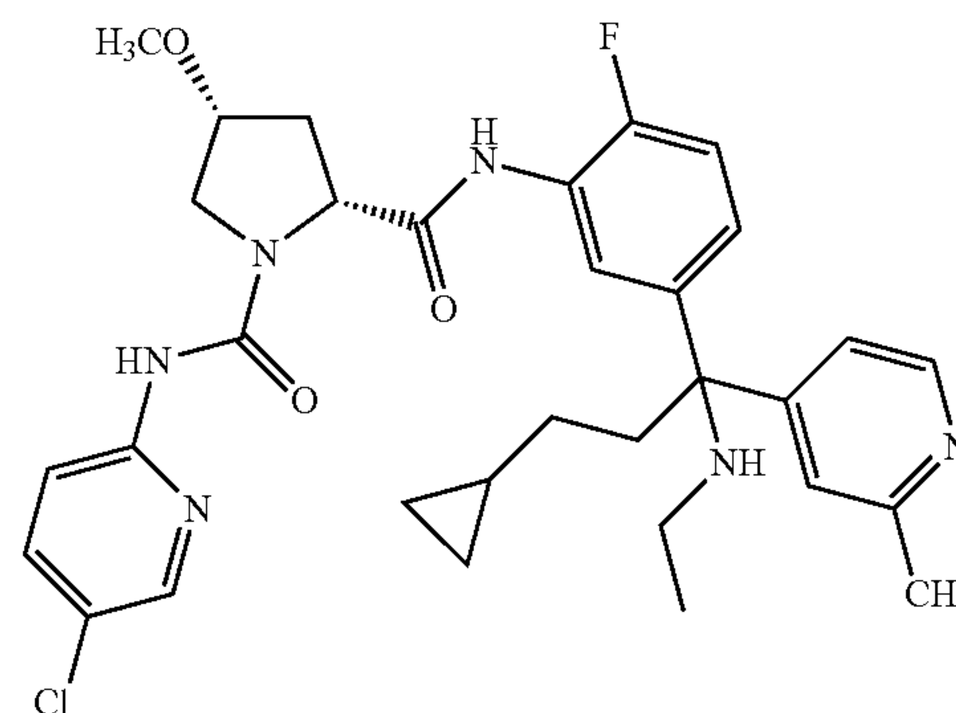
78a (+)-isomer
