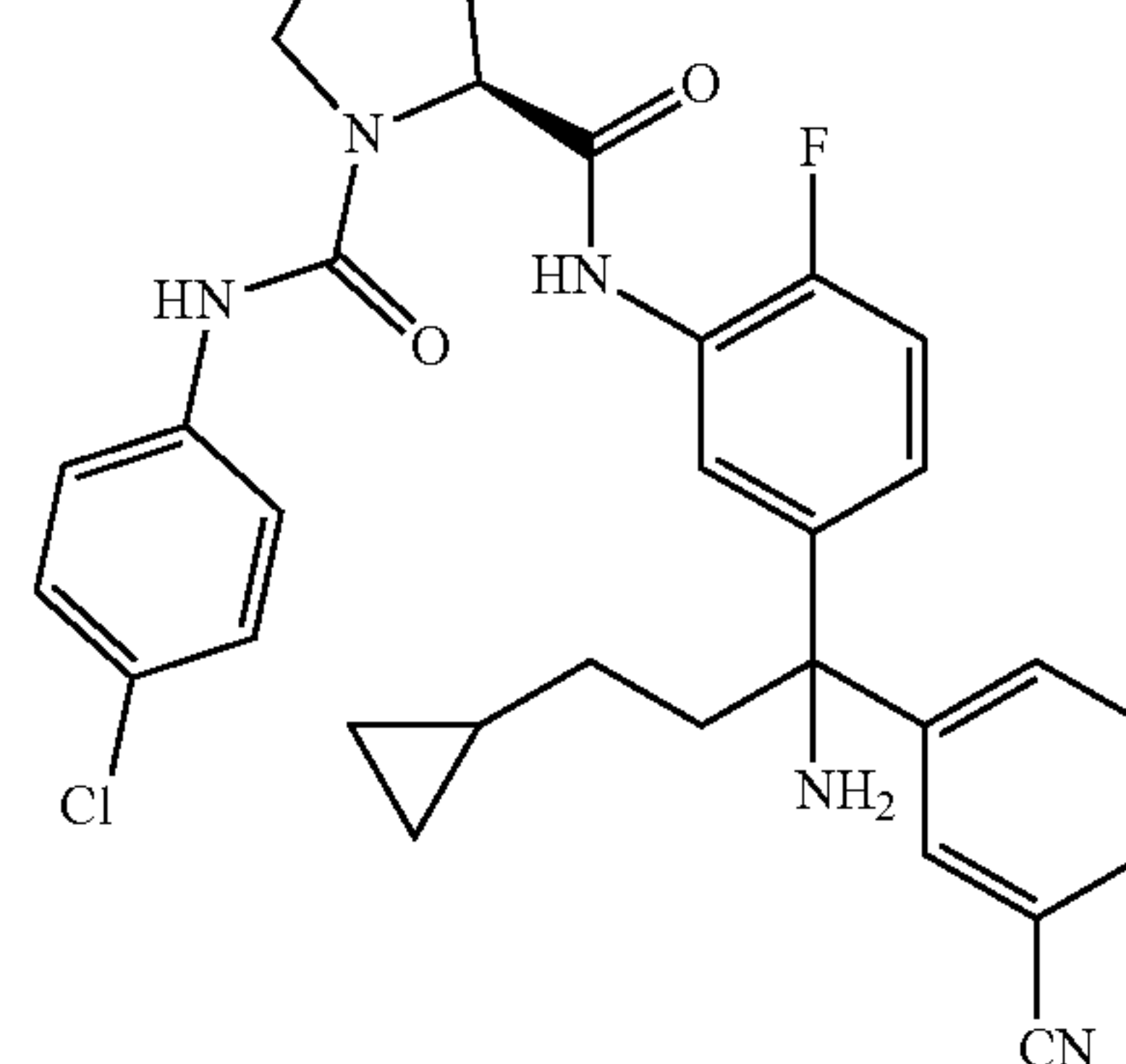
11e (-)-isomer
