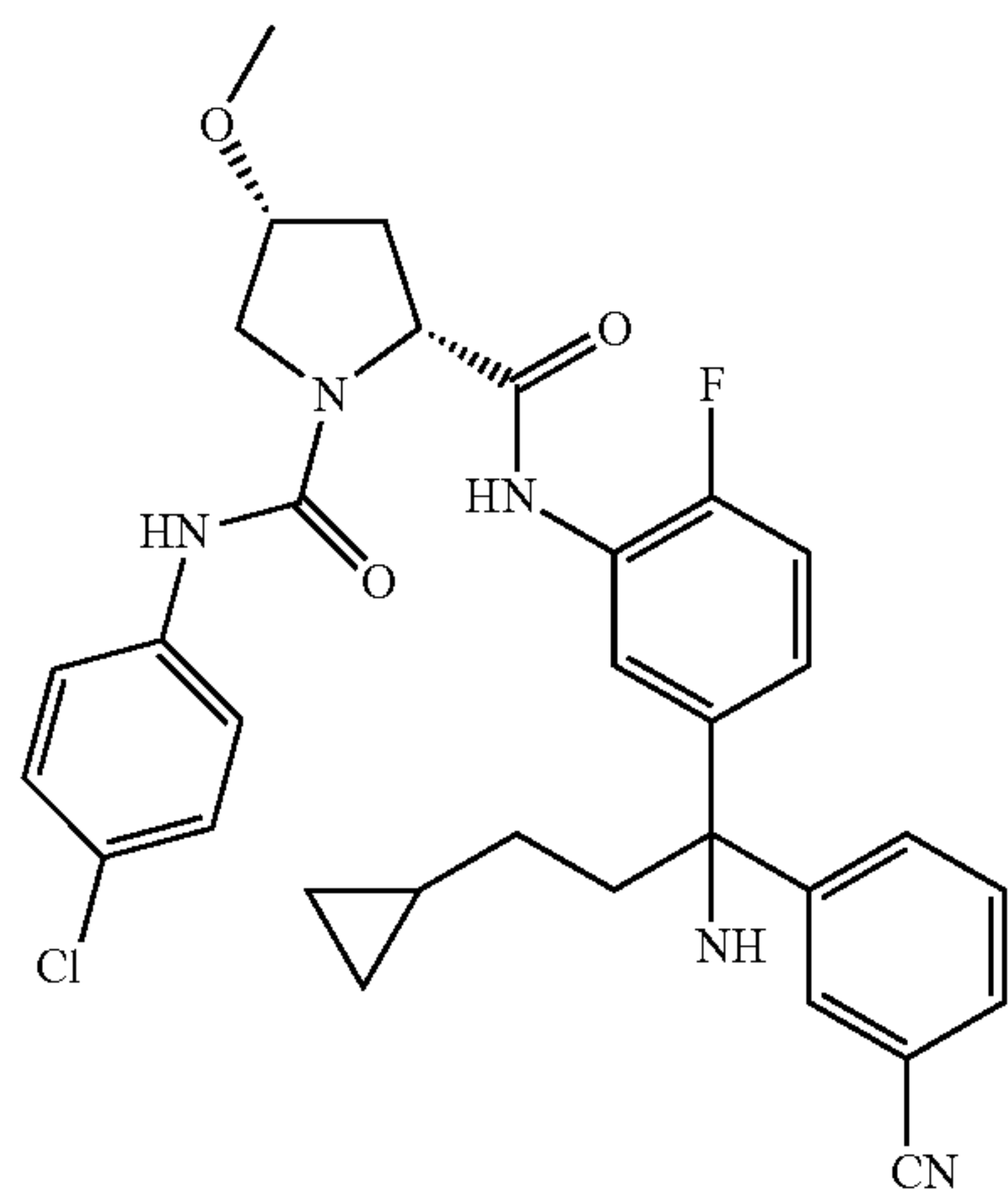
17b (+)-isomer
