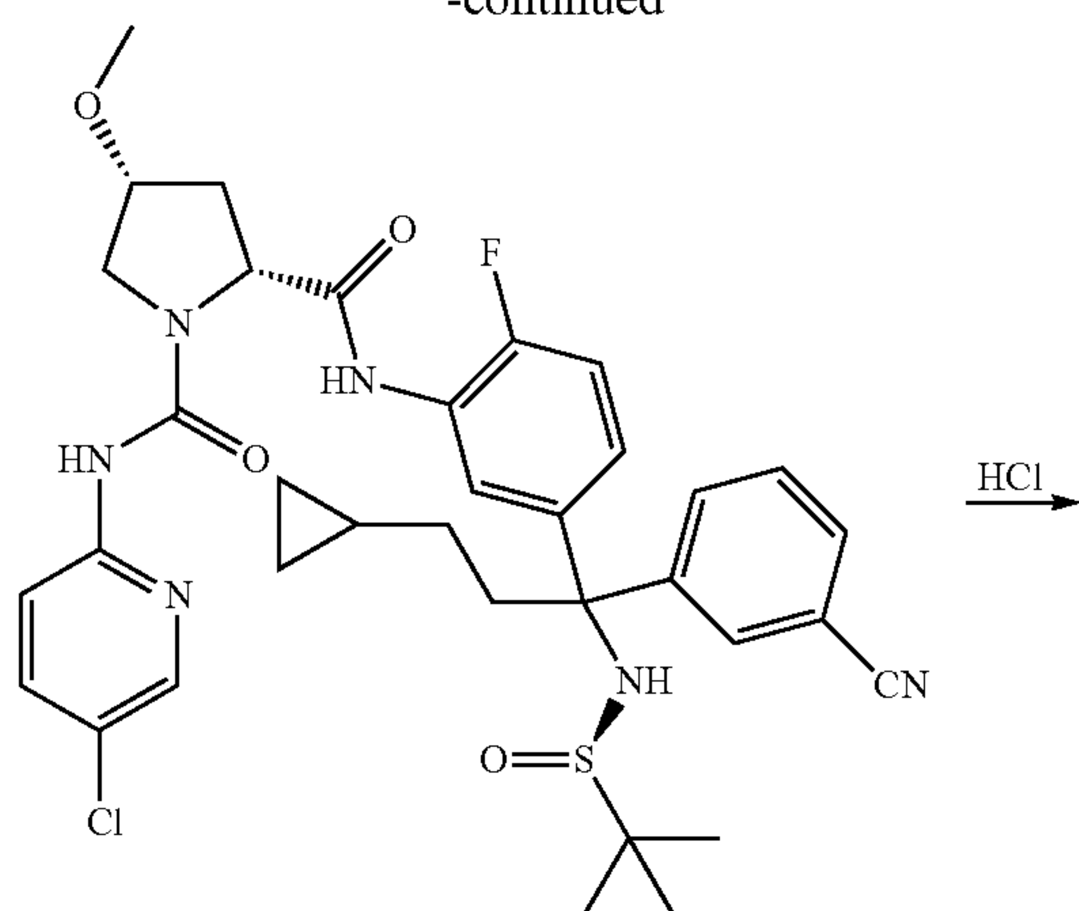
18a (-)-isomer
