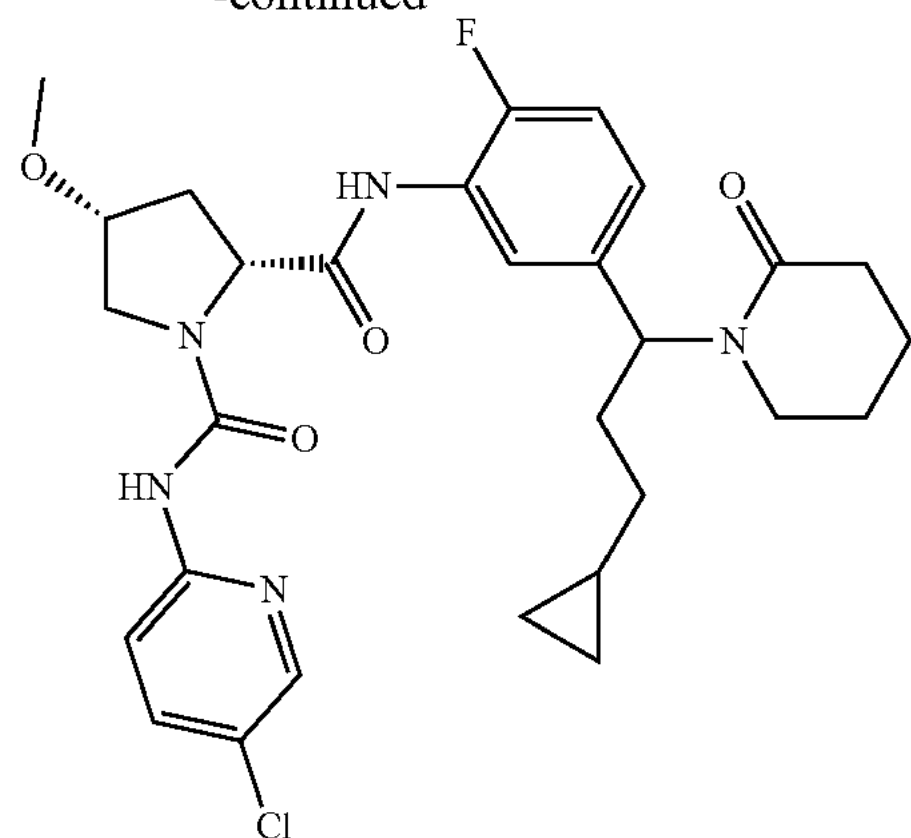
44e (+)-isomer
