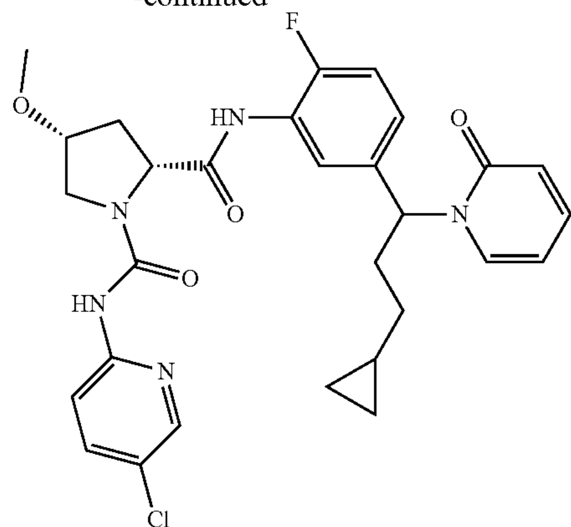
43m (+)-isomer
