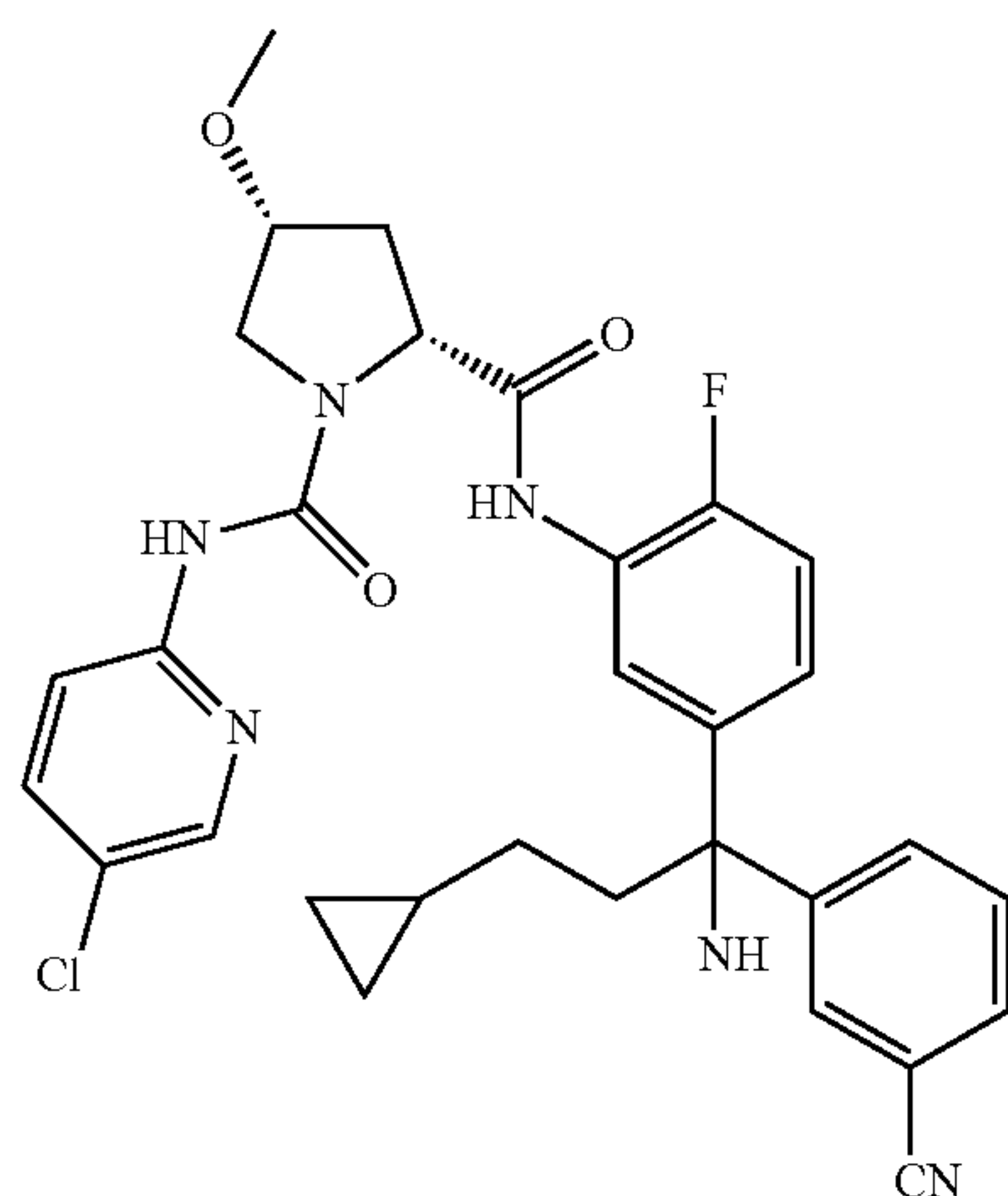
18b (+)-isomer
