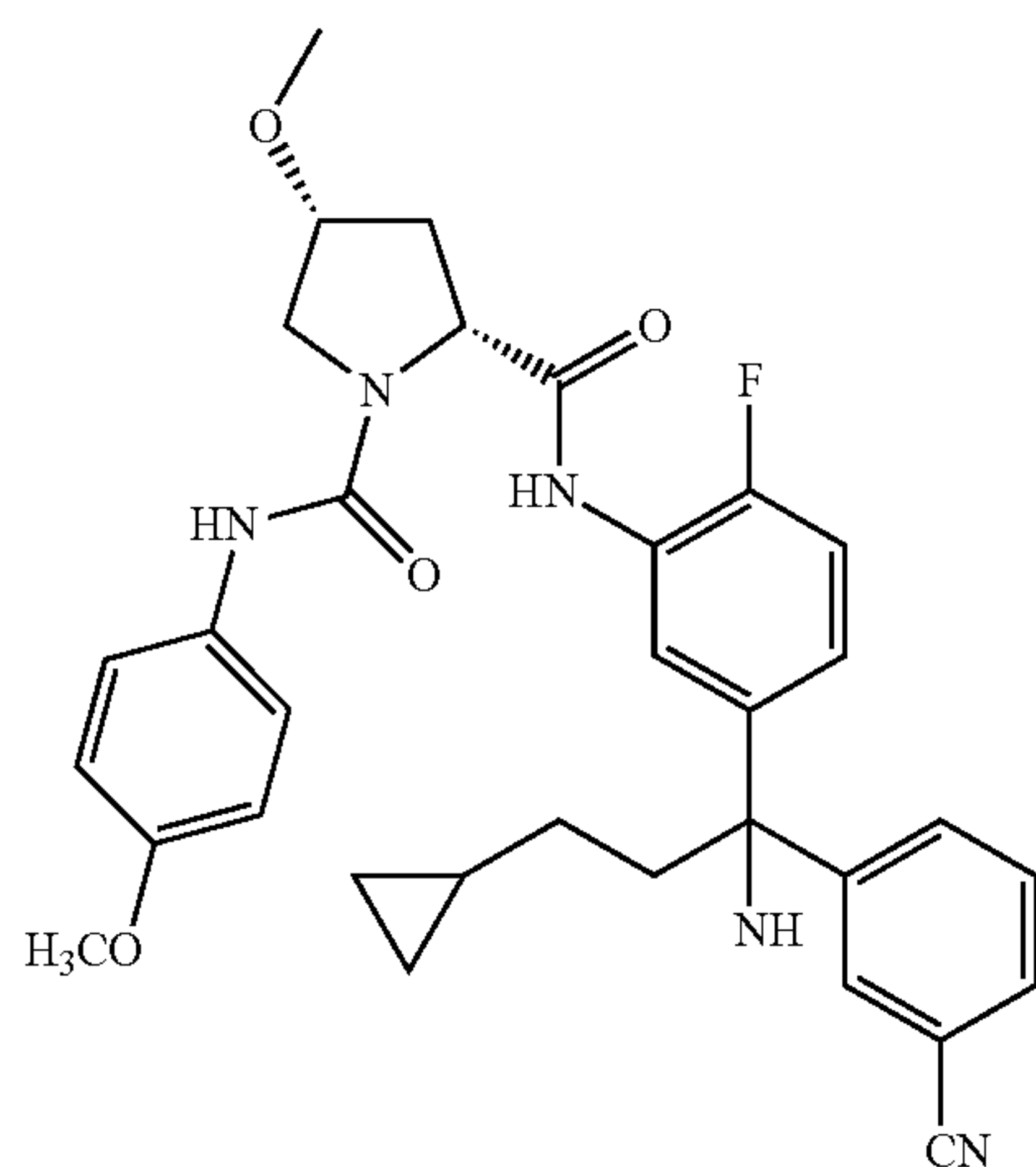
16b (+)-isomer
