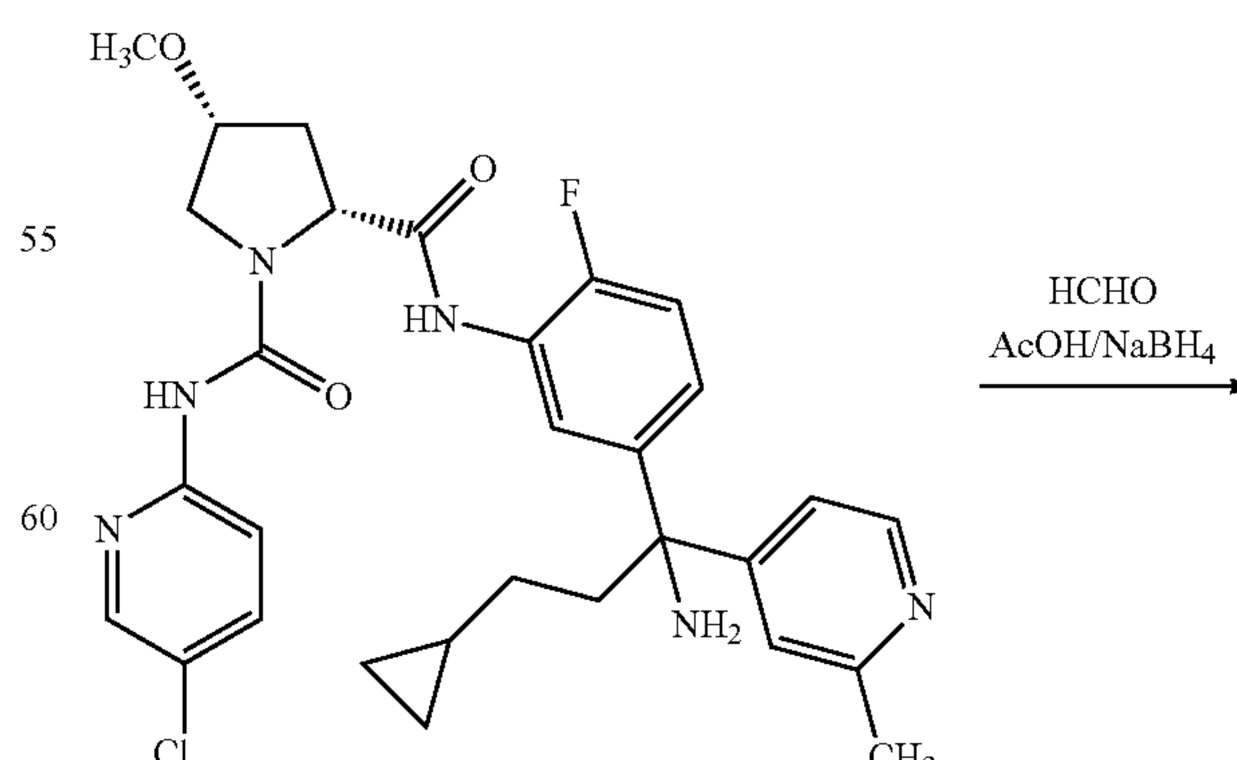
46k (+)-isomer
