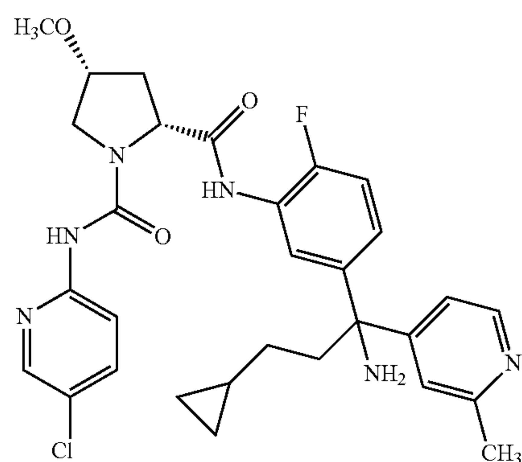
46k (+)-isomer
