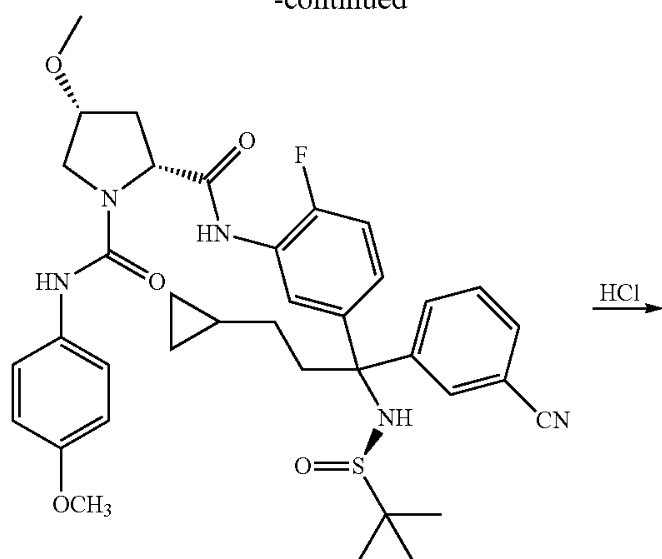
16a (-)-isomer
