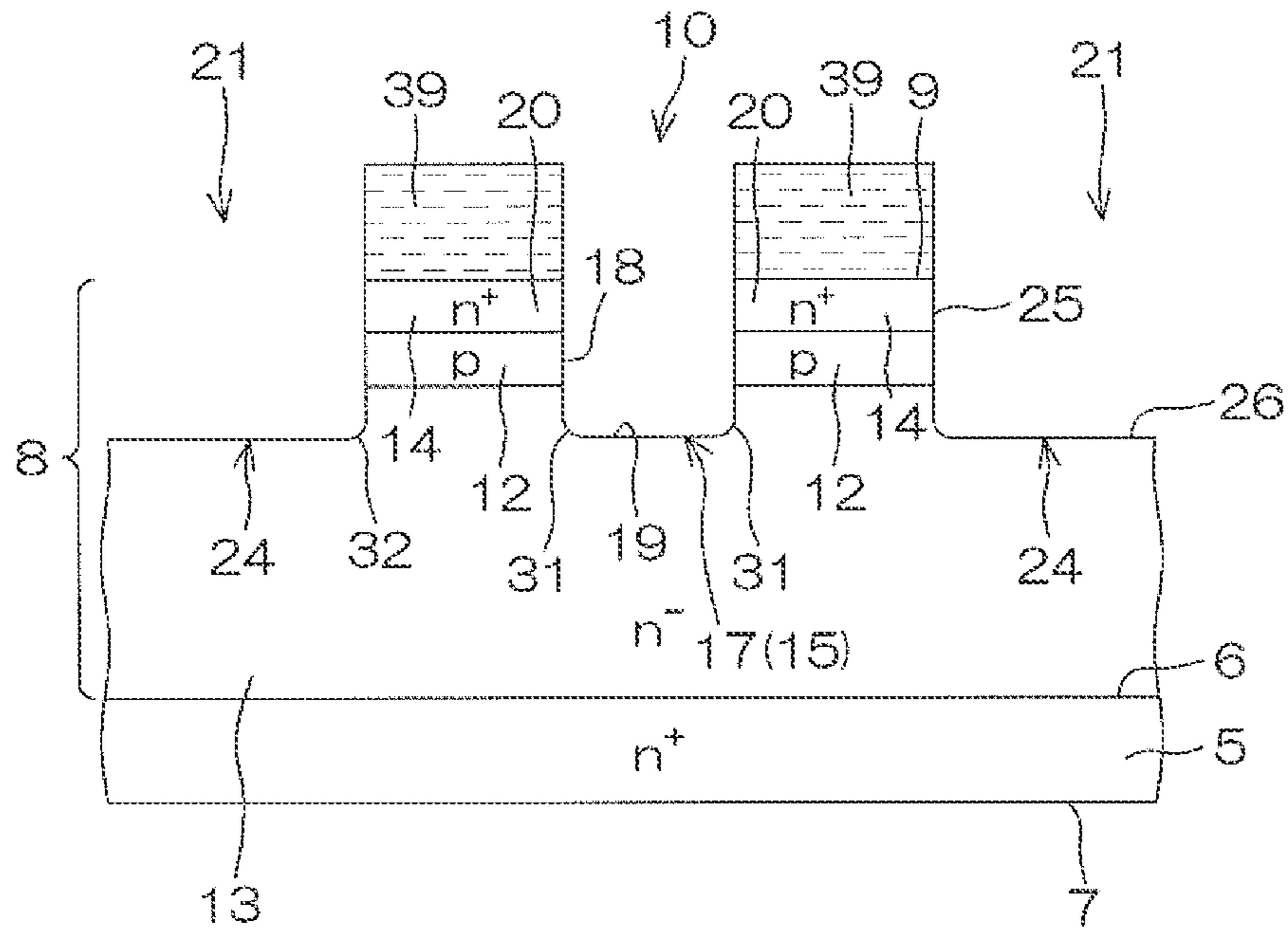
FIG. 3C A-A SECTION
