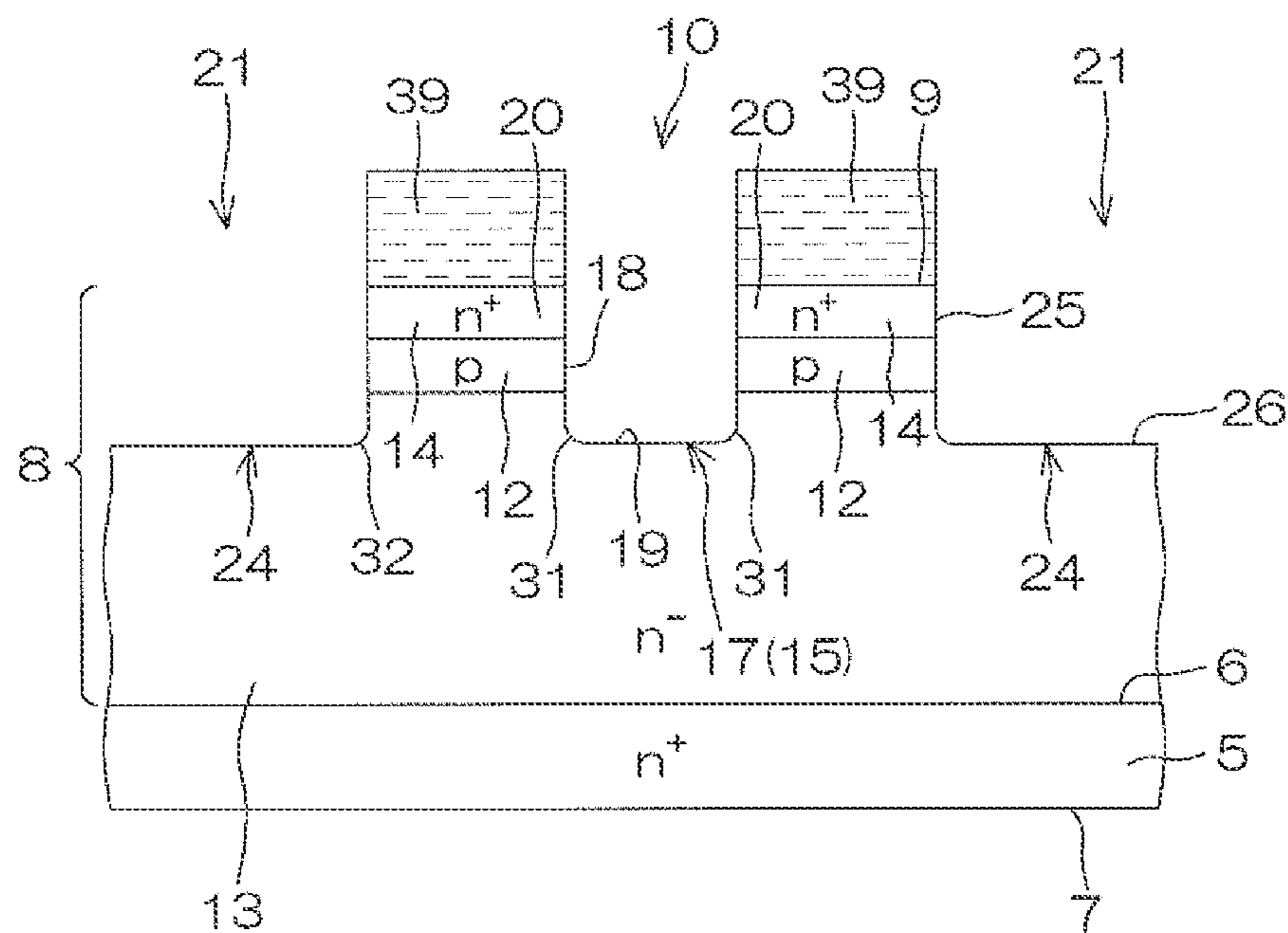
FIG. 3C A-A SECTION
