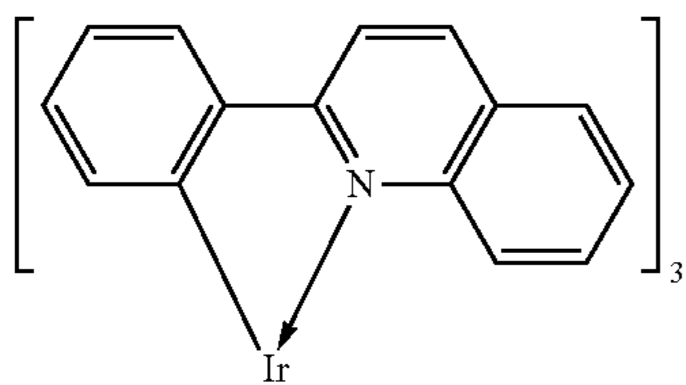
Ir(pq) 3
