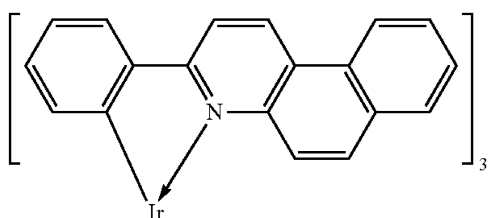
Ir(pq) 3
