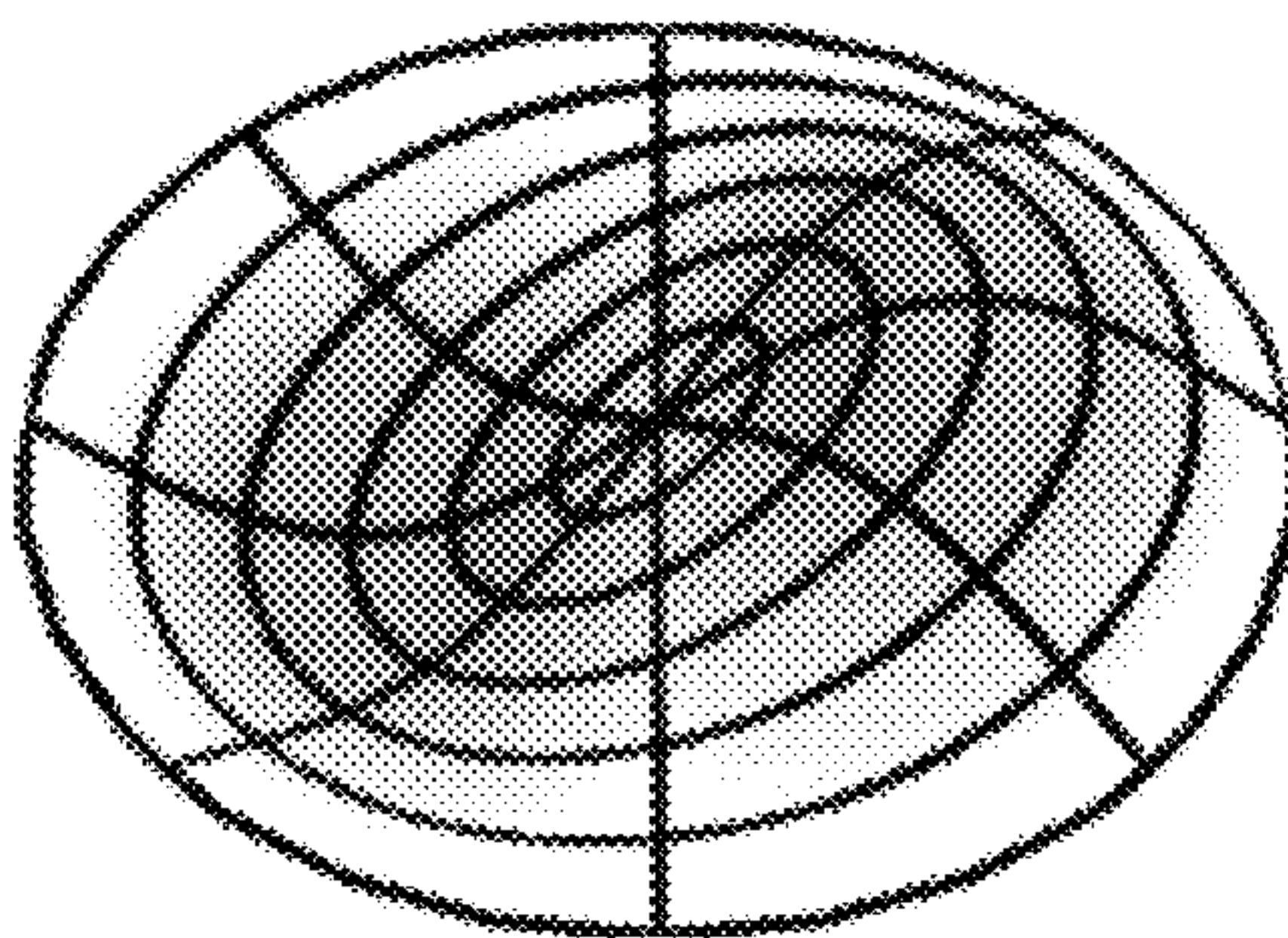
mode (1,1)
