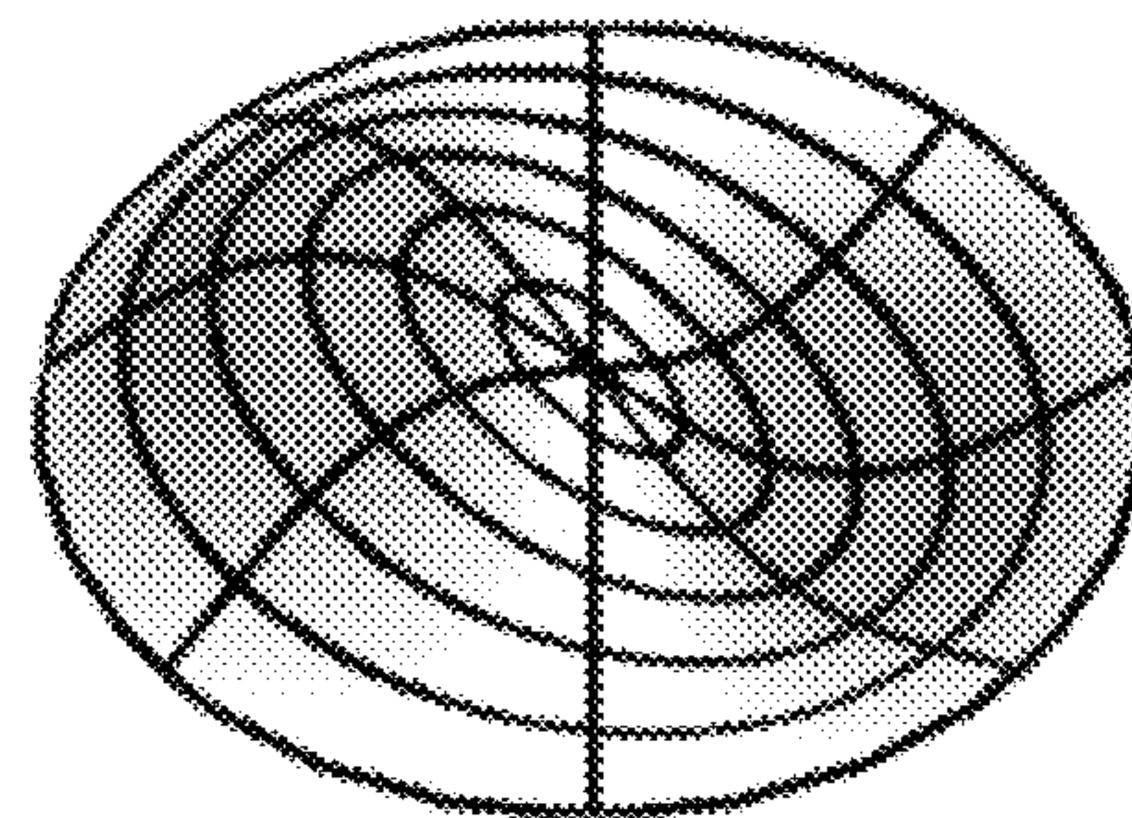
mode (1,1)
