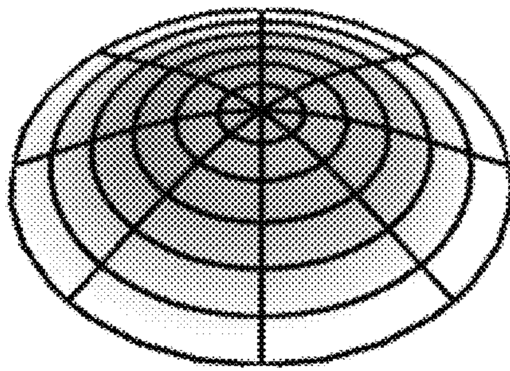
mode (0,1)
