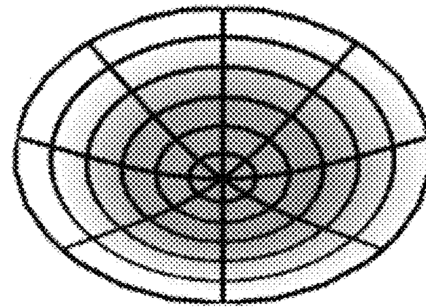
mode (0,1)
