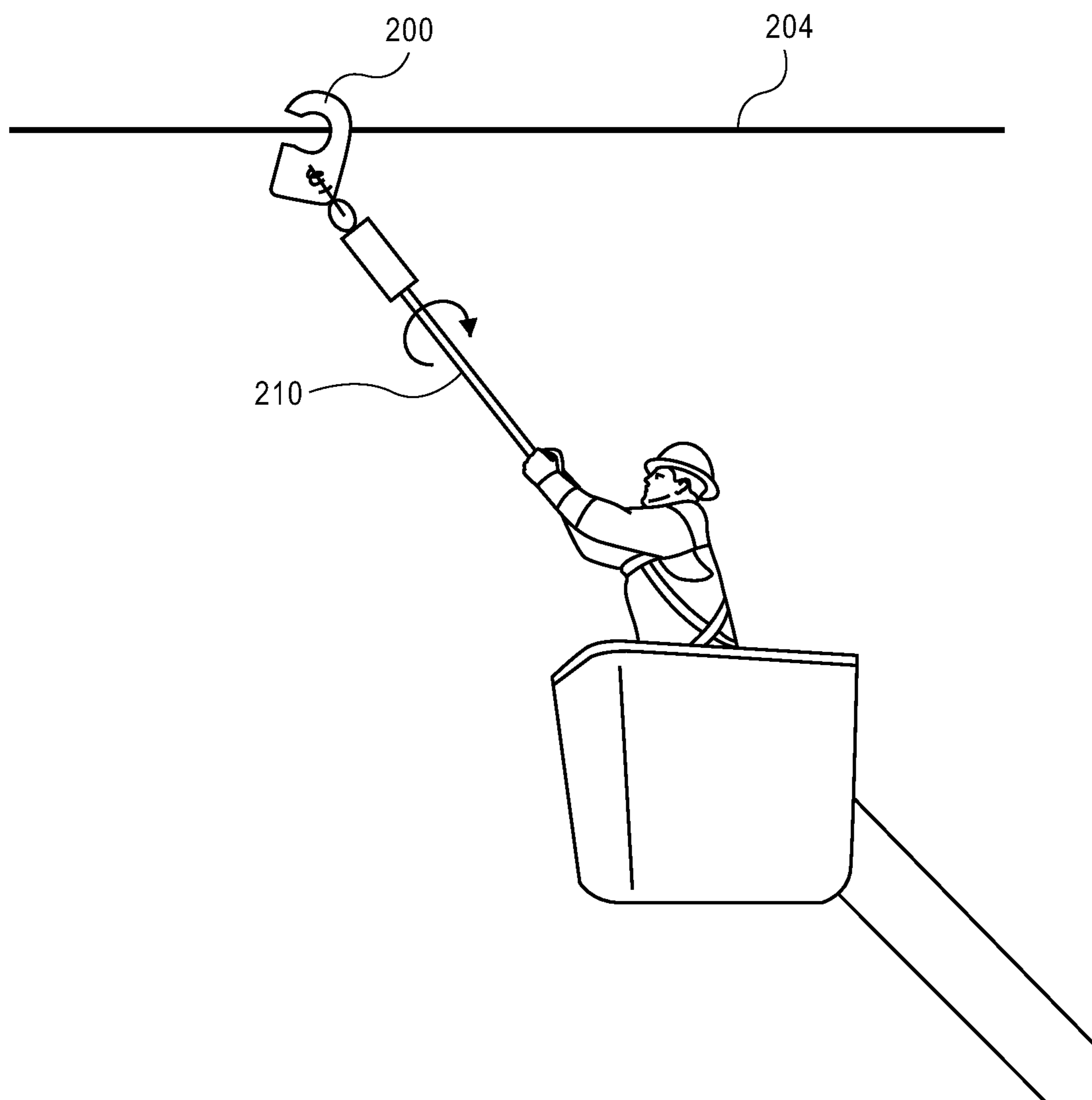
FIG. 2
